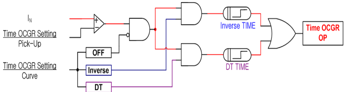
【그림 3.2】 Time OCGR(TOCGR) Logic Diagram
