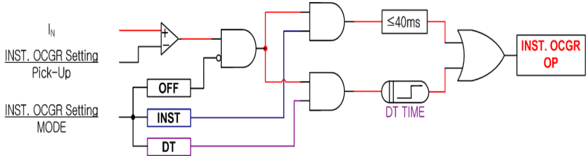
【그림 3.1】 INST.OCGR(IOCGR) Logic Diagram
