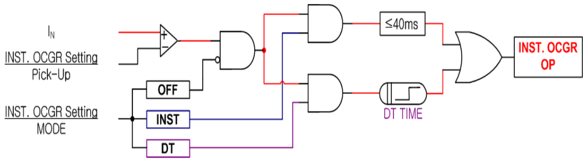
【그림 3.1】 INST.OCGR(IOCGR) Logic Diagram
