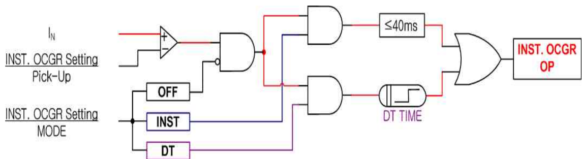
【Figure 3.10】 INST.OCGR(IOCGR) Logic Diagram
