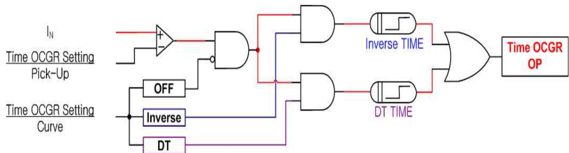
【Figure 3.11】 Time OCGR(TOCGR) Logic Diagram
