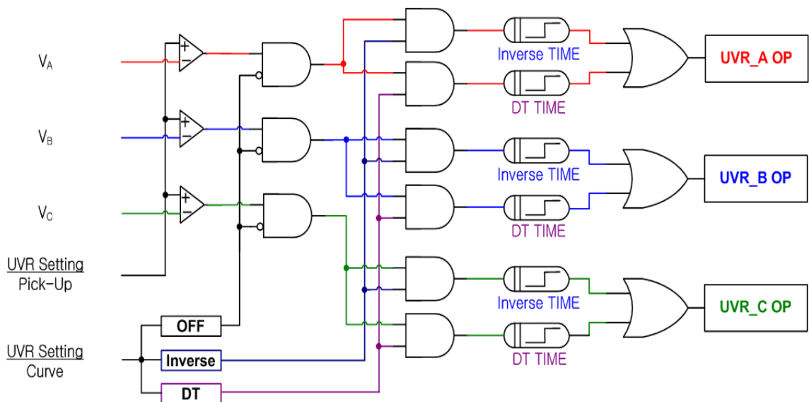
【그림 3.2】 UVR Logic Diagram
