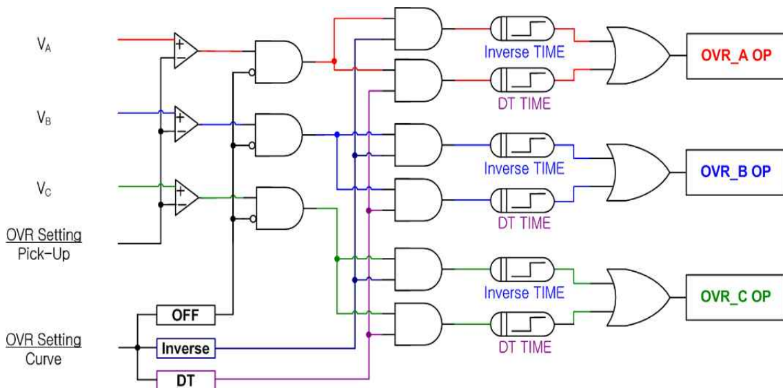
【그림 3.1】 OVR Logic Diagram
