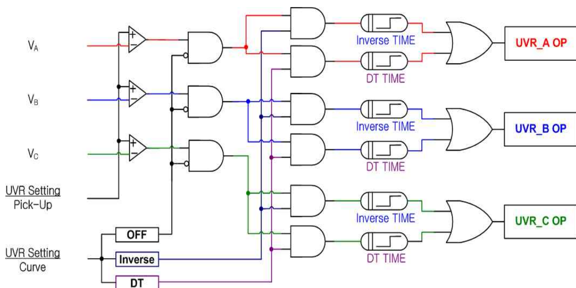
【Figure 3.2】 UVR Logic Diagram
