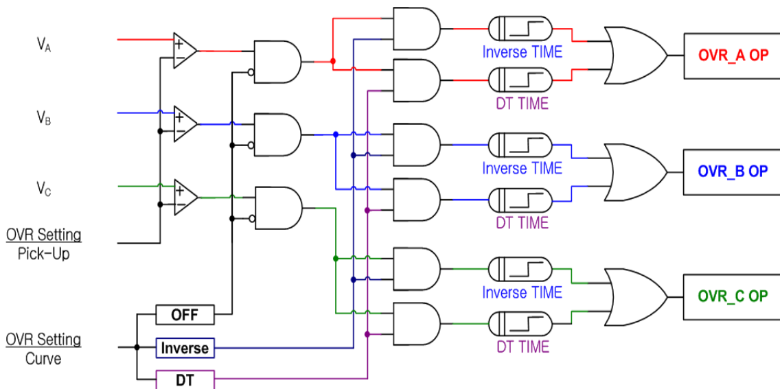
【그림 3.1】 OVR Logic Diagram
