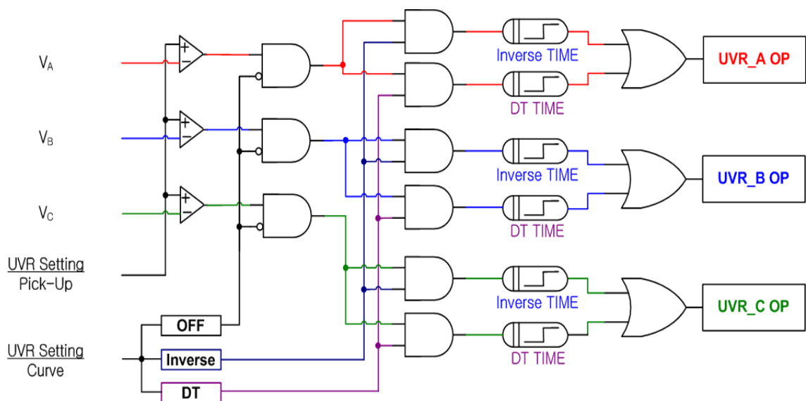
【그림 3.2】 UVR Logic Diagram
