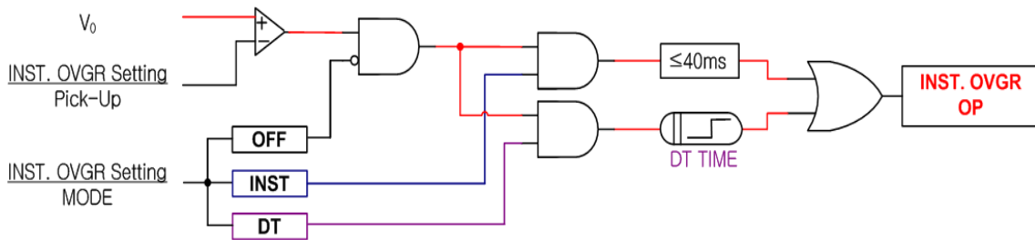
【그림 3.3】 INST. OVGR(IOVGR) Logic Diagram
