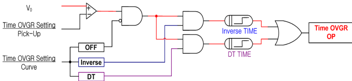
【그림 3.4】 TIME OVGR(TOVGR) Logic Diagram
