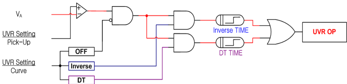
【그림 3.1】 UVR Logic Diagram
