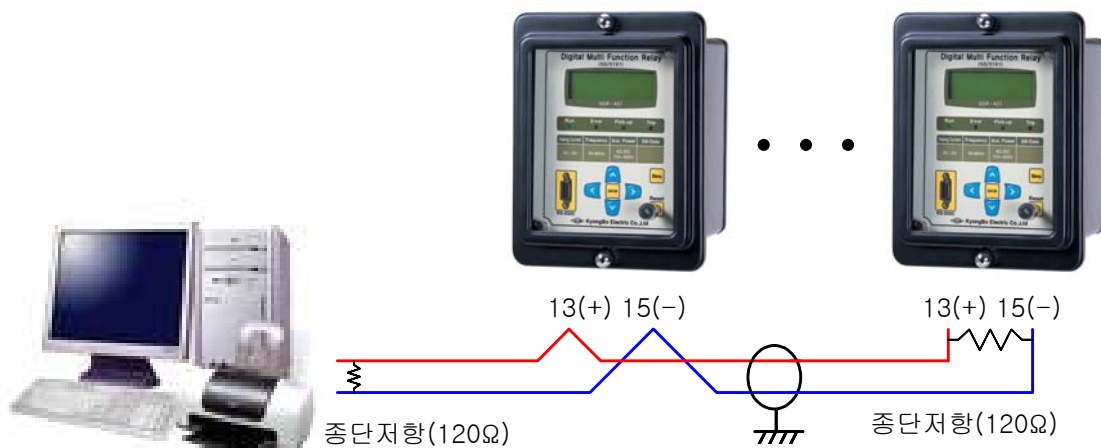
【그림 4.3】 RS-485C 결선도
