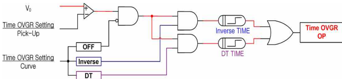
【그림 3.2】 TIME OVGR(TOVGR) Logic Diagram
