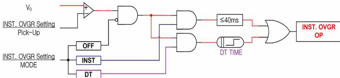
【그림 3.1】 INST. OVGR(IOVGR) Logic Diagram
