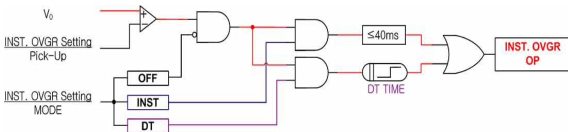
【그림 3.1】 INST. OVGR(IOVGR) Logic Diagram
