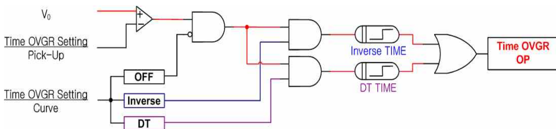
【그림 3.2】 TIME OVGR(TOVGR) Logic Diagram
