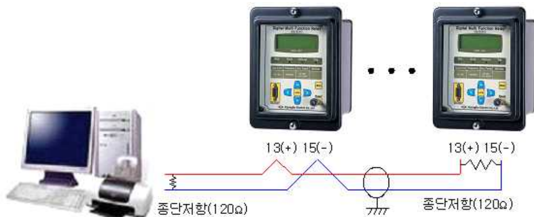
【그림 4.3】 RS-485C 결선도
