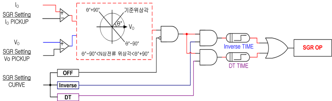
【그림 3.1】 SGR Logic Diagram
