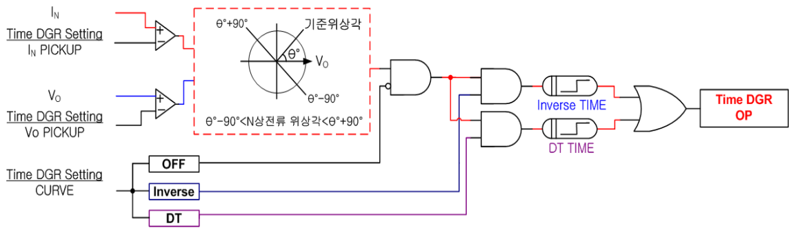
【그림 3.1】 Time DGR Logic Diagram
