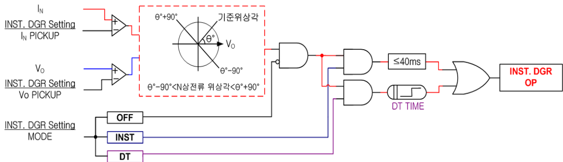
【그림 3.2】 INST. DGR Logic Diagram
