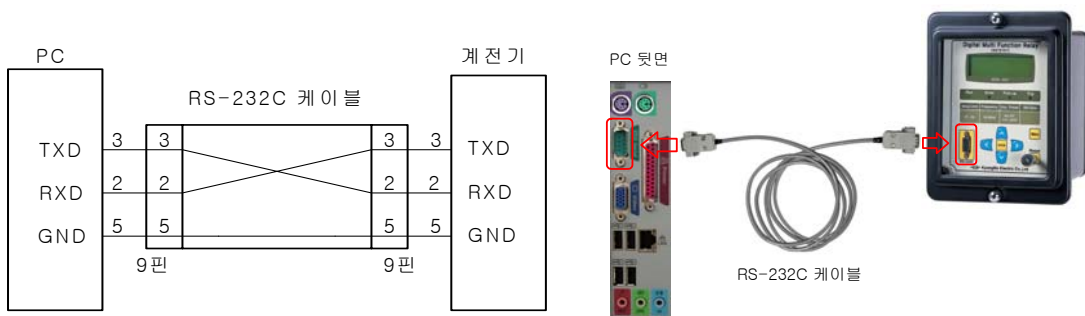
【그림 4.1】 RS-232C 회로도
