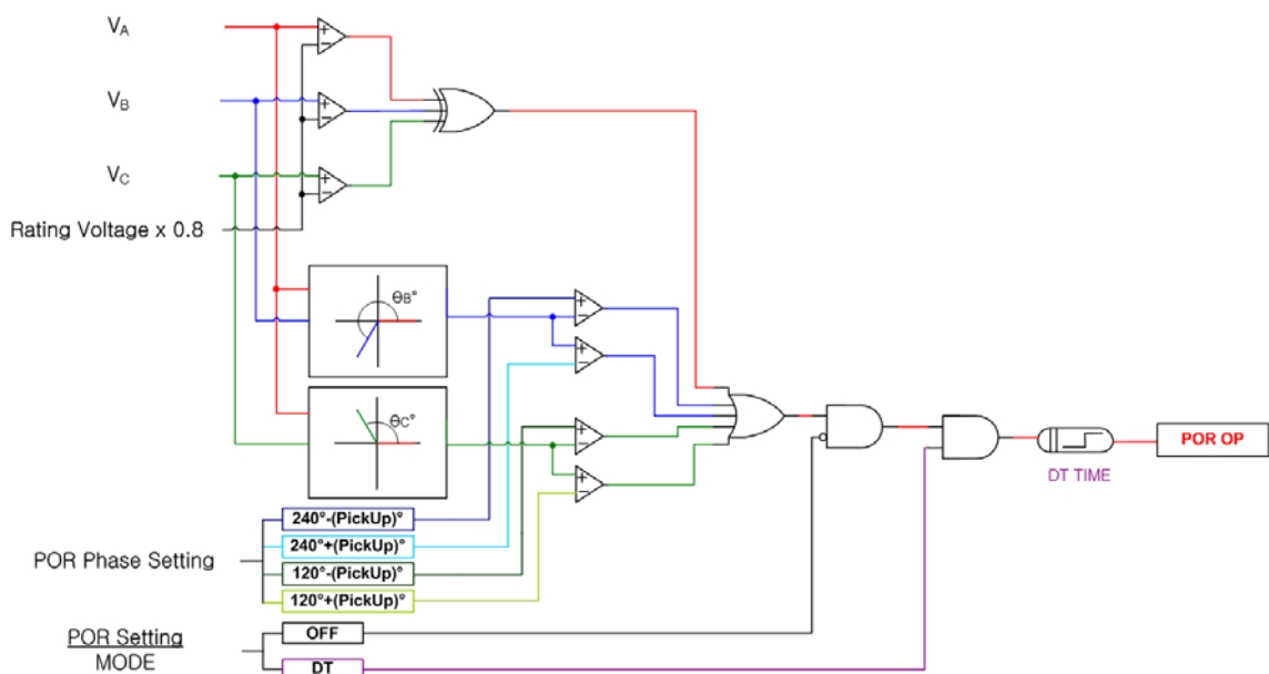
【그림 3.1】 POR Logic Diagram
