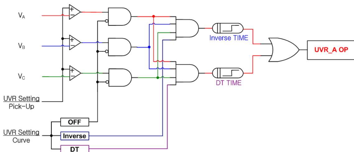
【그림 3.3】 UVR Logic Diagram
