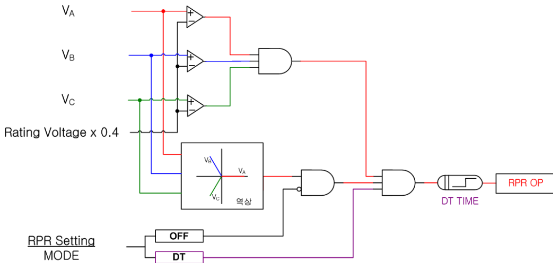
【그림 3.2】 RPR Logic Diagram
