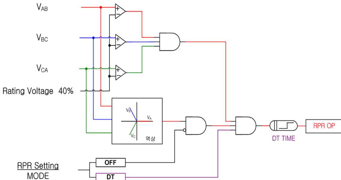
【그림 3.9】 RPR Logic Diagram
