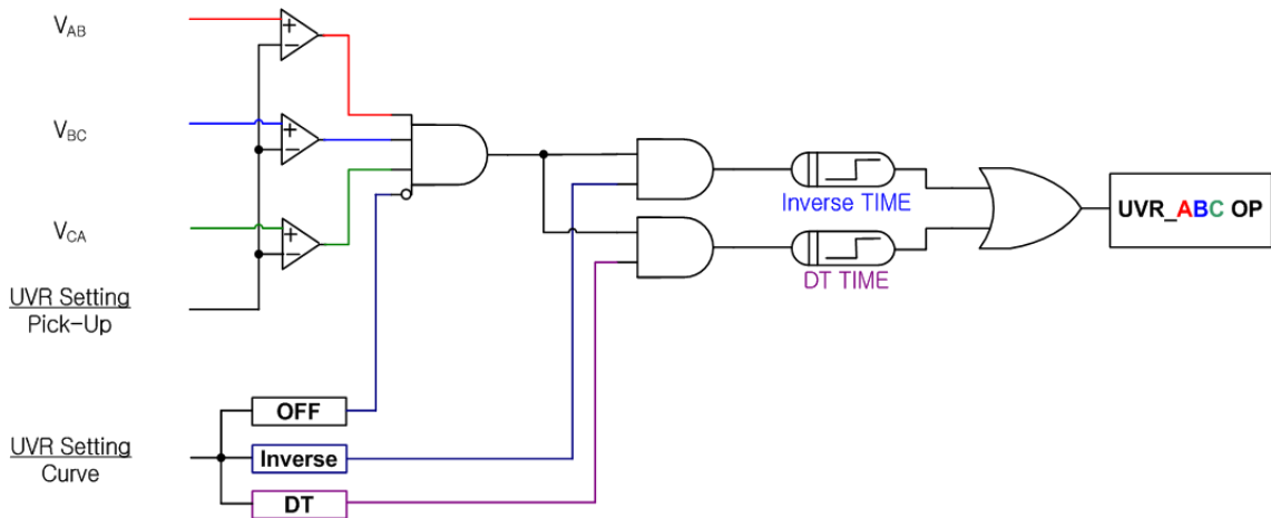
【그림 3.7】 UVR Logic Diagram ( 3 Phases )
