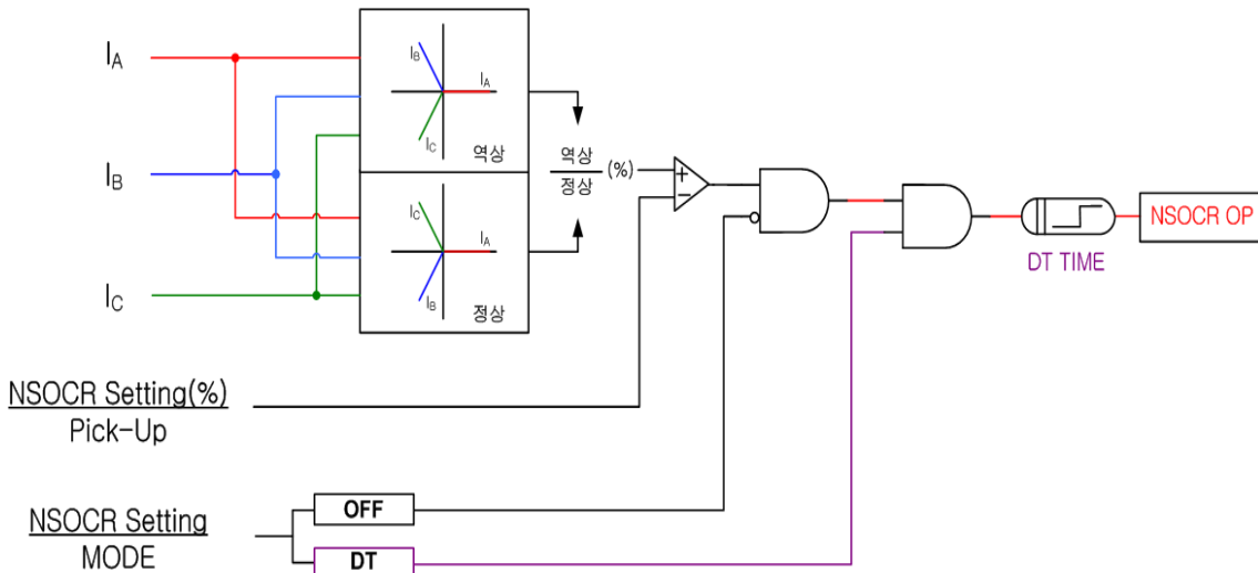
【그림 3.8】 NSOCR Logic Diagram
