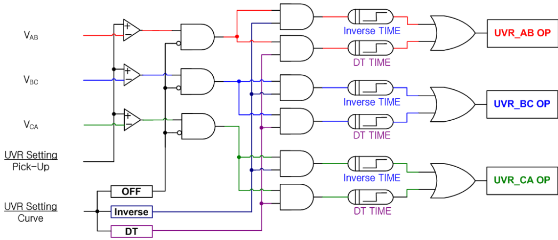
【그림 3.6】 UVR Logic Diagram ( 1 Phase )
