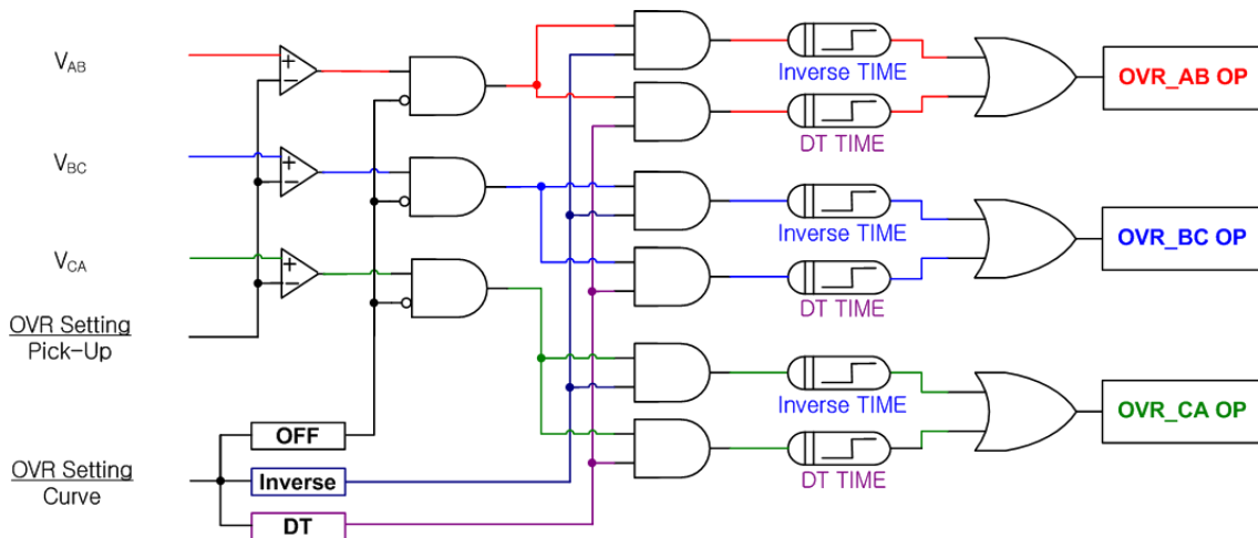
【그림 3.4】 OVR Logic Diagram ( 1 Phase )
