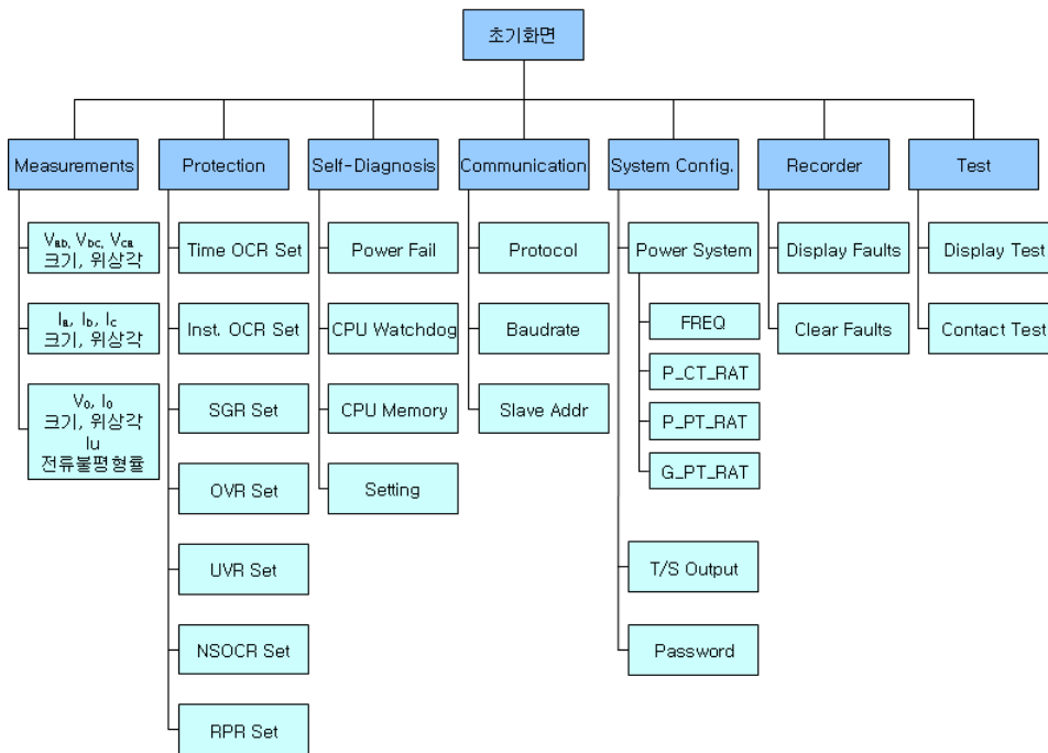
【그림 6.1】 Menu Tree
