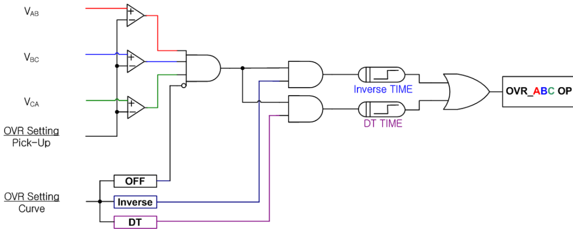
【그림 3.5】 OVR Logic Diagram ( 3 Phases )
