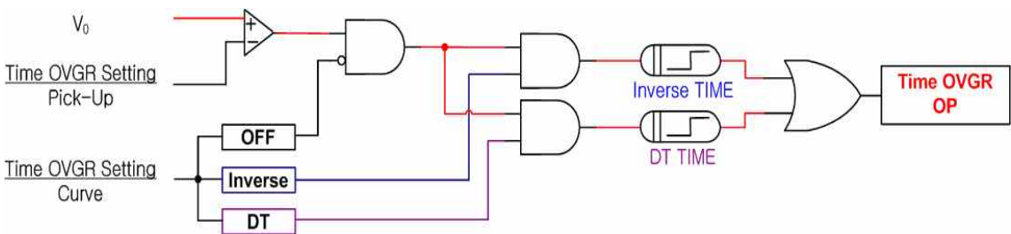
【그림 3.12】 TIME OVGR(TOVGR) Logic Diagram
