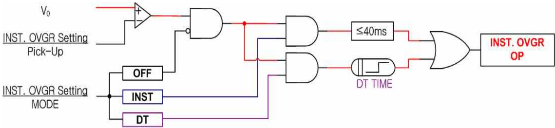
【그림 3.11】 INST OVGR(IOVGR) Logic Diagram
