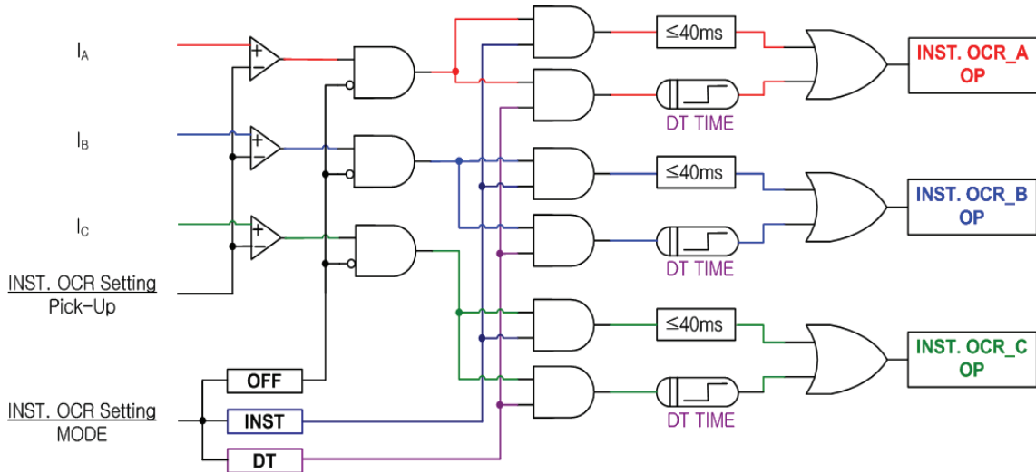
【그림 3.1】 INST.OCR(IOCR) Logic Diagram
