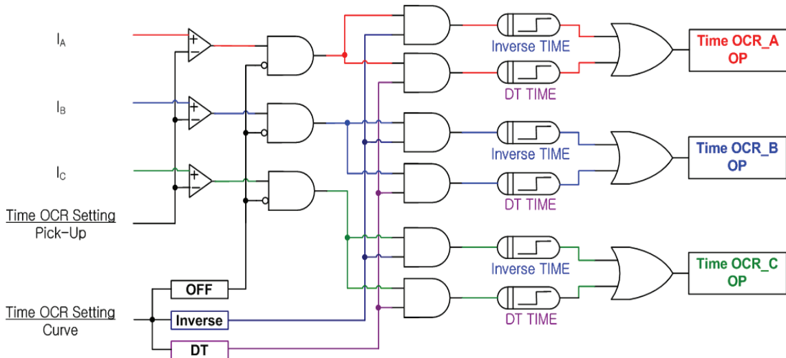
【그림 3.2】 Time OCR(TOCR) Logic Diagram
