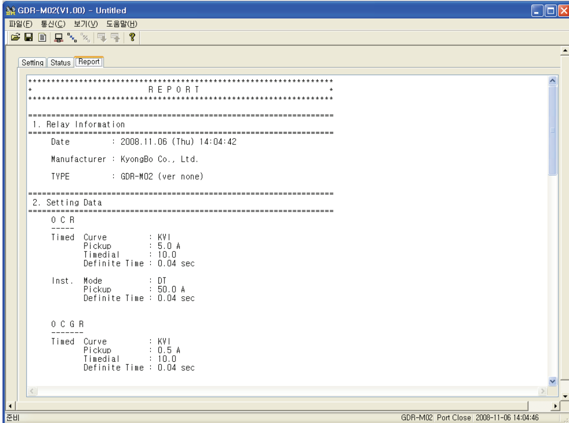
【그림 7.5】 GDR-M02 Report
