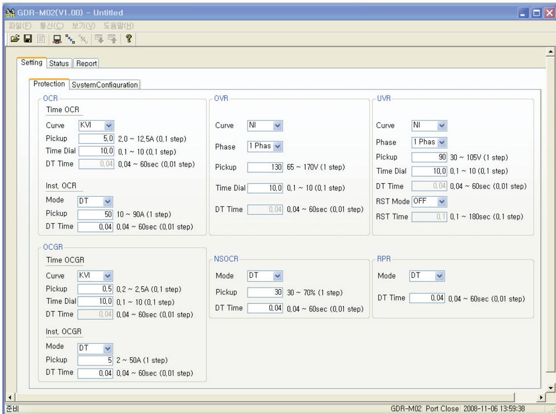
【그림 7.1】 GDR-M02 초기화면
