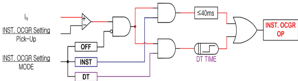
【그림 3.3】 INST.OCGR(IOCGR) Logic Diagram
