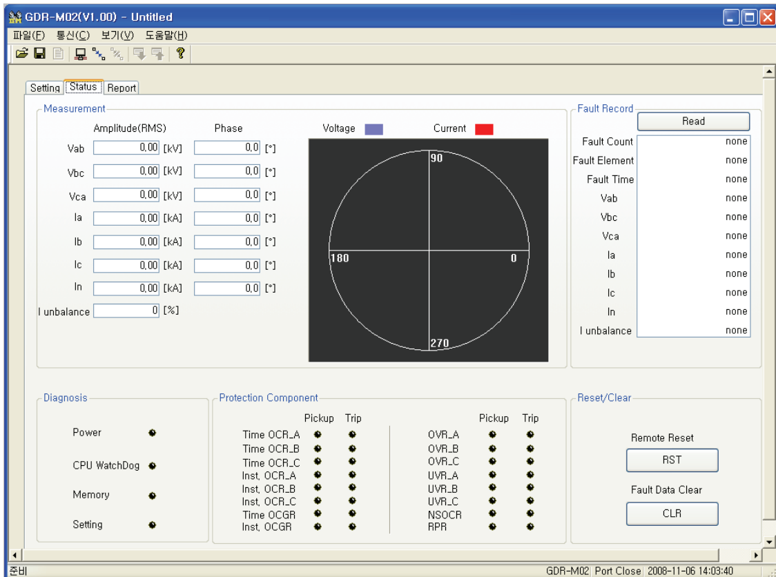
【그림 7.4】 GDR-M02 Status
