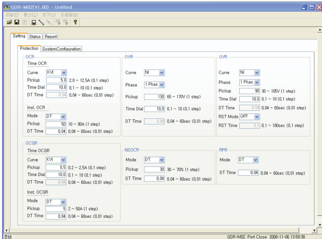
【그림 7.3】 GDR-M02 Setting
