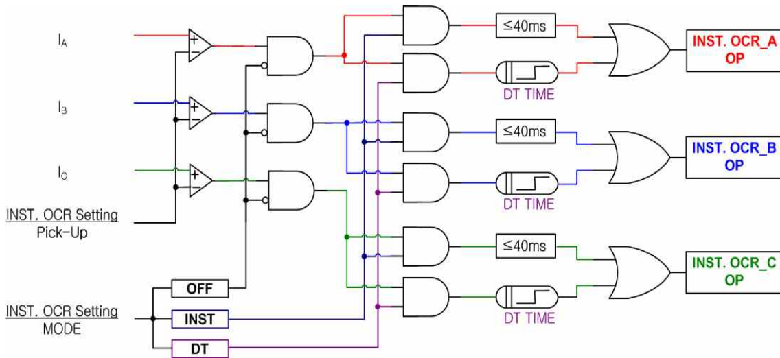
【그림 3.1】 INST.OCR(IOCR) Logic Diagram
