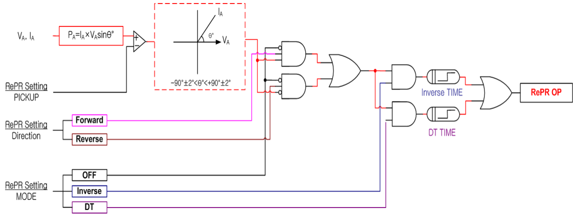
【그림 3.6】 RePR Logic Diagram
