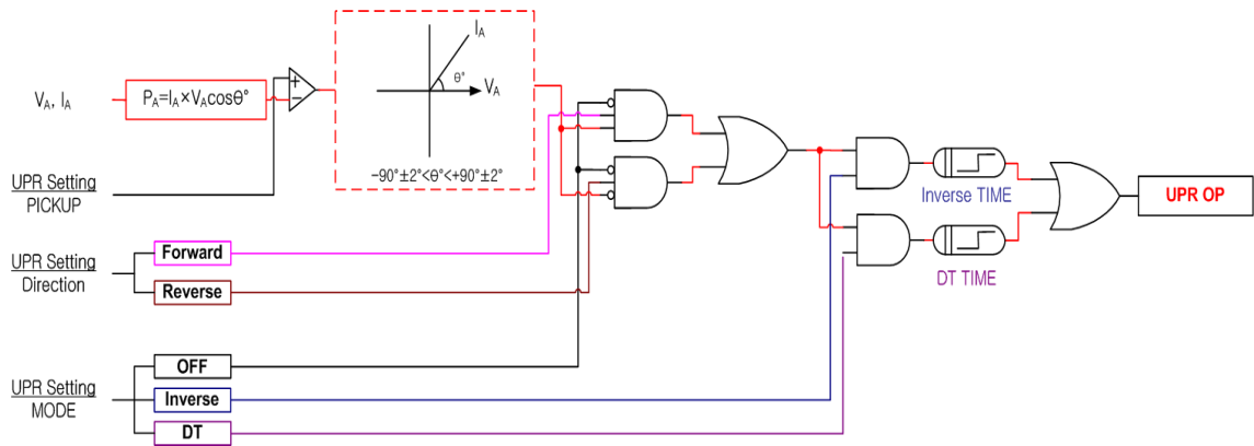
【그림 3.4】 UPR Logic Diagram
