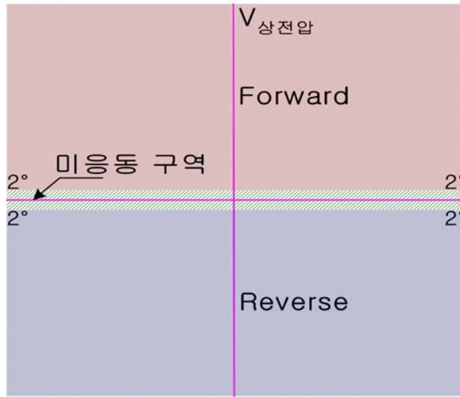
【그림 3.1】 O(R)PR 방향성 동작 특성
