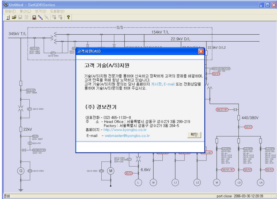
[그림 7.7] 도움말
