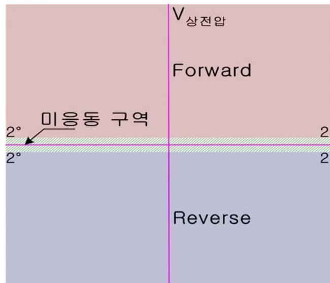
【그림 3.5】 RePR 방향성 동작 특성
