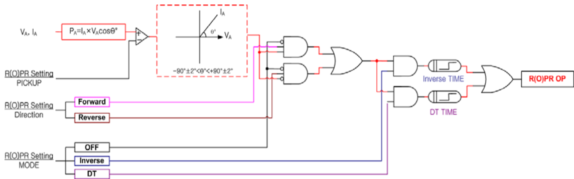
【그림 3.2】 O(R)PR Logic Diagram
