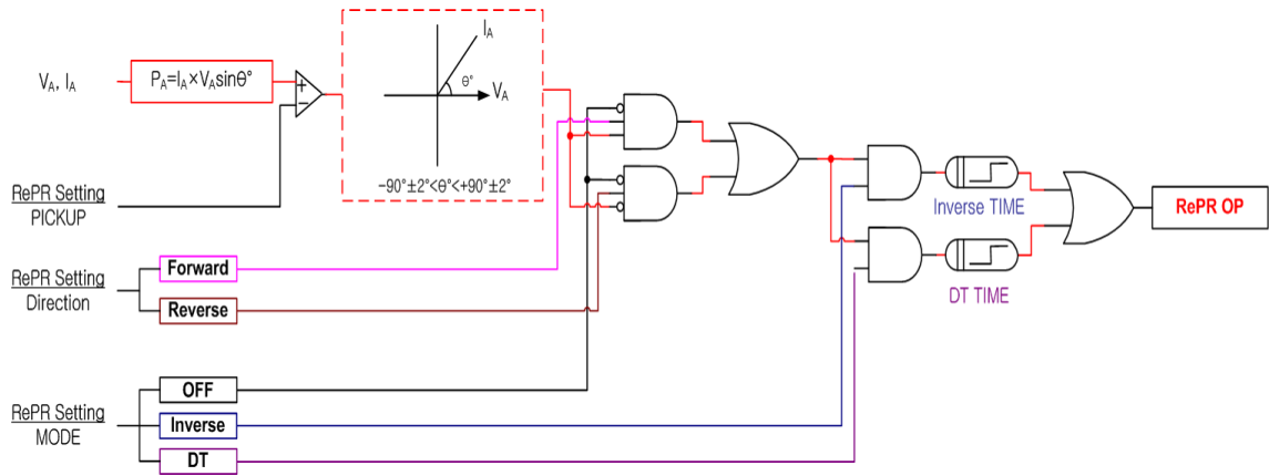
【그림 3.6】 RePR Logic Diagram
