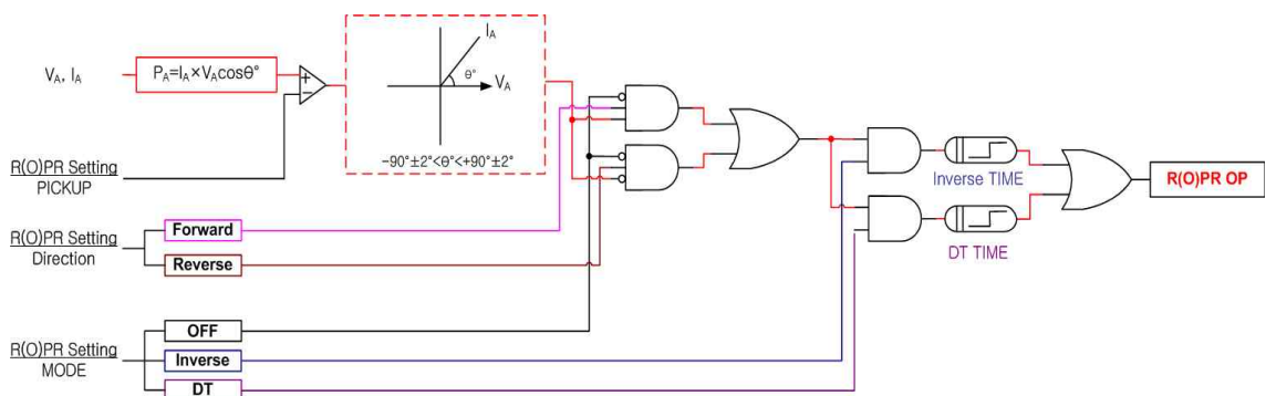
【Figure 3.2】 O(R)PR Logic Diagram
