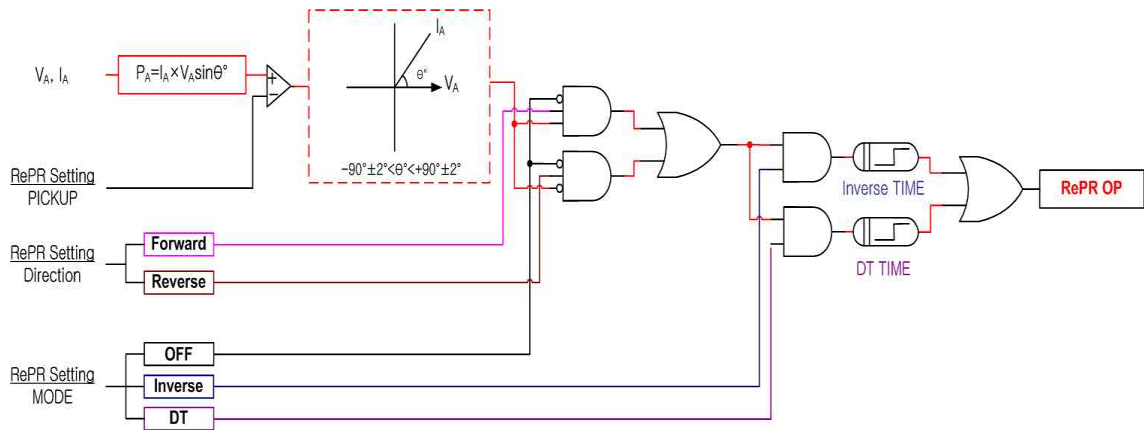
【Figure 3.6】 RePR Logic Diagram
