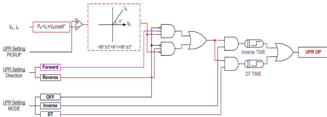
【Figure 3.4】 UPR Logic Diagram
