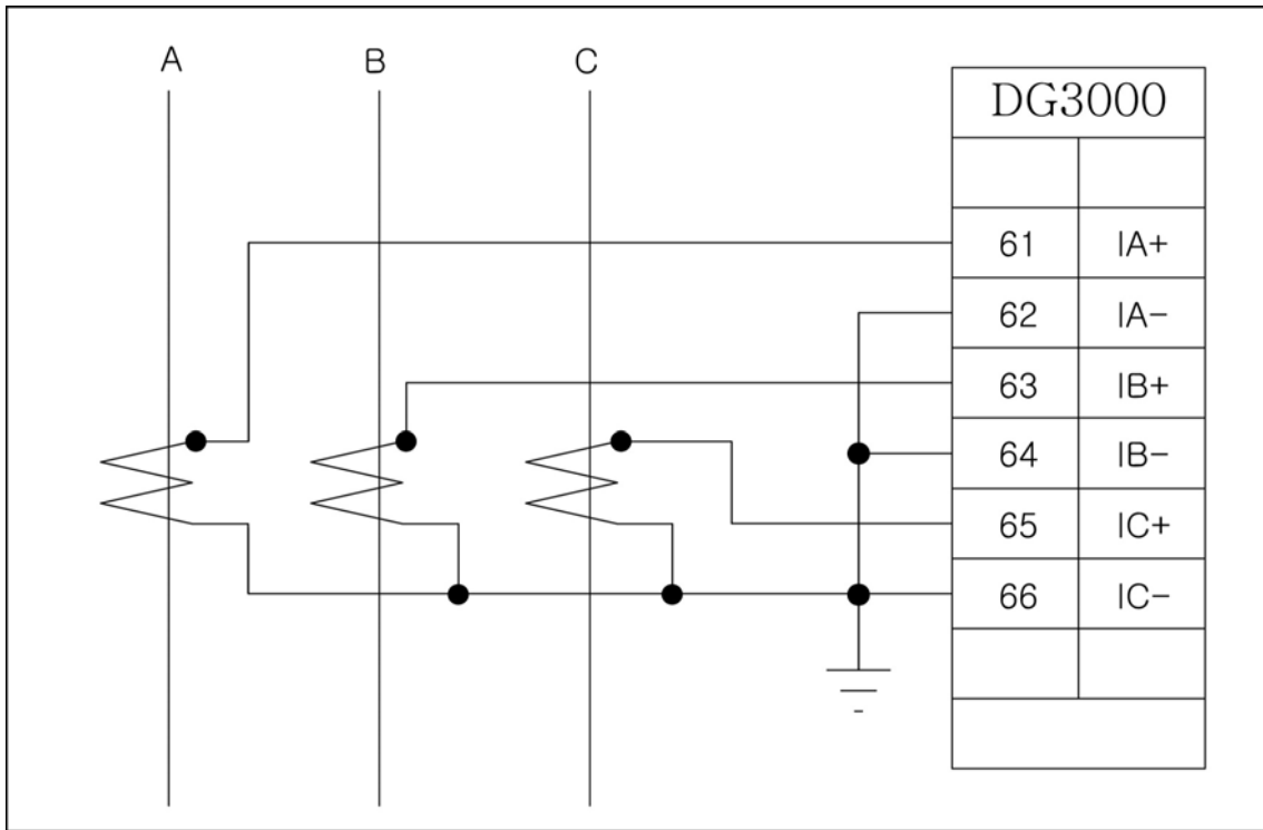
<그림 81. 3상 3선식 3CT 결선 - ABC Rotation>
