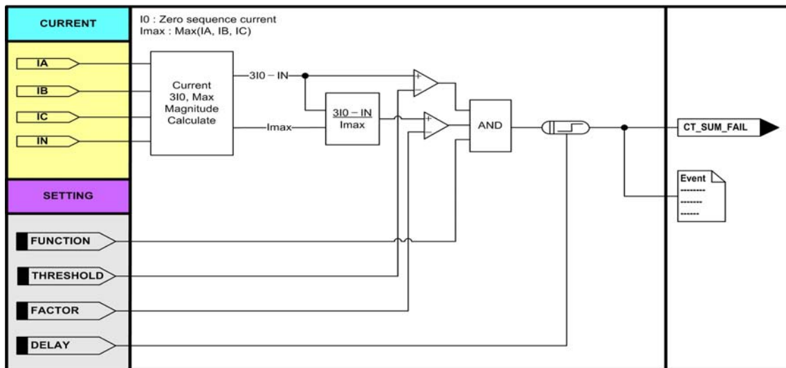
<그림 8. 전류입력회로 감시 동작특성>
