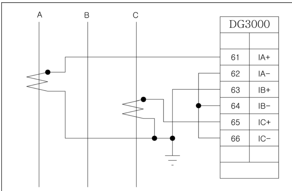
<그림 80. 3상 3선식 2CT 결선 - ABC Rotation>
