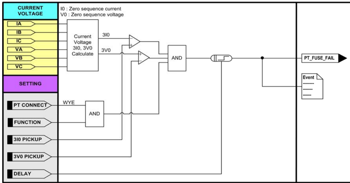
<그림 6. PT Fuse 감시 동작특성>
