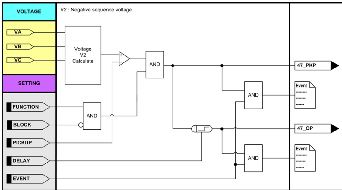
<그림 27. 역상 과전압보호 동작특성>
