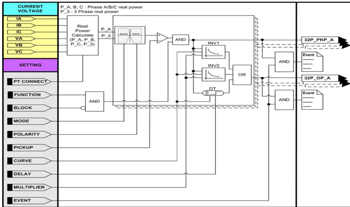
<그림 31. 역전력 보호 동작특성>
