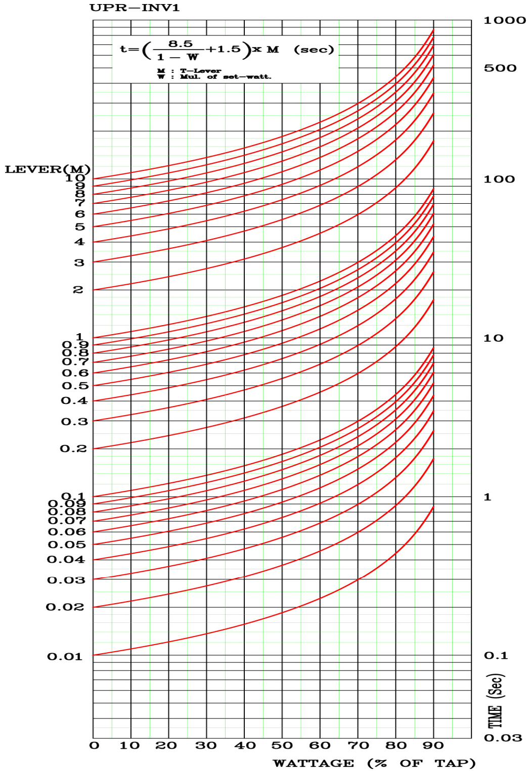
<부도 1.19 저전력 역반한시 특성 곡선>
