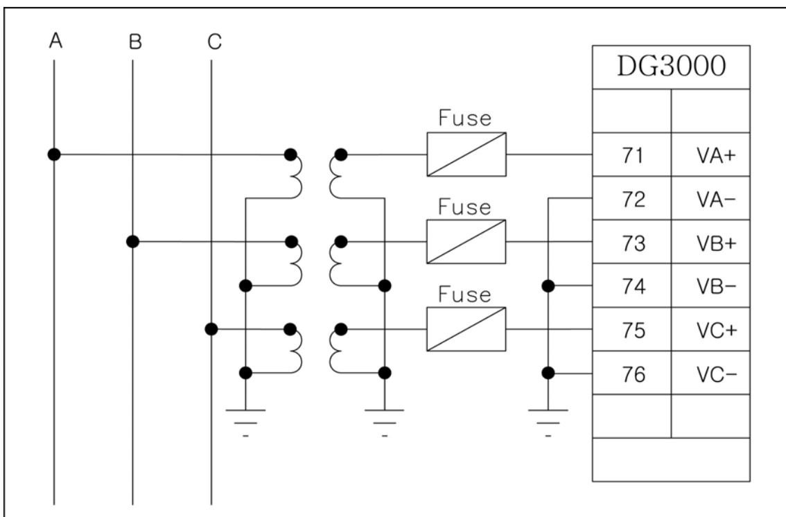
<그림 76. 3상 3선식 3PT 결선 - ABC Rotation>
