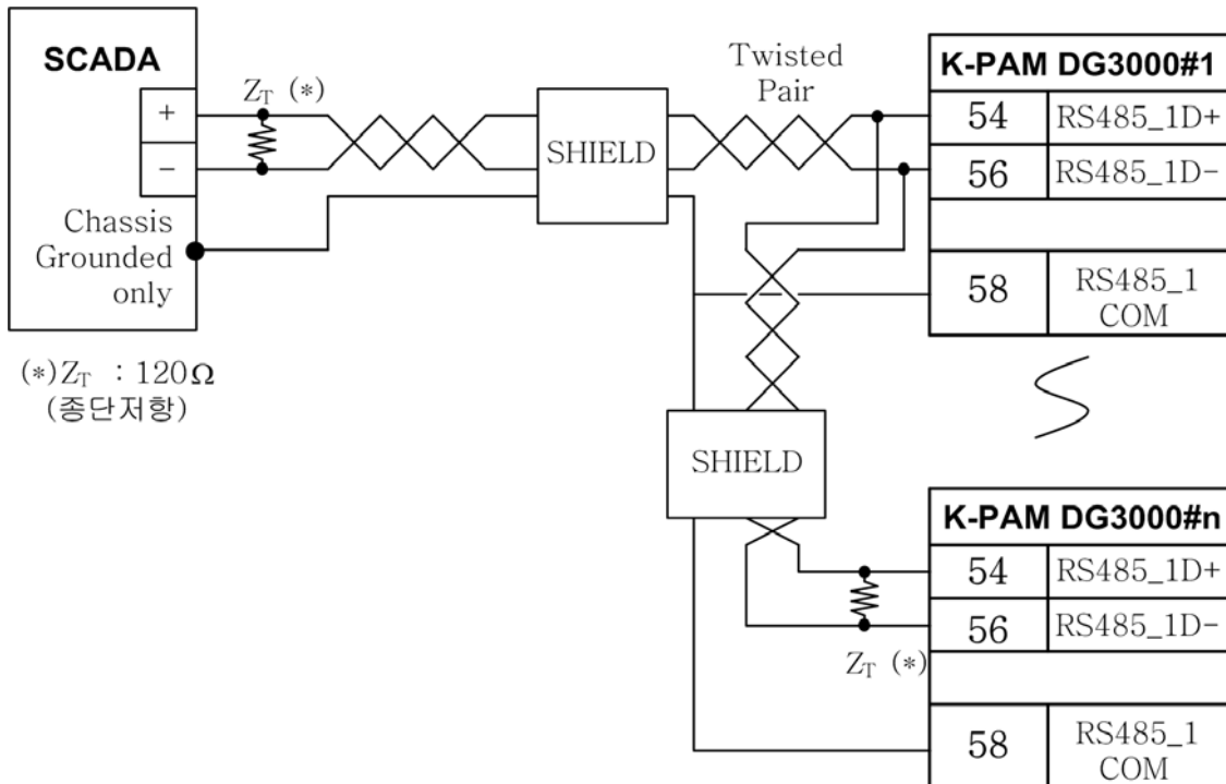
<그림 86. RS-485C 통신포트 결선도>
