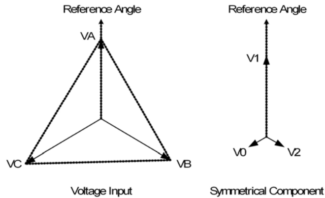
<그림 71. Sequence 전압>
