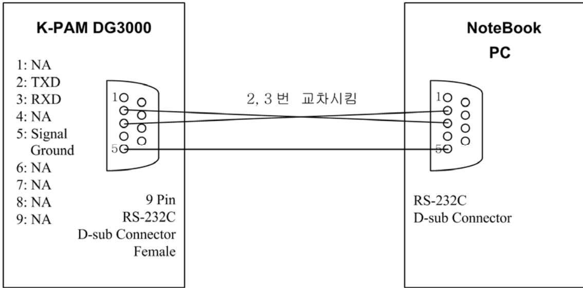
<그림 85. RS-232C 통신포트 결선도>
