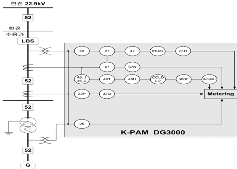
<그림 1. 기능 단선도>
