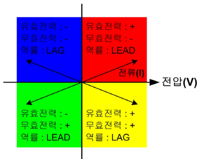
<그림 5. DG3000 유효/무효전력의 부호 및 역률 표시>
