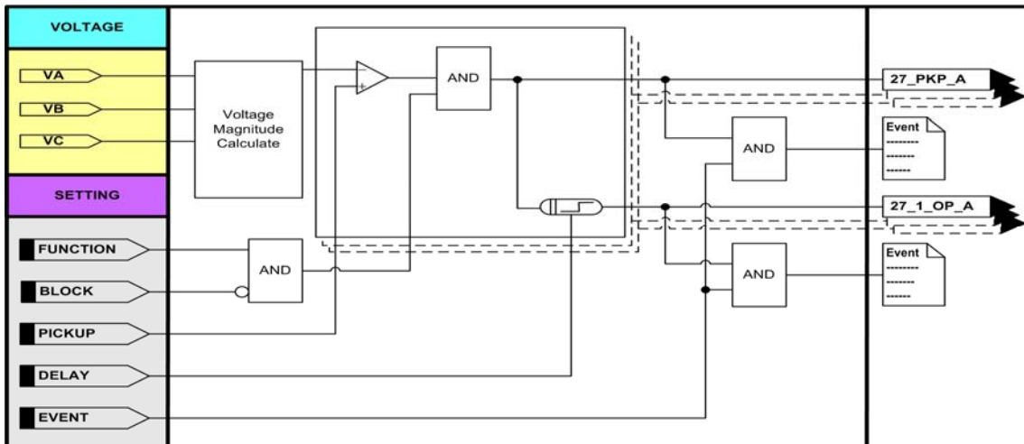
<그림 25. 순시/정한시 저전압보호 동작특성>
