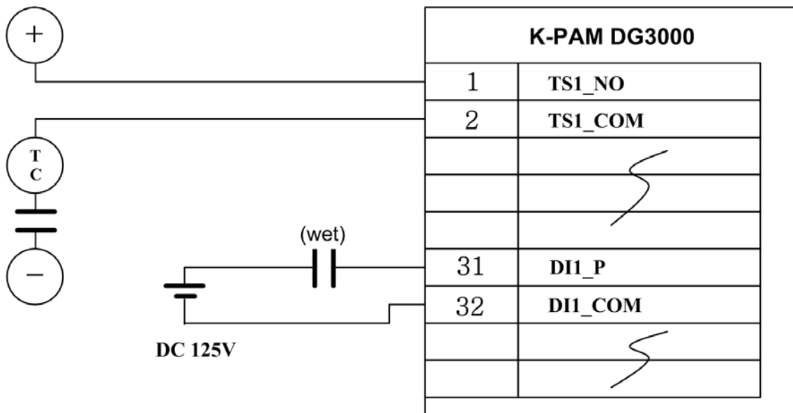
<그림 84. 입력/출력접점 결선도>
