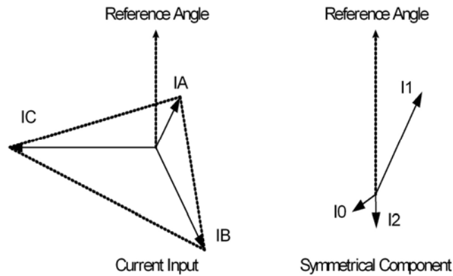
<그림 72. Sequence 전류>
