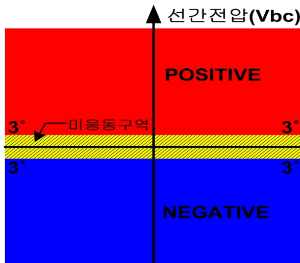
<그림 34. 무효전력 보호요소의 IA상에 대한 동작 영역>
