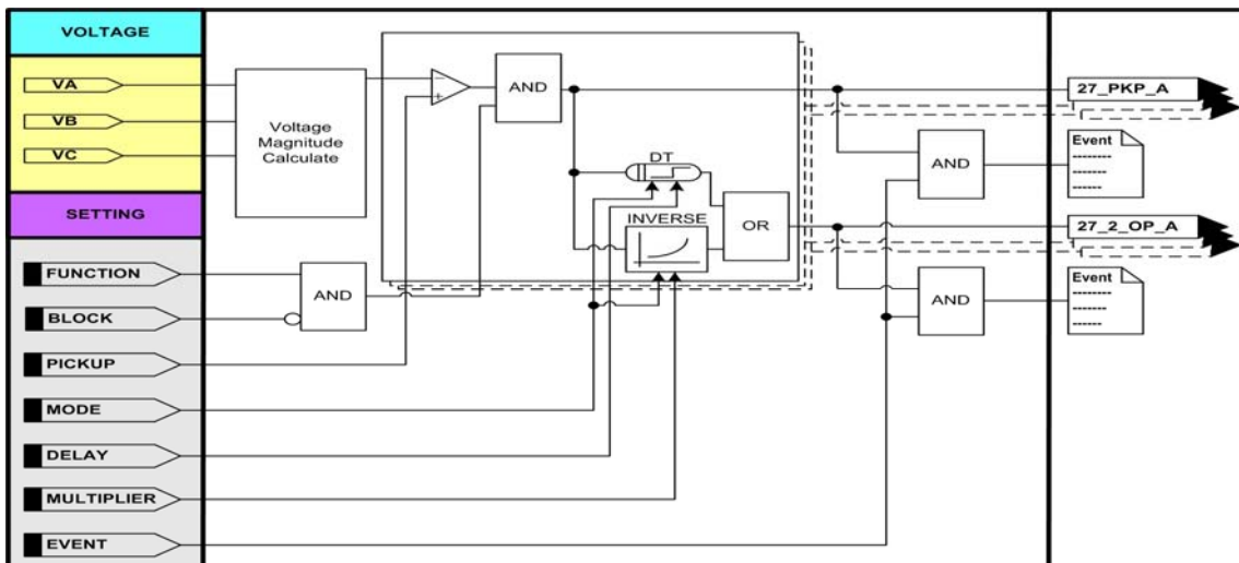
<그림 26. 한시 저전압보호 동작특성>
