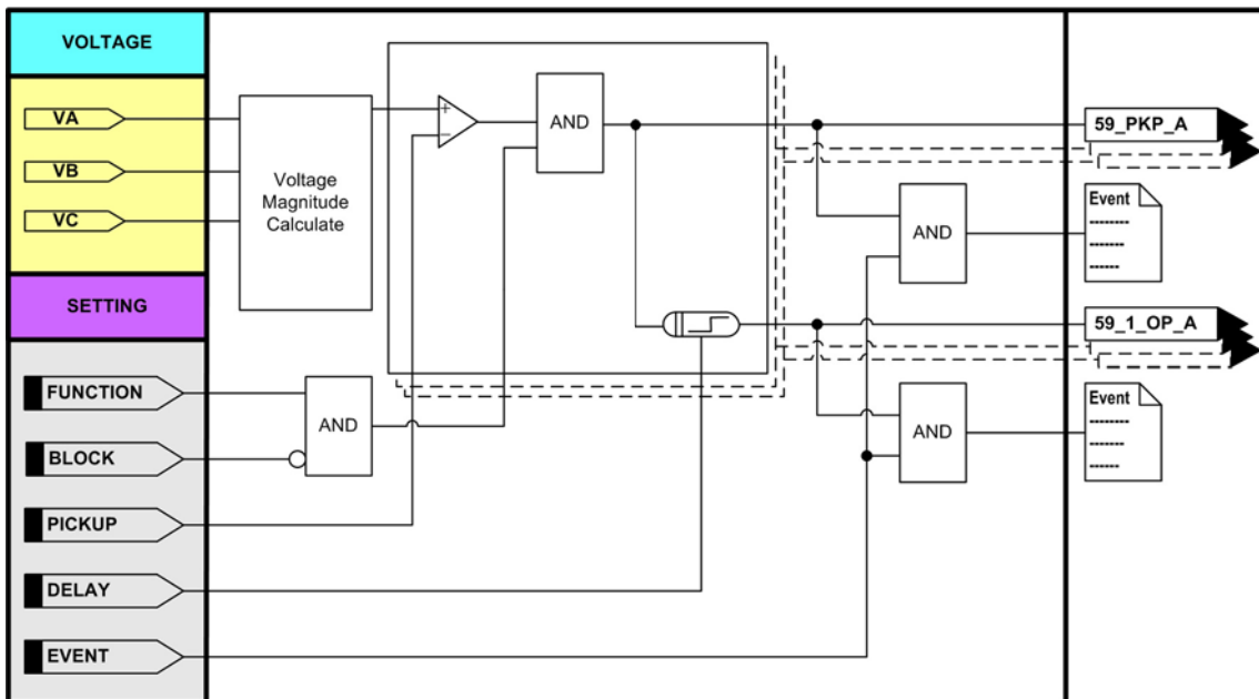
<그림 23. 순시/정한시 과전압보호 동작특성>
