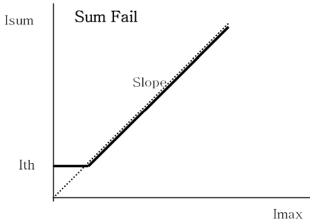
<그림 7. 전류입력회로 감시 특성 Curve>
