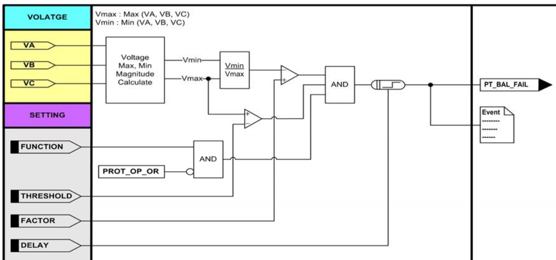
<그림 10. 전압불평형 감시 동작특성>
