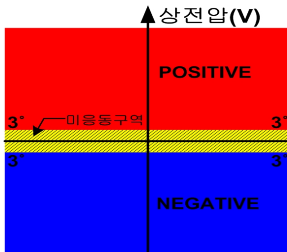
<그림 30. 역전력 보호요소의 동작 영역>
