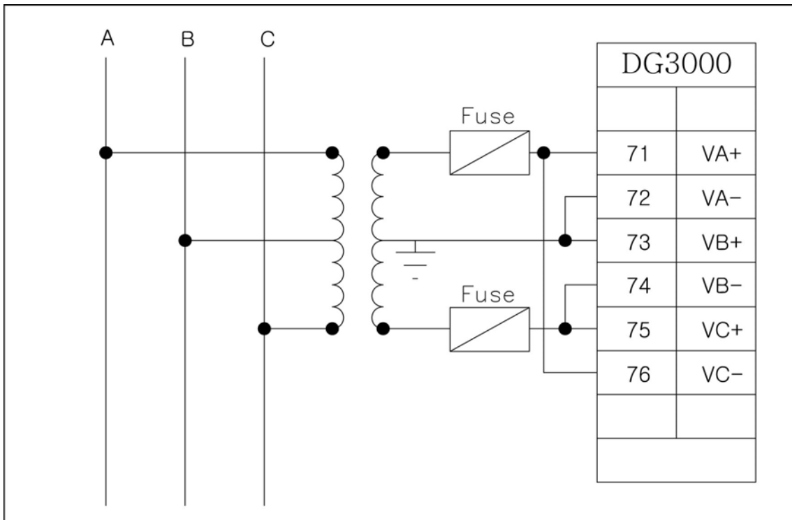
<그림 75. 3상 3선식 V 결선 - ABC Rotation>
