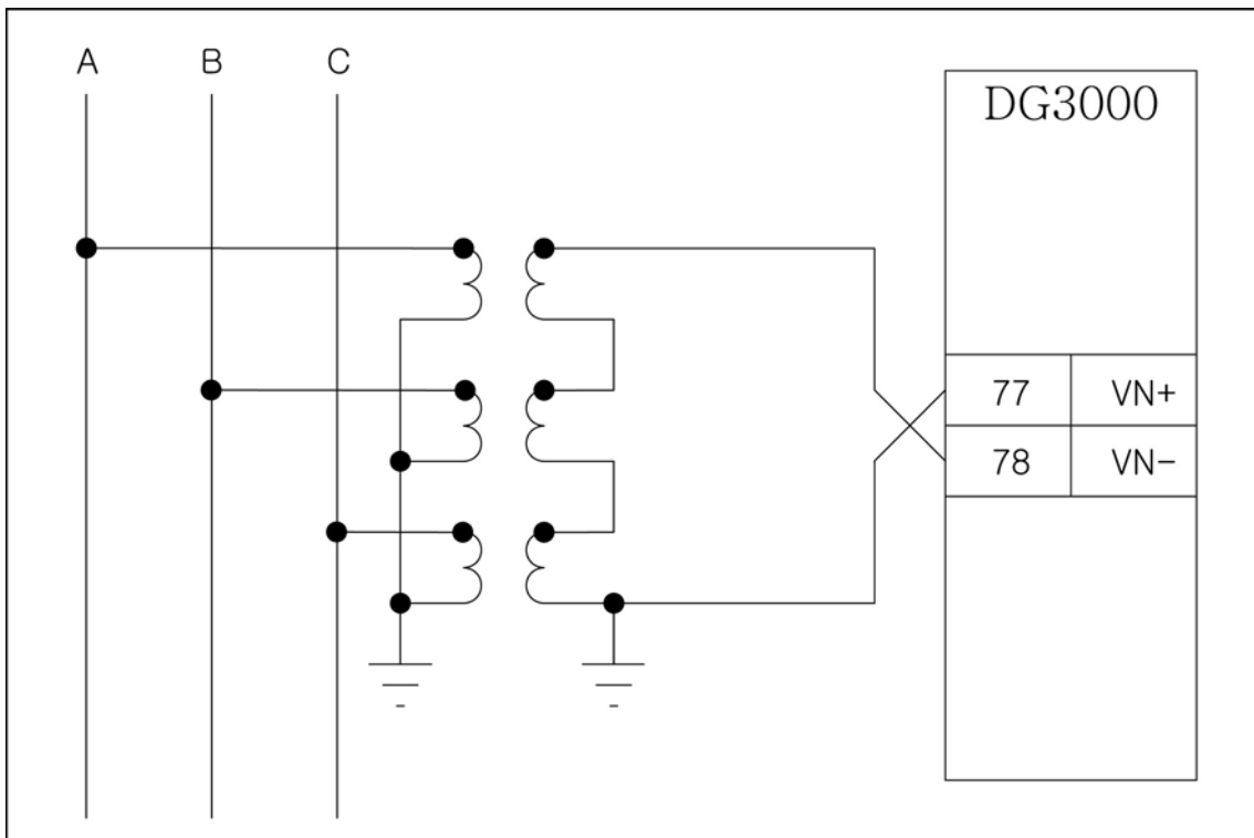
<그림 78. GPT 결선 >
