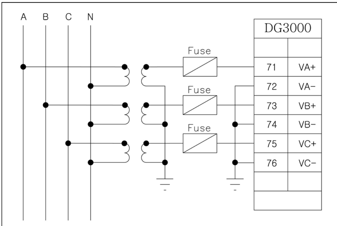
<그림 77. 3상 4선식 3PT 결선 - ABC Rotation>
