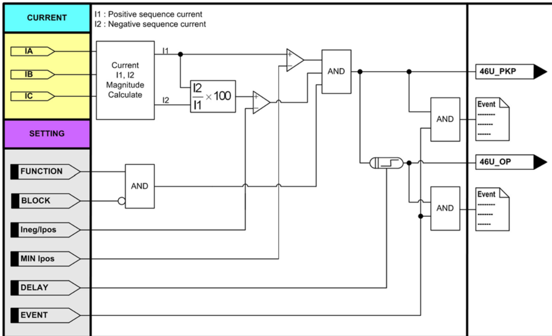
<그림 22. 전류 불평형(결상)보호 동작특성>
