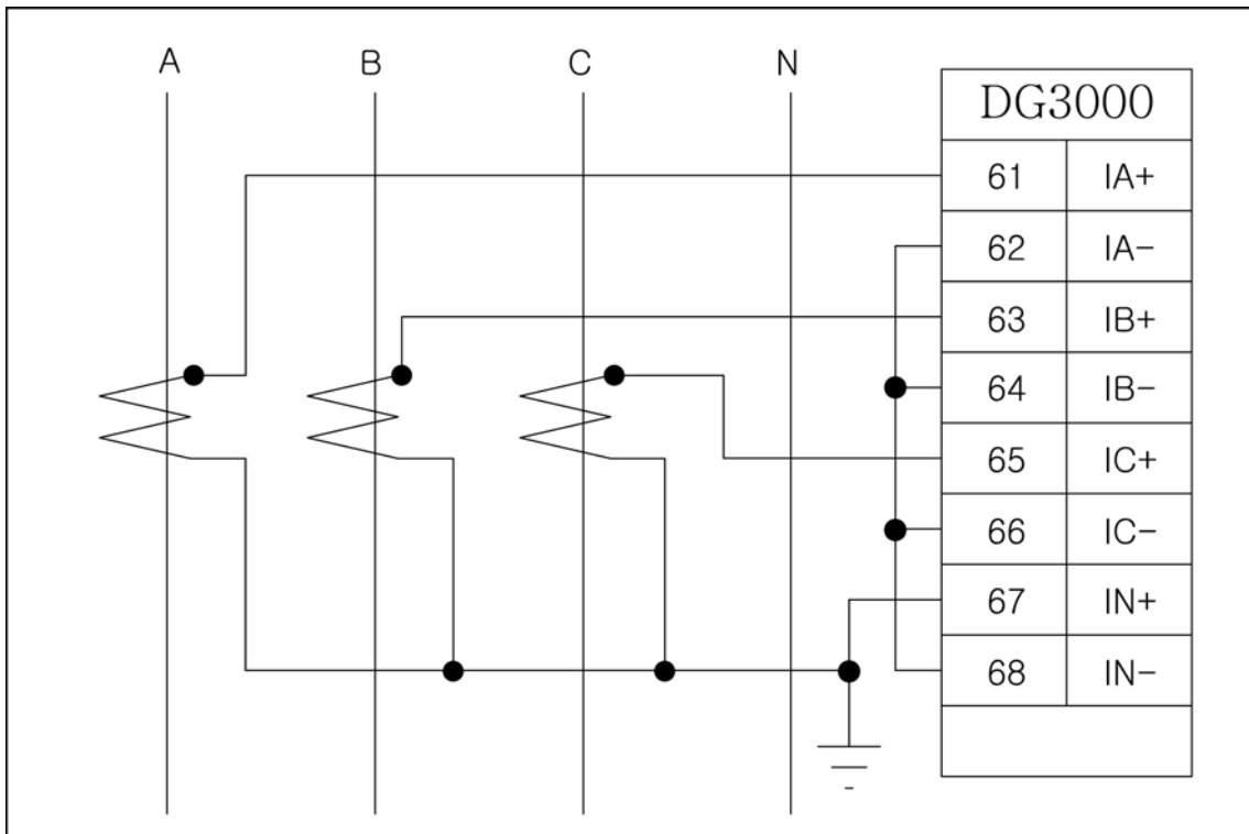
<그림 82. 3상 4선식 3CT 잔류회로 결선 - ABC Rotation>
