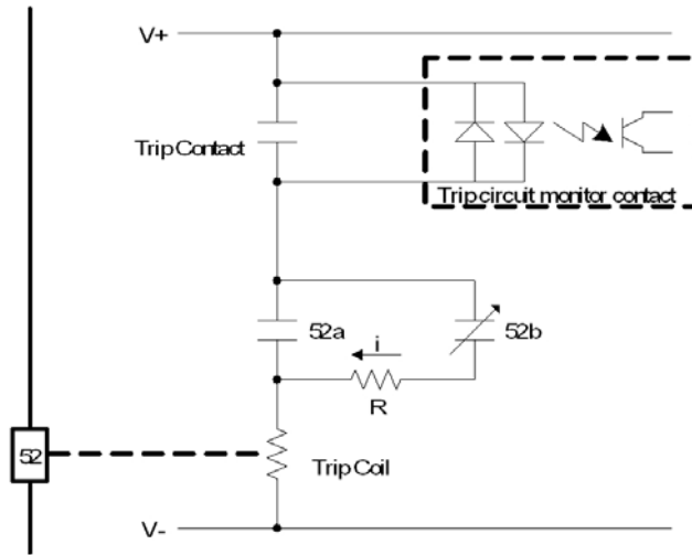
<그림 13. TCS 회로 구성>
