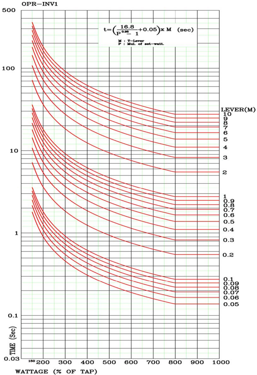
<부도 1.17 과전력 반한시_1 특성 곡선>
