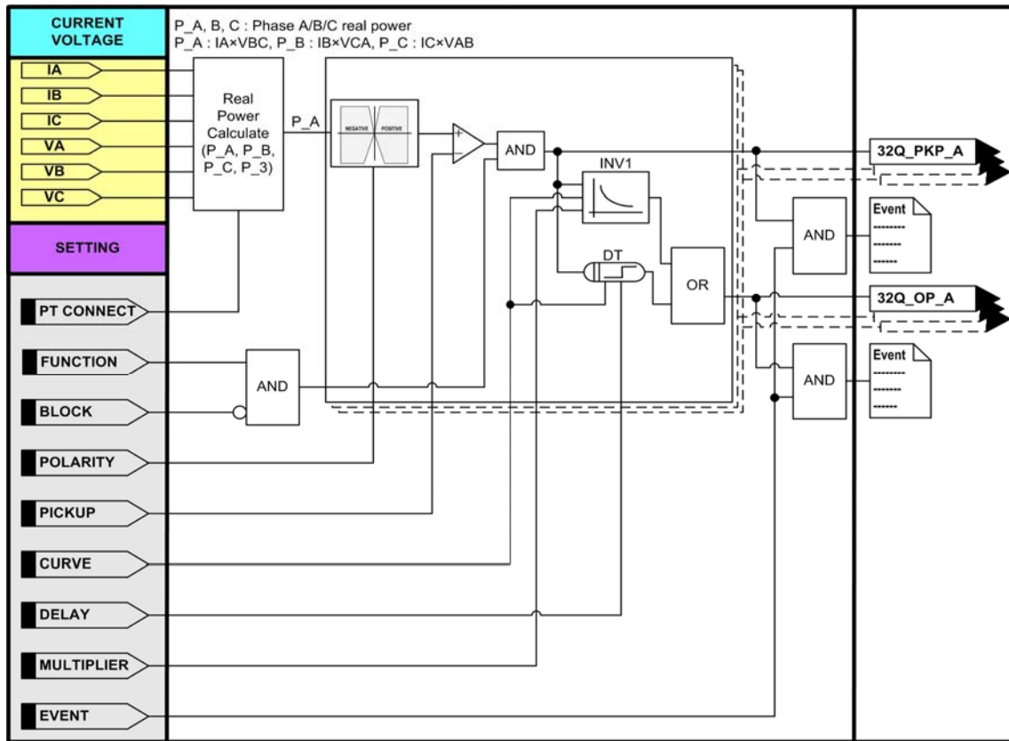
<그림 35. 무효전력 보호 동작특성>
