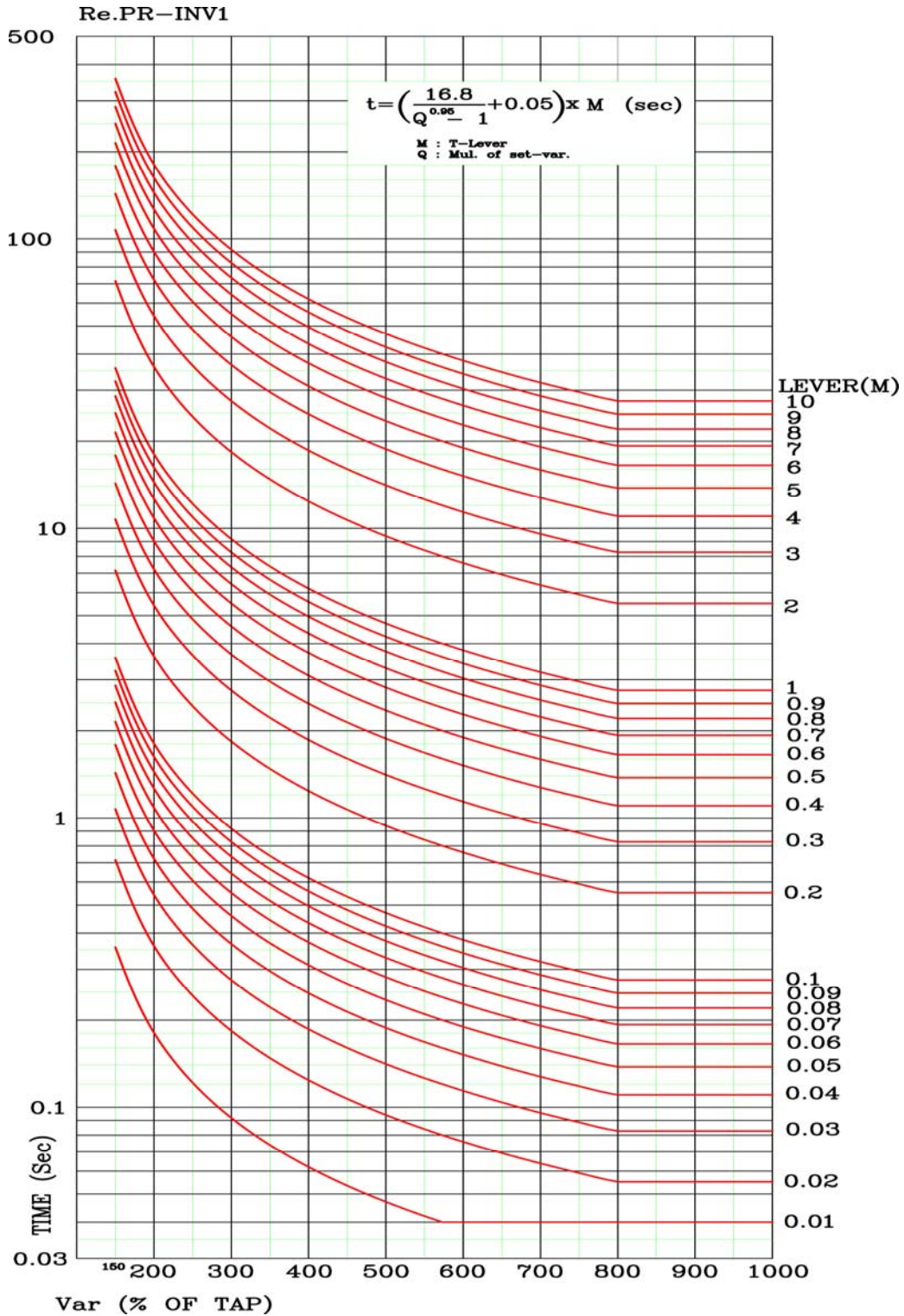
<부도 1.20 무효전력 반한시 특성 곡선>
