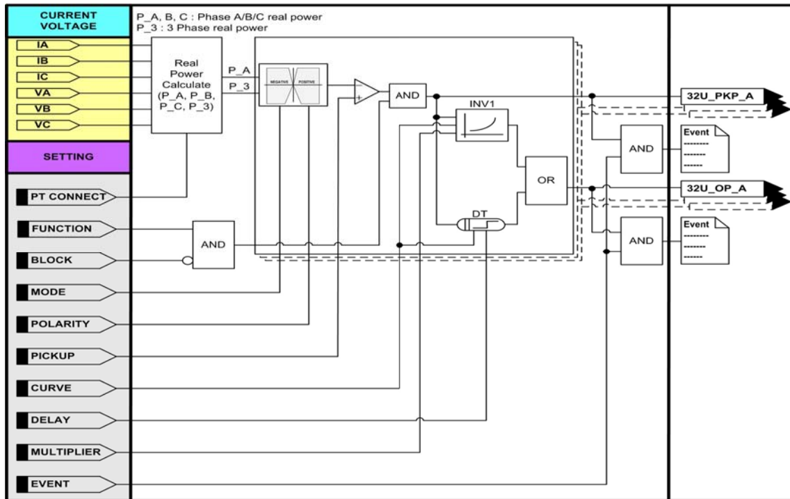
<그림 33. 저전력 보호 동작특성>
