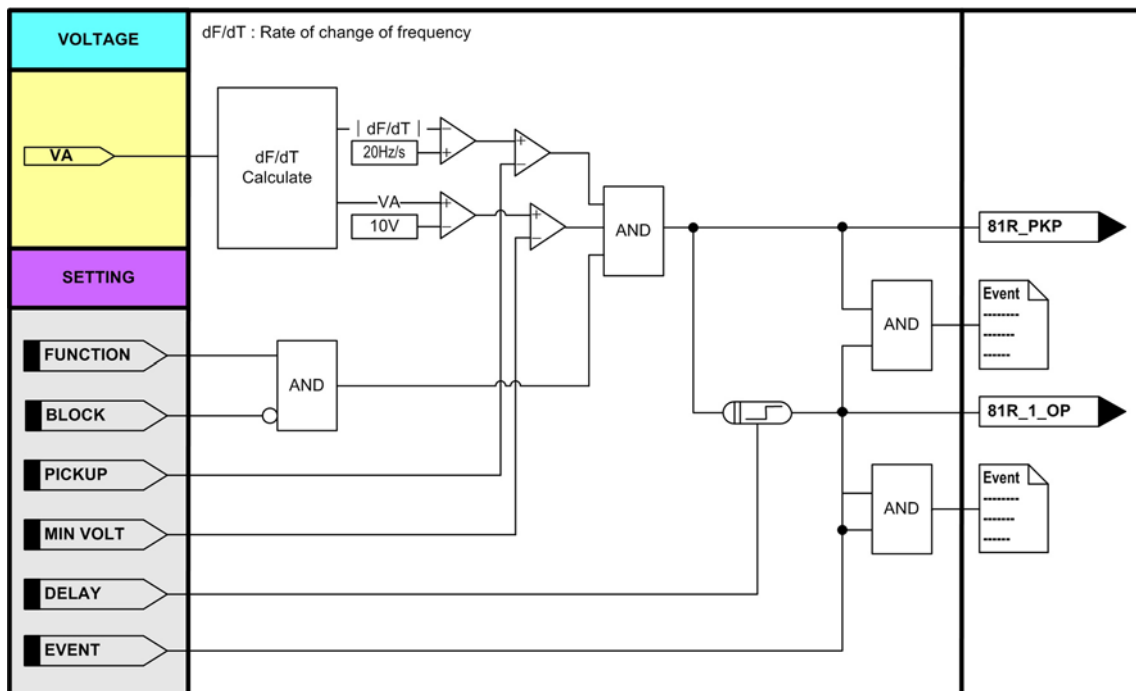
<그림 29. 주파수 변동률보호 동작특성>
