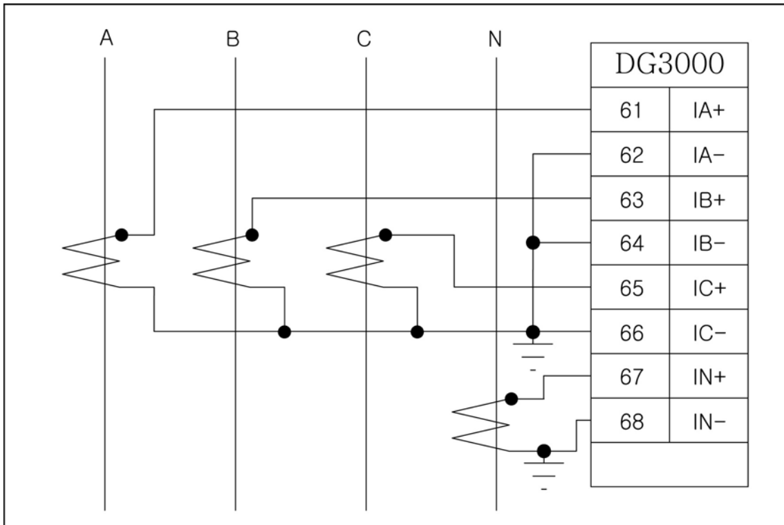
<그림 83. 3상 4선식 4CT 결선 - ABC Rotation>
