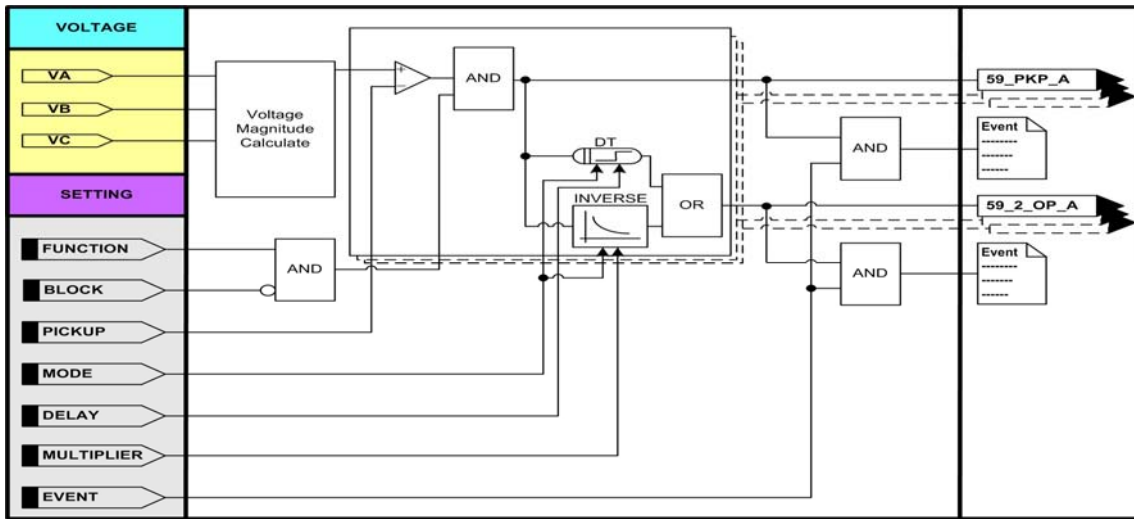
<그림 24. 한시 과전압보호 동작특성>
