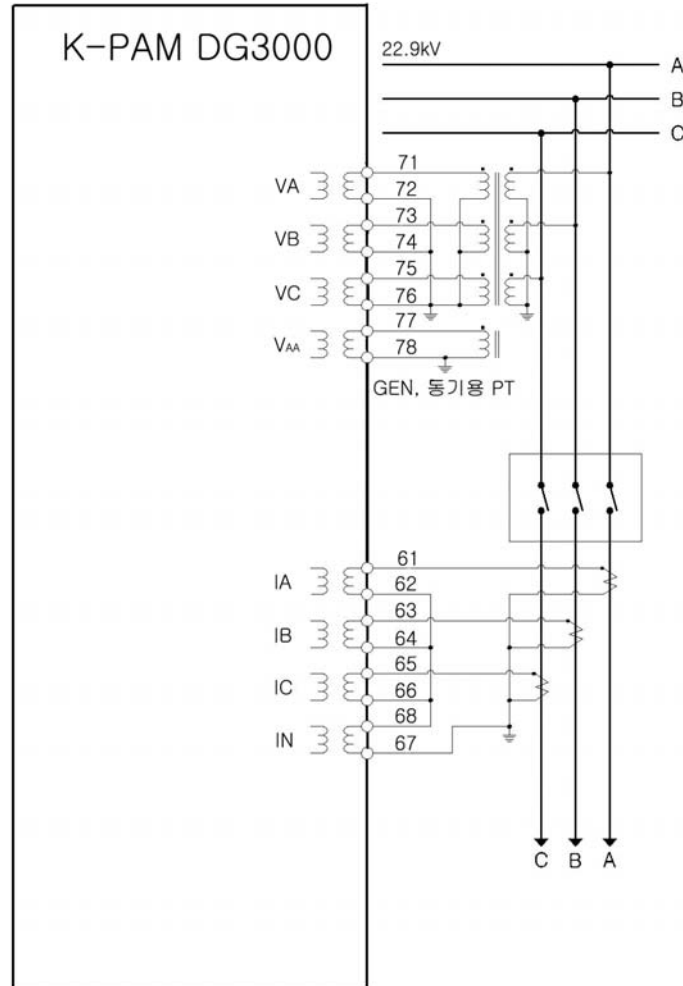
<그림 70. 적용 예시 결선도>
