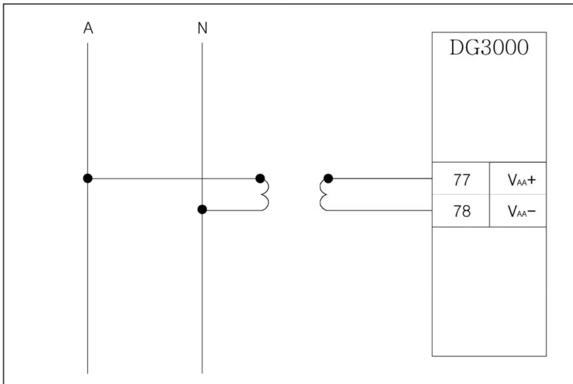
<그림 79. GEN. 동기 PT 결선 >
