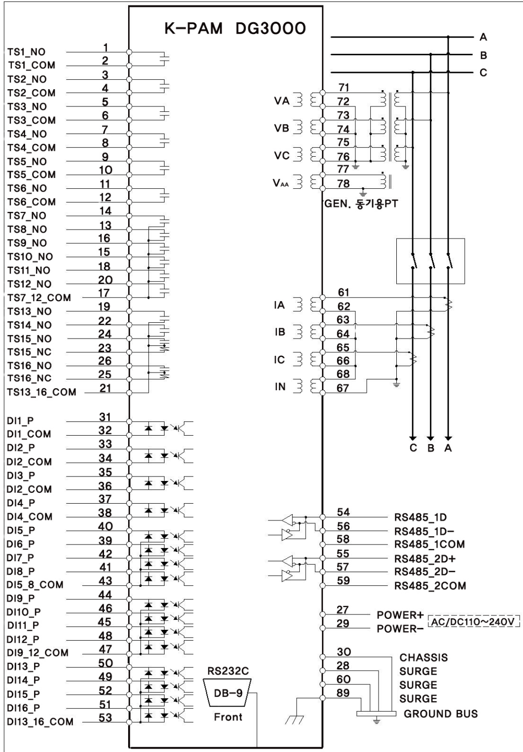
<그림 74. K-PAM DG3000 PT/CT 결선도>
