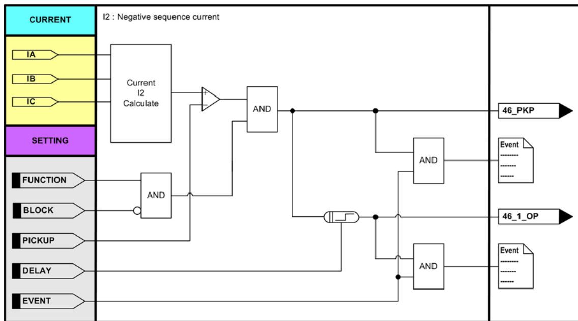
<그림 20. 순시/정한시 역상 과전류보호 동작특성>
