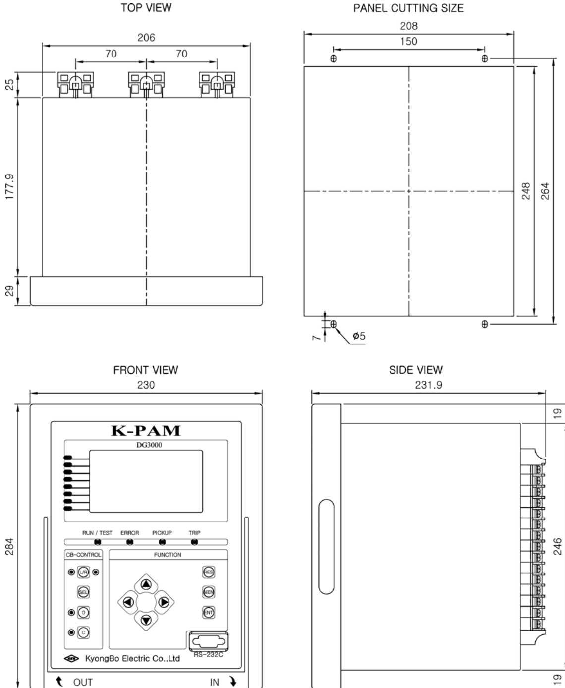
<그림 73. K-PAM DG3000 치수도>
