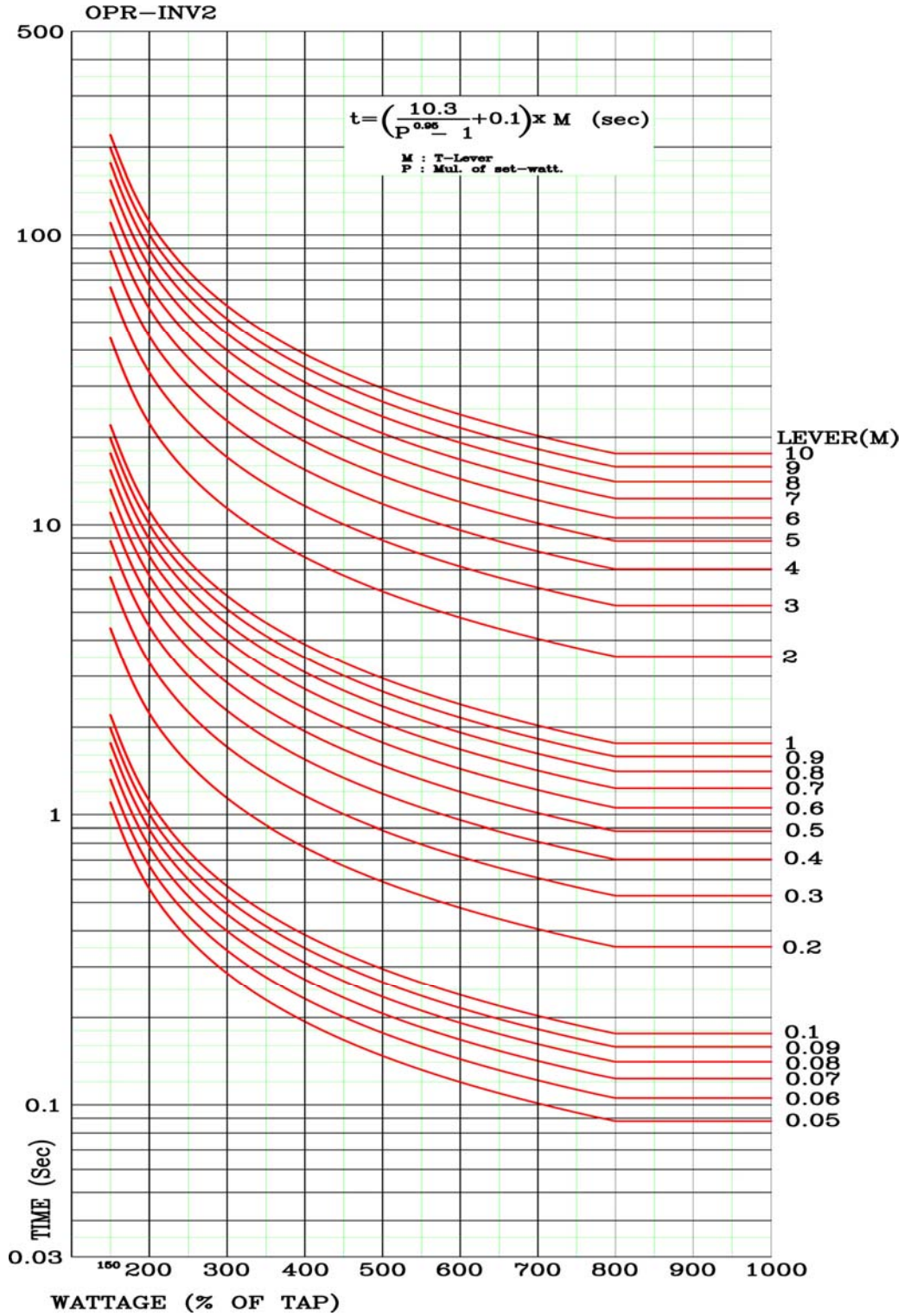
<부도 1.18 과전력 반한시_2 특성 곡선>
