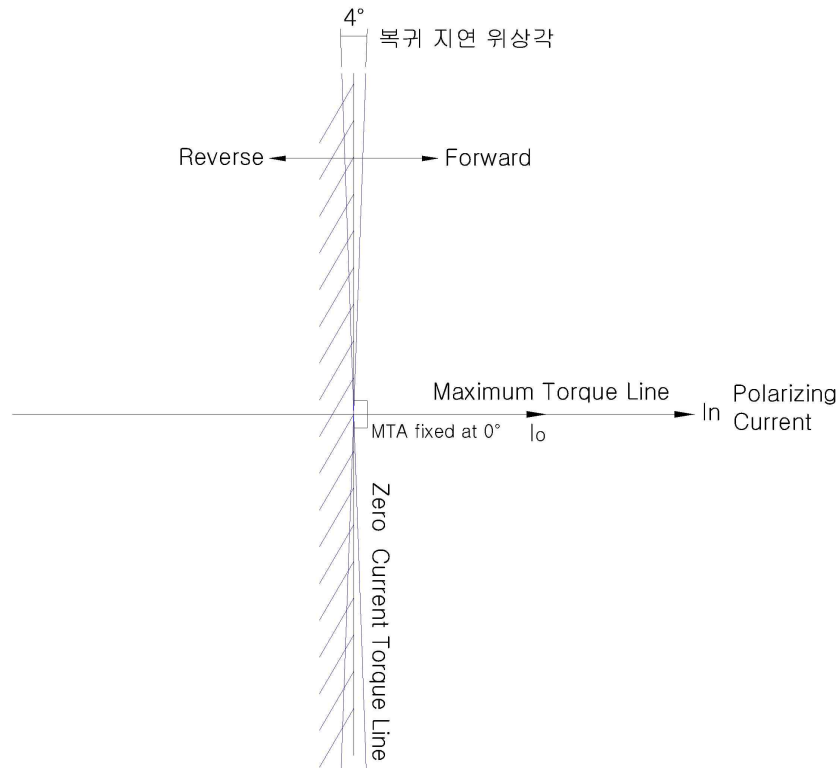
<Figure 24. 기준 Polarizing을 Current 로 하였을 때의 동작 특성>
