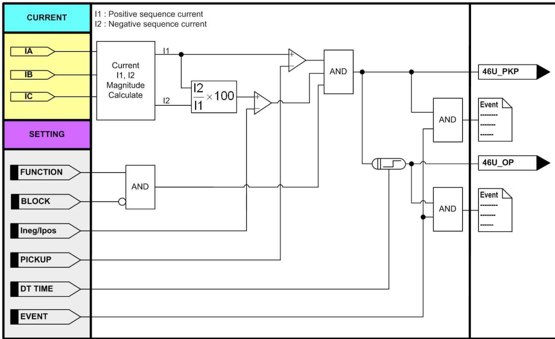
<Figure 29. 전류 불평형(결상)보호 동작특성>
