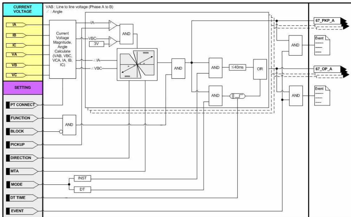
<Figure 21. 순시/정한시 방향성 과전류보호 동작특성>
