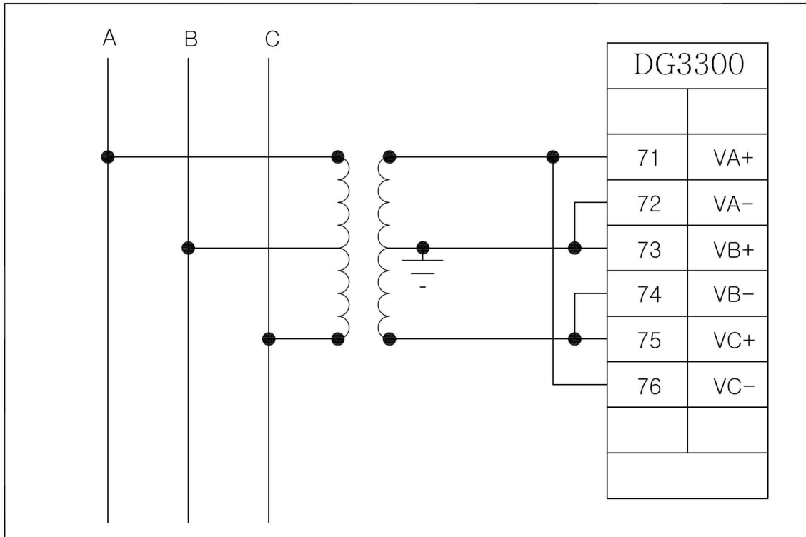
<Figure 98. 3상 3선식 V 결선 - ABC Rotation>
