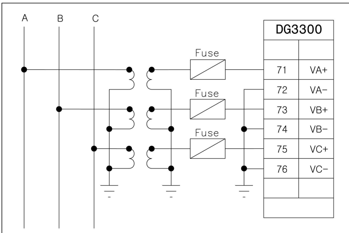
<Figure 99. 3상 3선식 3PT 결선 - ABC Rotation>
