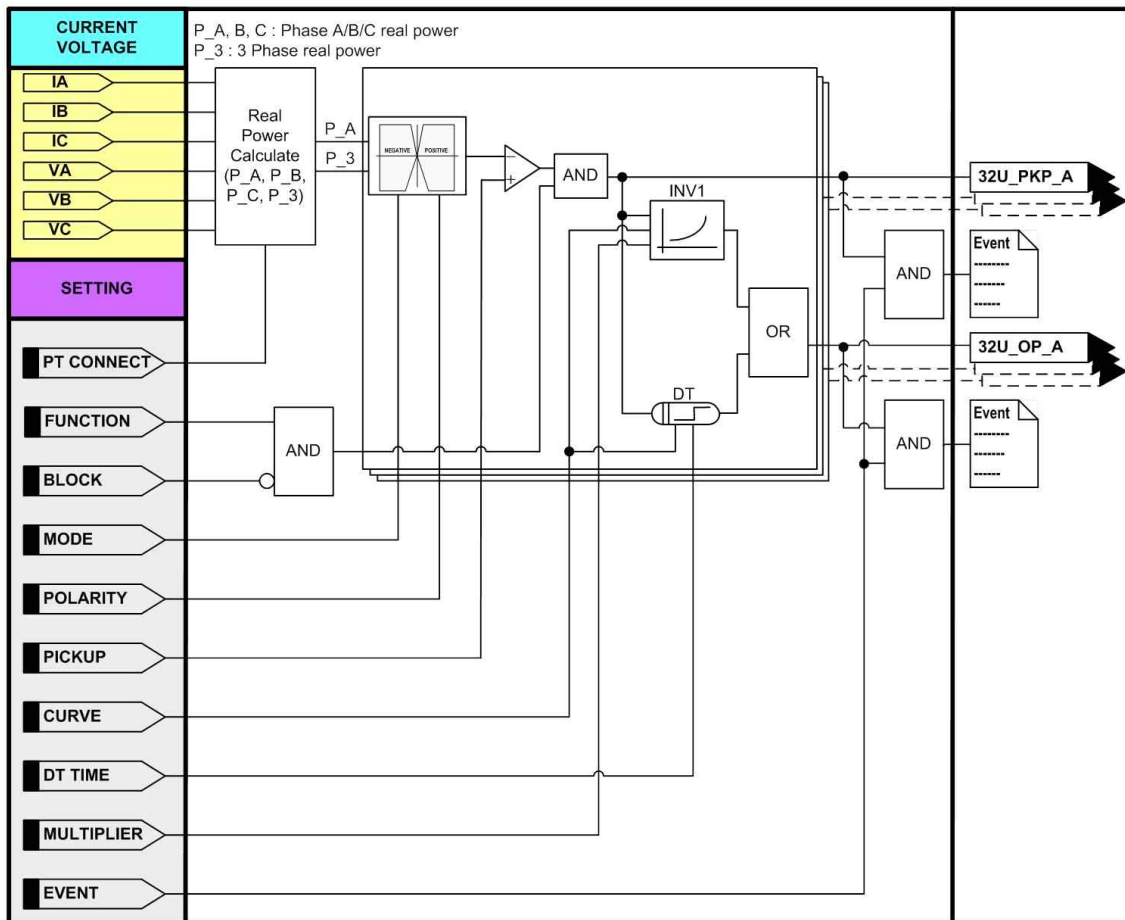
<Figure 40. 저전력 보호 동작특성>
