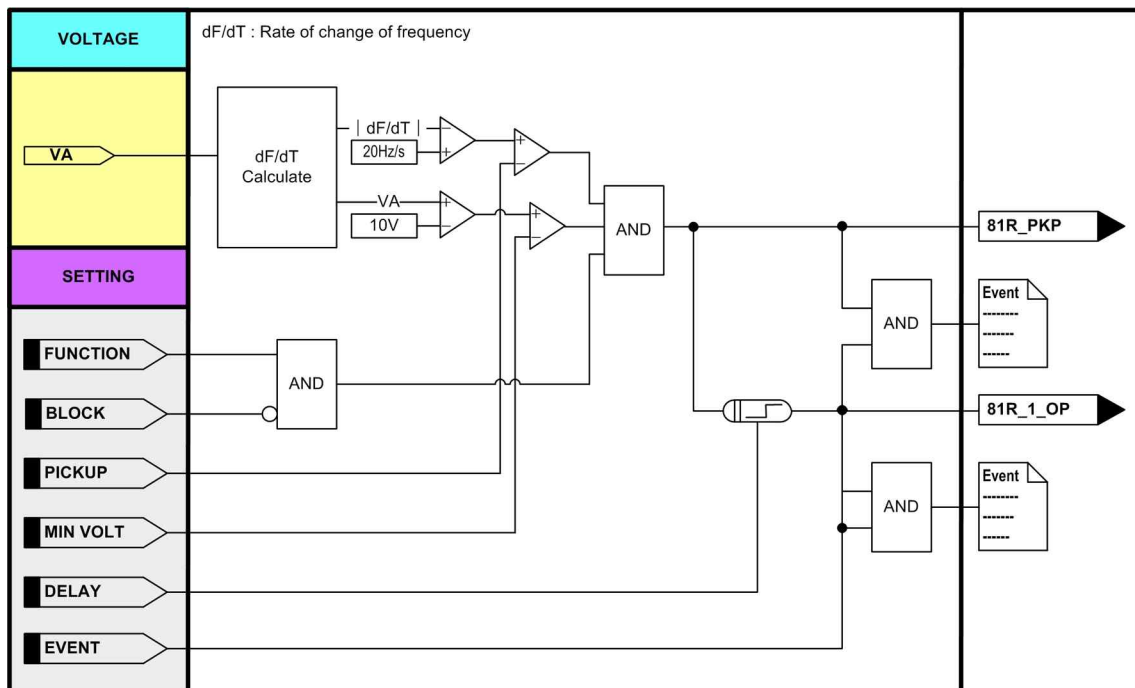
<Figure 36. 주파수 변동률보호 동작특성>
