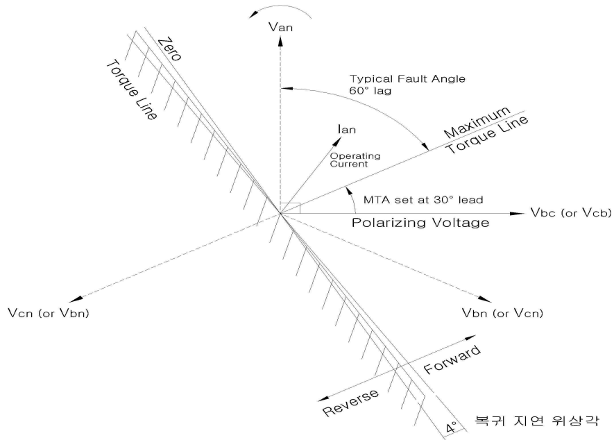
<Figure 20. A상 전류의 동작 특성>
