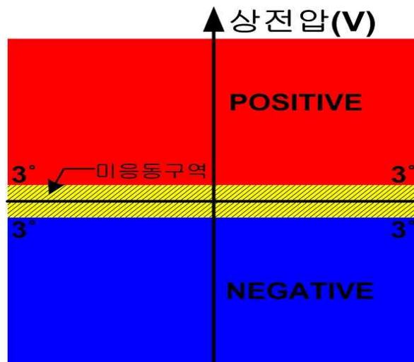
<Figure 37. 역전력 보호요소의 동작 영역>
