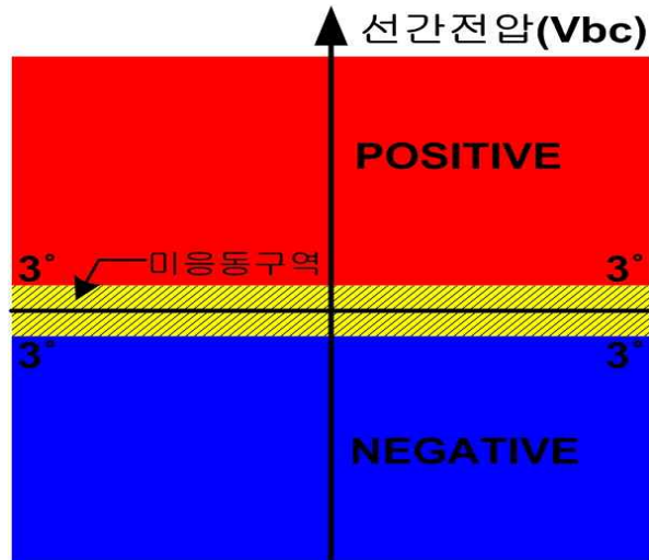
<Figure 41. 무효전력 보호요소의 IA상에 대한 동작 영역>
