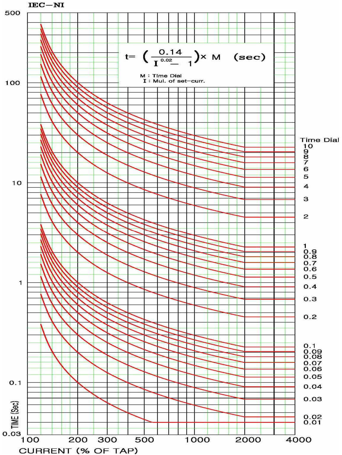
<부도 1.1 과전류/지락과전류/역상과전류 IEC_NI 특성 곡선>
