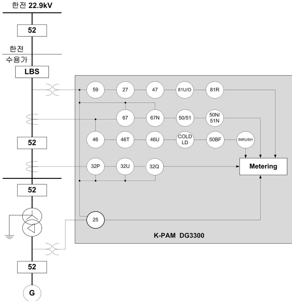
<Figure 1. 기능 단선도>
