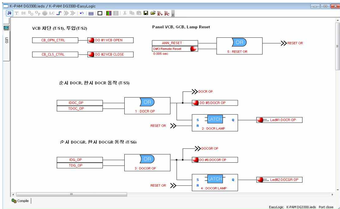
<Figure 71. EasyLogic 구성 예>
