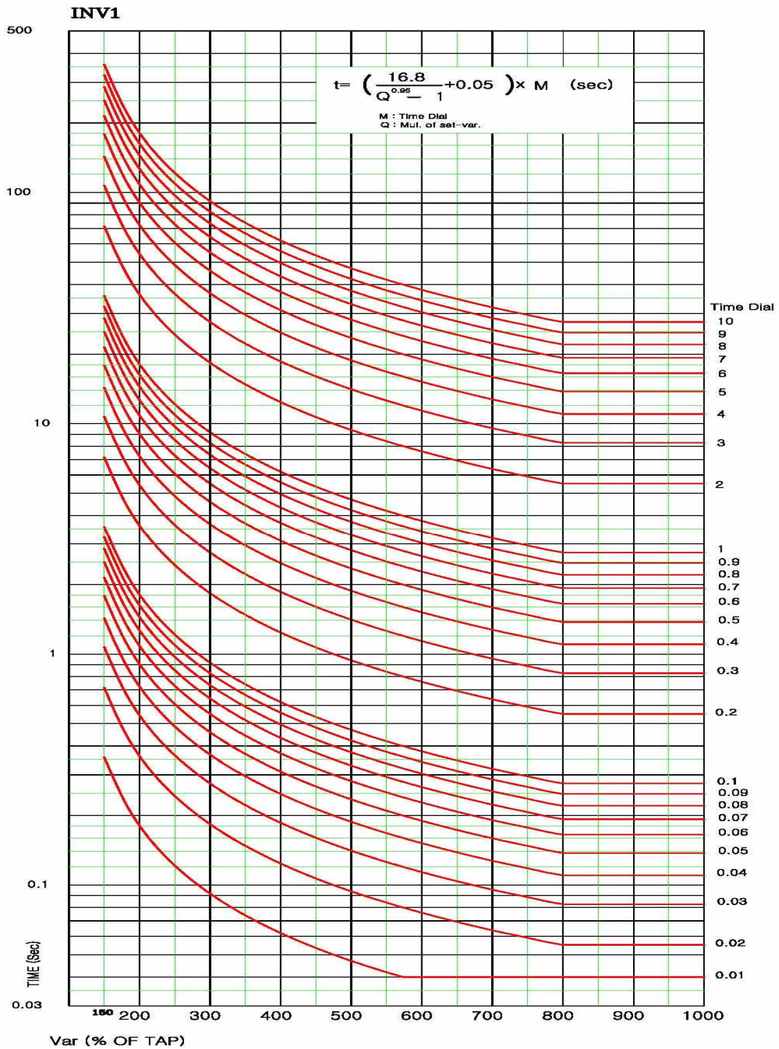
<부도 1.20 무효전력 반한시 특성 곡선>
