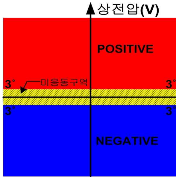
<Figure 39. 저전력 보호요소의 동작 영역>
