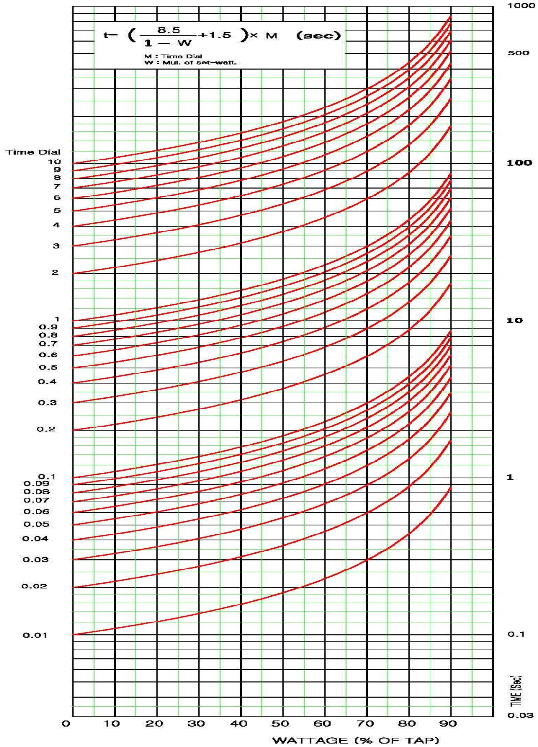
<부도 1.19 저전력 역반한시 특성 곡선>
