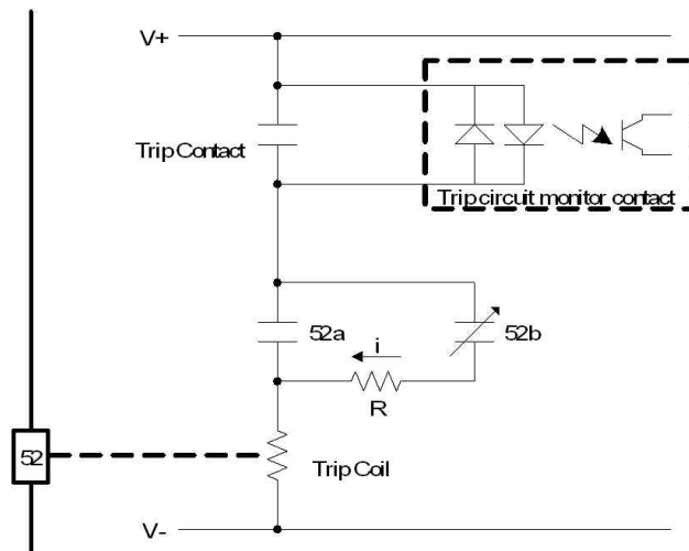
<Figure 13. TCS 회로 구성>
