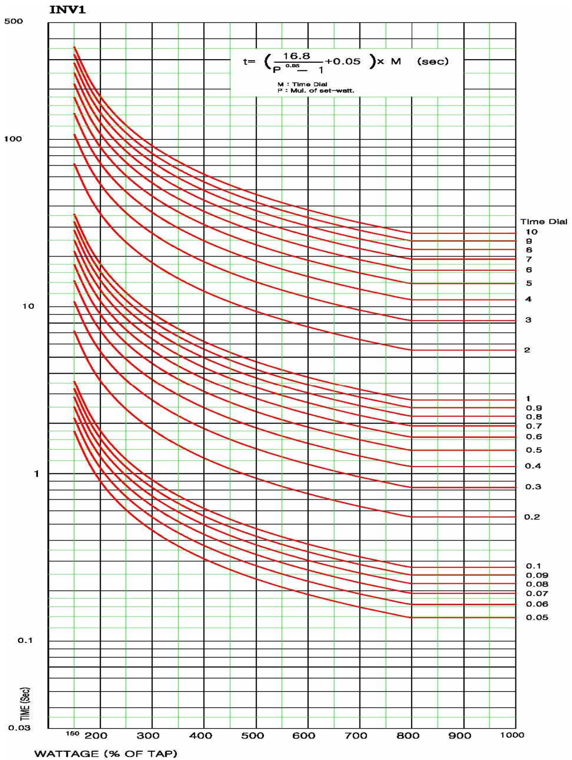
<부도 1.17 과전력 반한시_1 특성 곡선>
