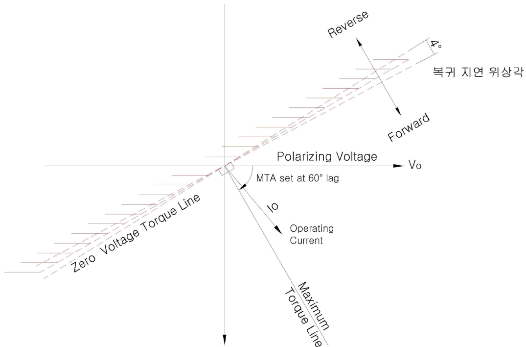
<Figure 23. 기준 Polarizing을 Voltage 로 하였을 때의 동작 특성>
