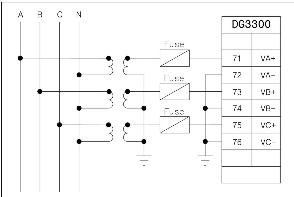
<Figure 100. 3상 4선식 3PT 결선 - ABC Rotation>
