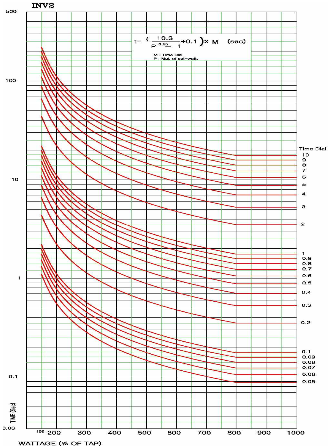
<부도 1.18 과전력 반한시_2 특성 곡선>
