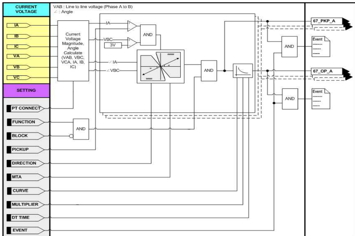
<Figure 22. 한시 방향성 과전류보호 동작특성>
