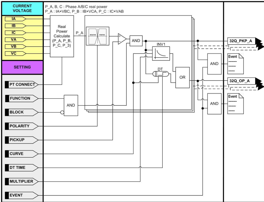
<Figure 42. 무효전력 보호 동작특성>
