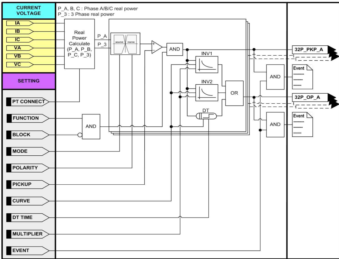
<Figure 38. 역전력 보호 동작특성>
