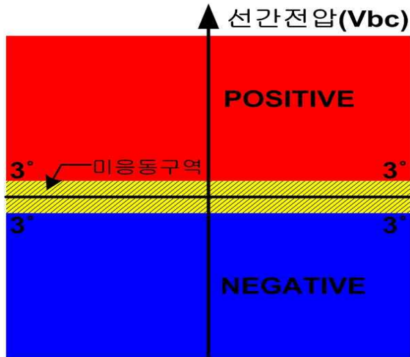
<Figure 41. 무효전력 보호요소의 IA상에 대한 동작 영역>
