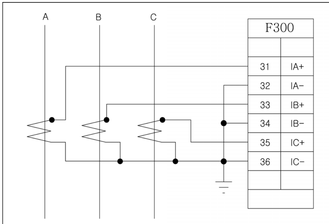
<그림 39. 3상 3선식 3CT결선 - ABC Rotation>
