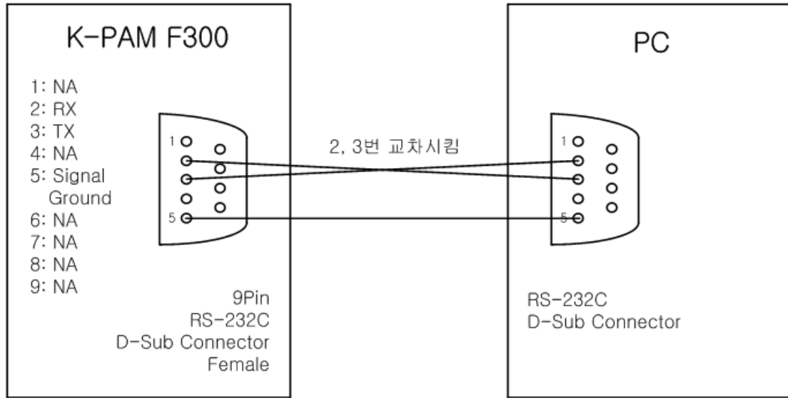
<그림 44. RS-232C 통신 포트 결선도>
