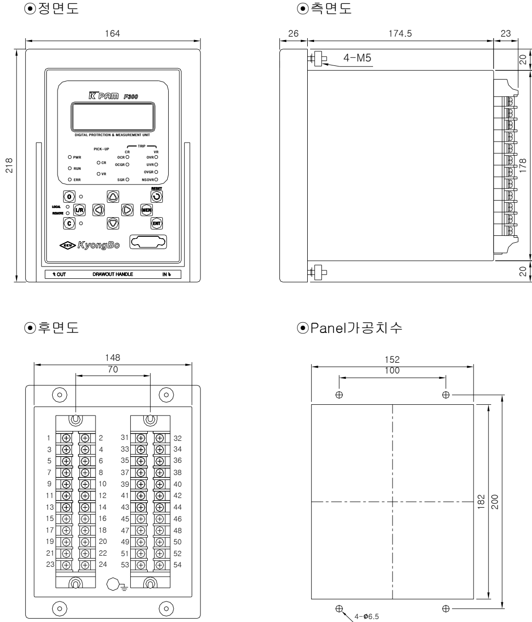
<그림 33. K-PAM F300 치수도>
