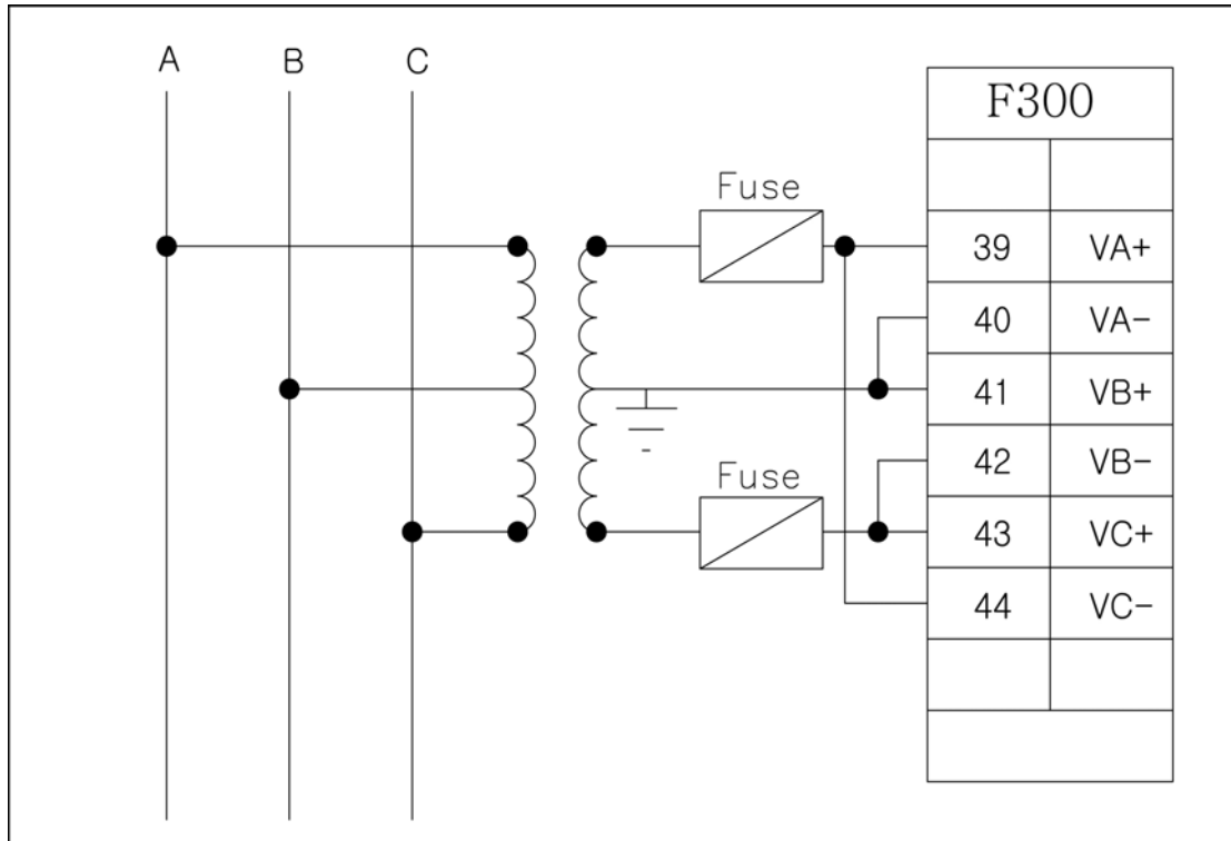
<그림 34. 3상 3선식 V결선 - ABC Rotation>
