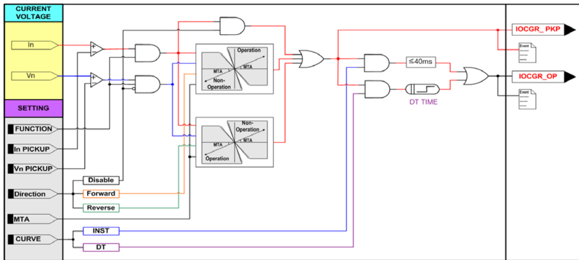
< 그림 9. (방향성) 순시/정한시 지락과전류보호 동작특성 >
