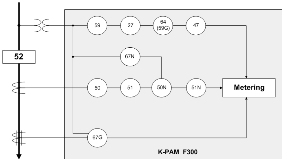
< 그림 1. 기능 단선도 >
