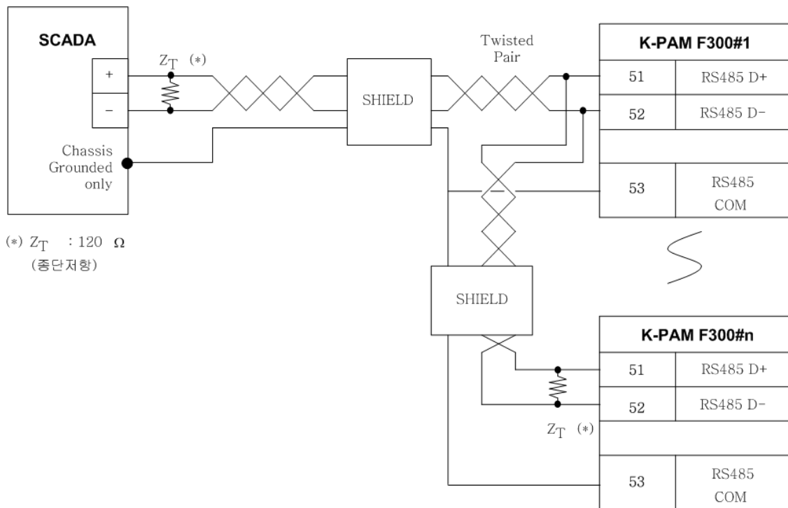
<그림 45. RS-485 통신 포트 결선도>
