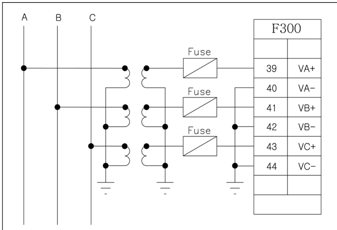
<그림 35. 3상 3선식 3PT결선 - ABC Rotation>
