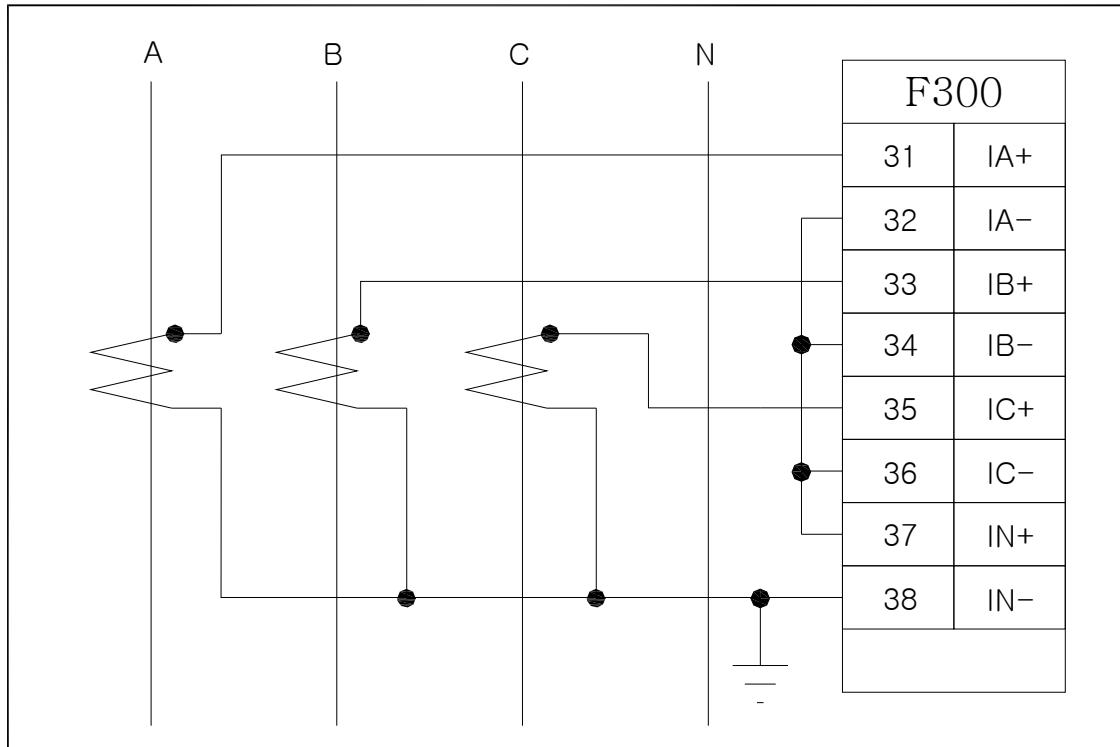
<그림 40. 3상 4선식 3CT 잔류회로 결선 - ABC Rotation>
