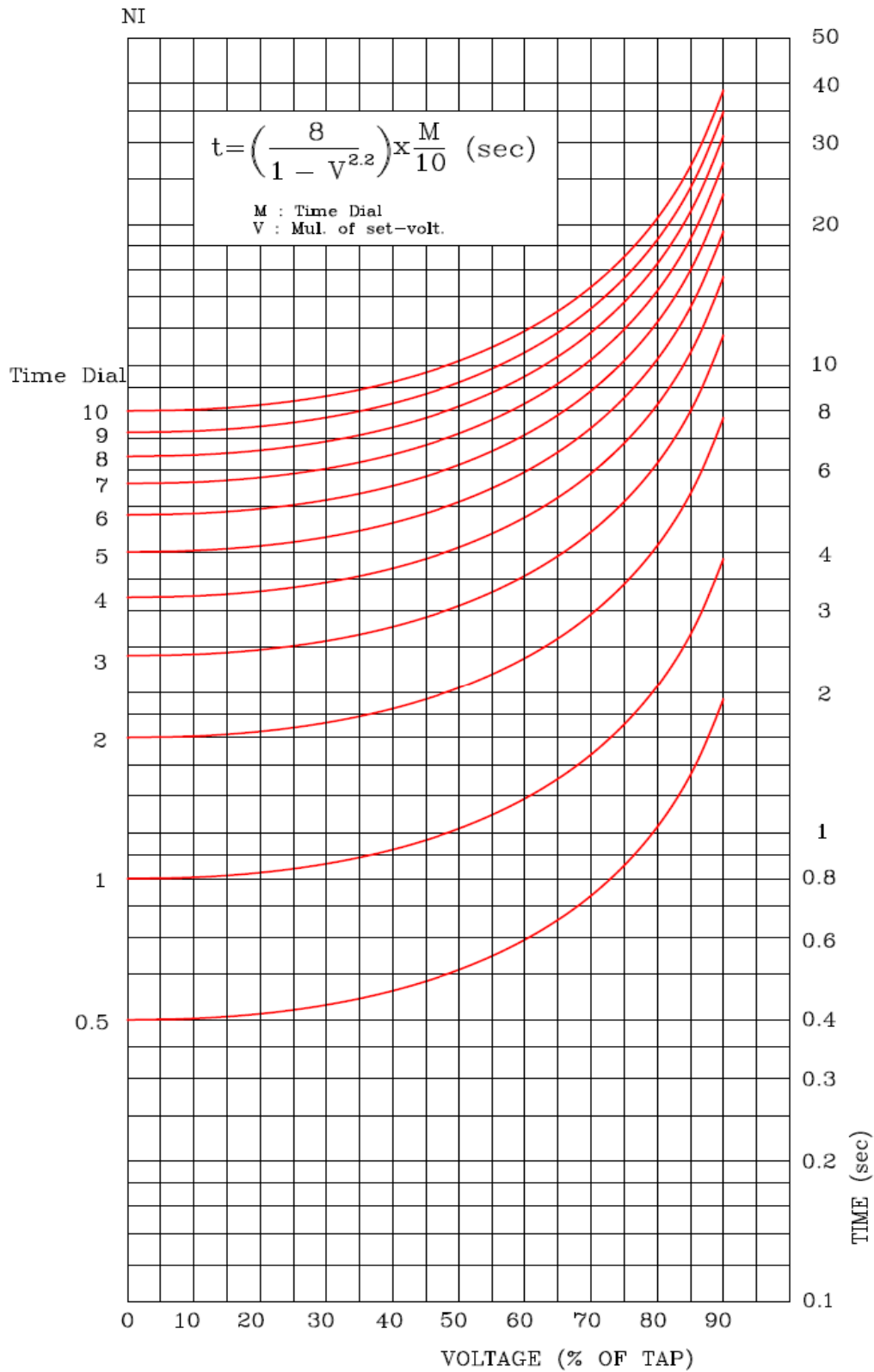
<부도 1.11 저전압 역반한시 특성 곡선>
