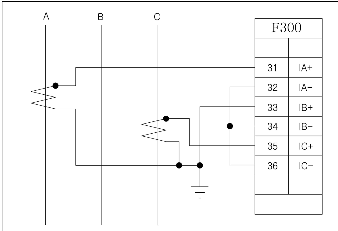
<그림 38. 3상 3선식 2CT결선 - ABC Rotation>
