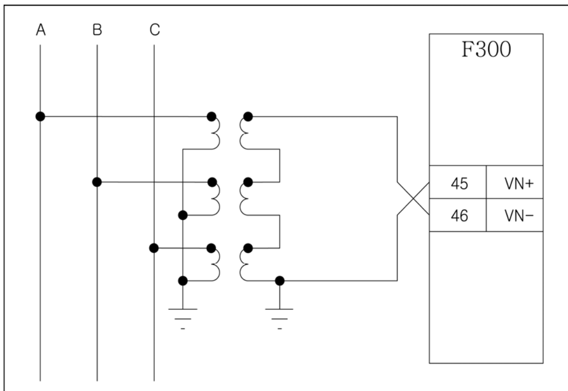
<그림 37. GPT결선>
