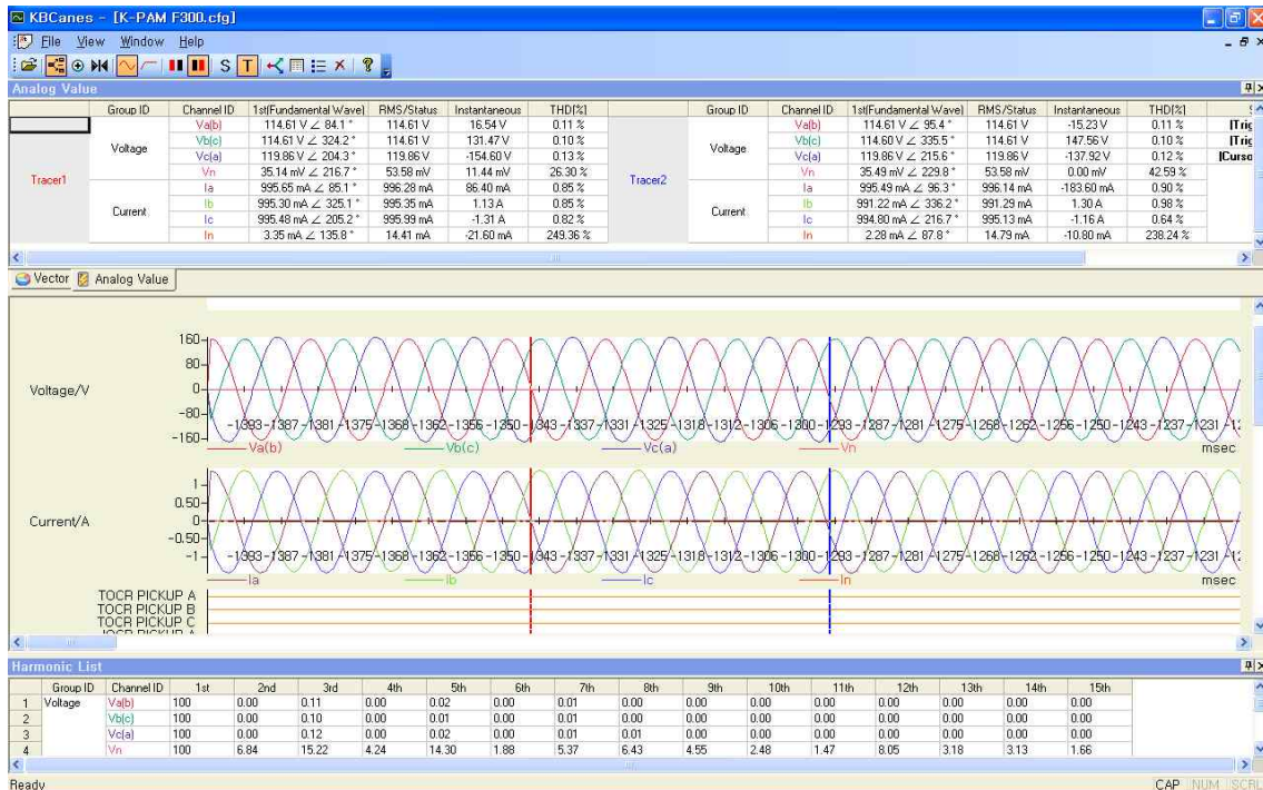
<그림 28. KbCanes>
