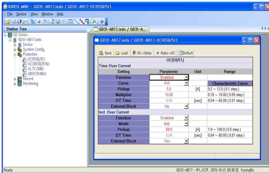
<그림 25. 설정 창 메뉴 화면>
