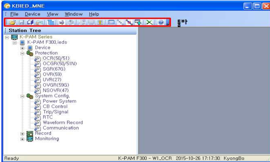
<그림 18. KBIED_MNE 초기 화면>
