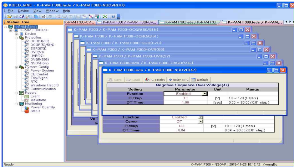
<그림 22. Project Tree 화면>
