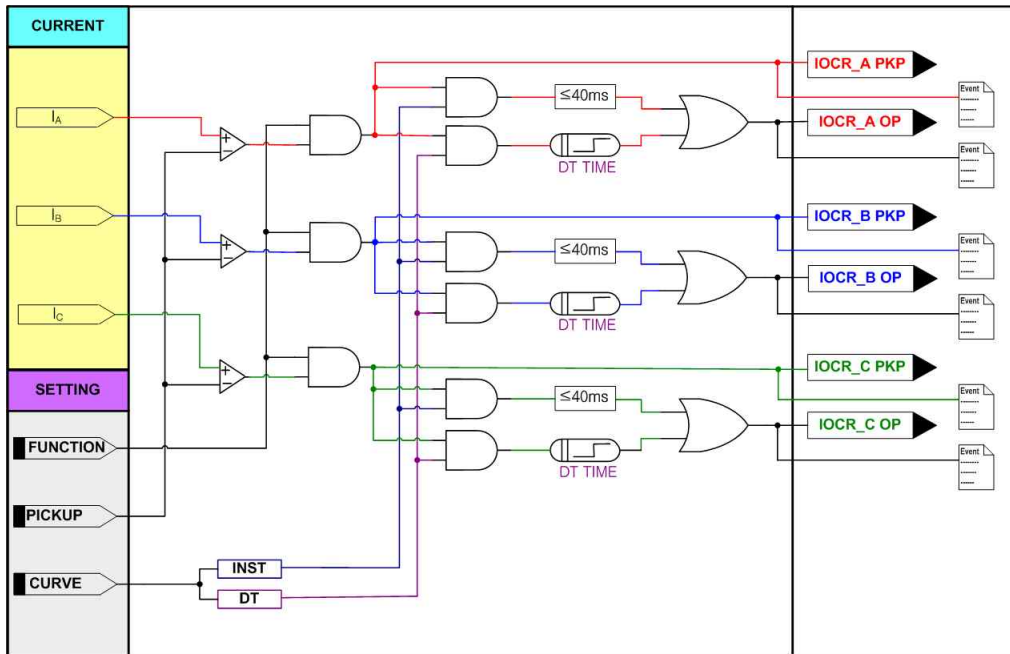
< 그림 6. 순시/제한시 과전류보호 동작특성 >
