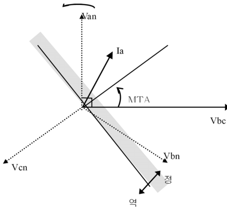
<그림 38. A상 고장 시 방향 특성>
