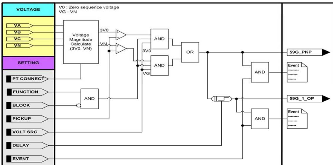
<그림 30. 순시/정한시 지락 과전압보호 동작특성>
