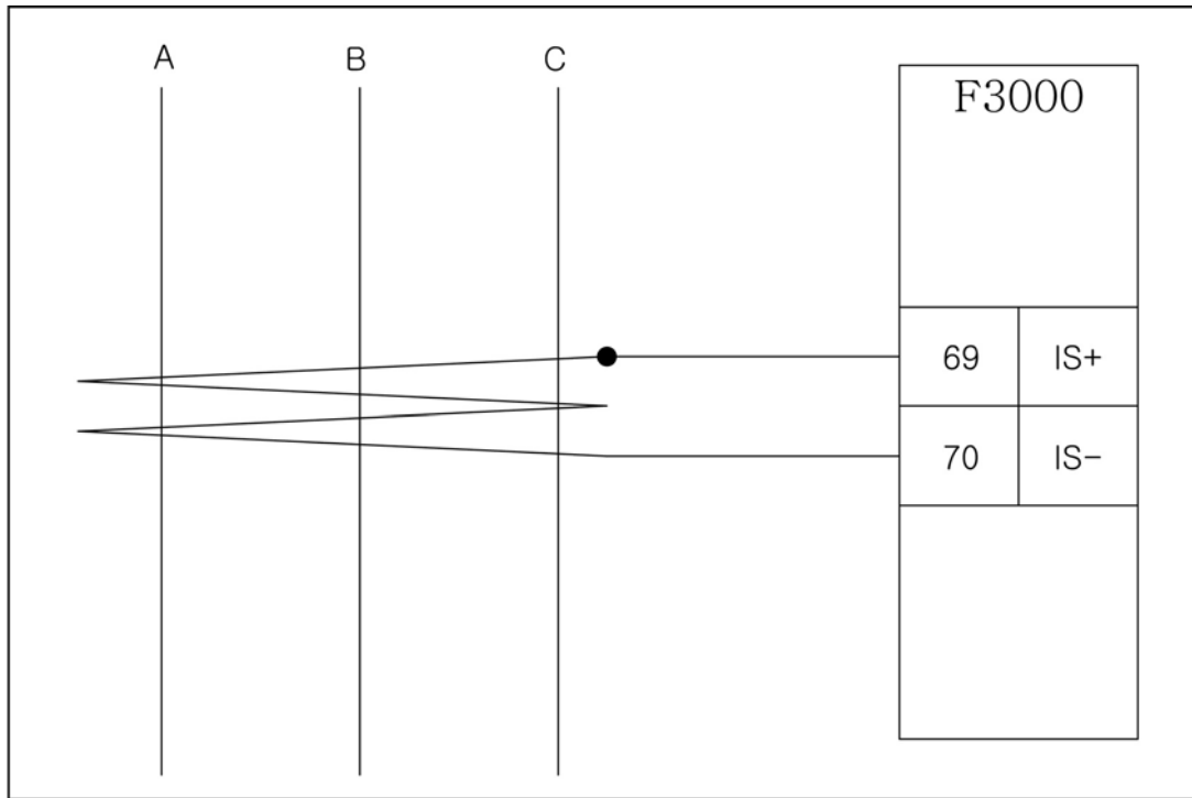
<그림 83. ZCT 결선>
