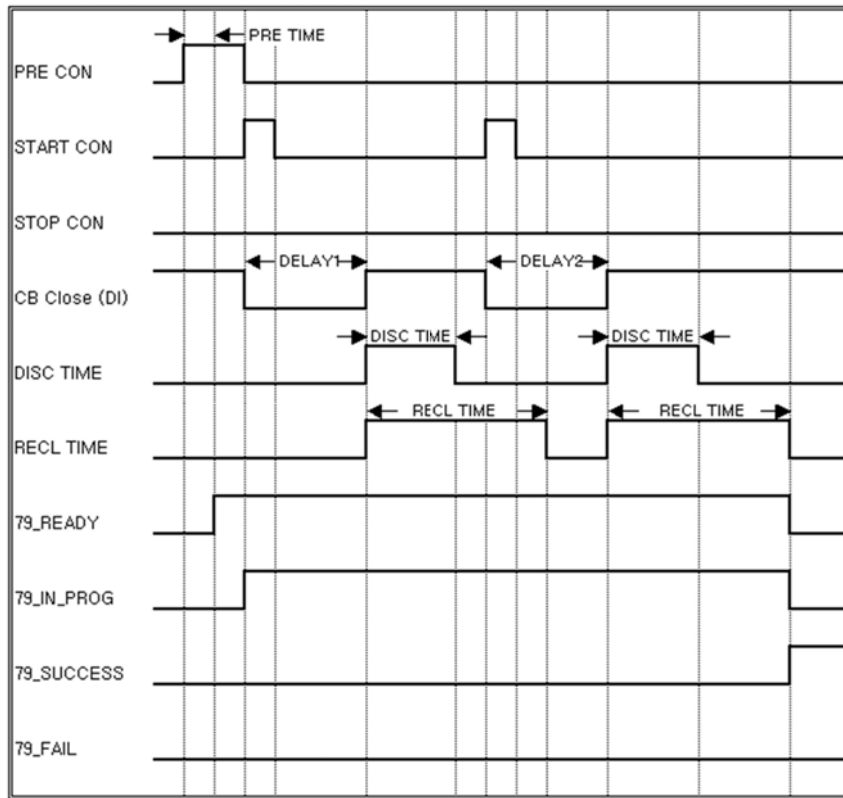
<그림 34. 자동재폐로 2회 재폐로 성공>
