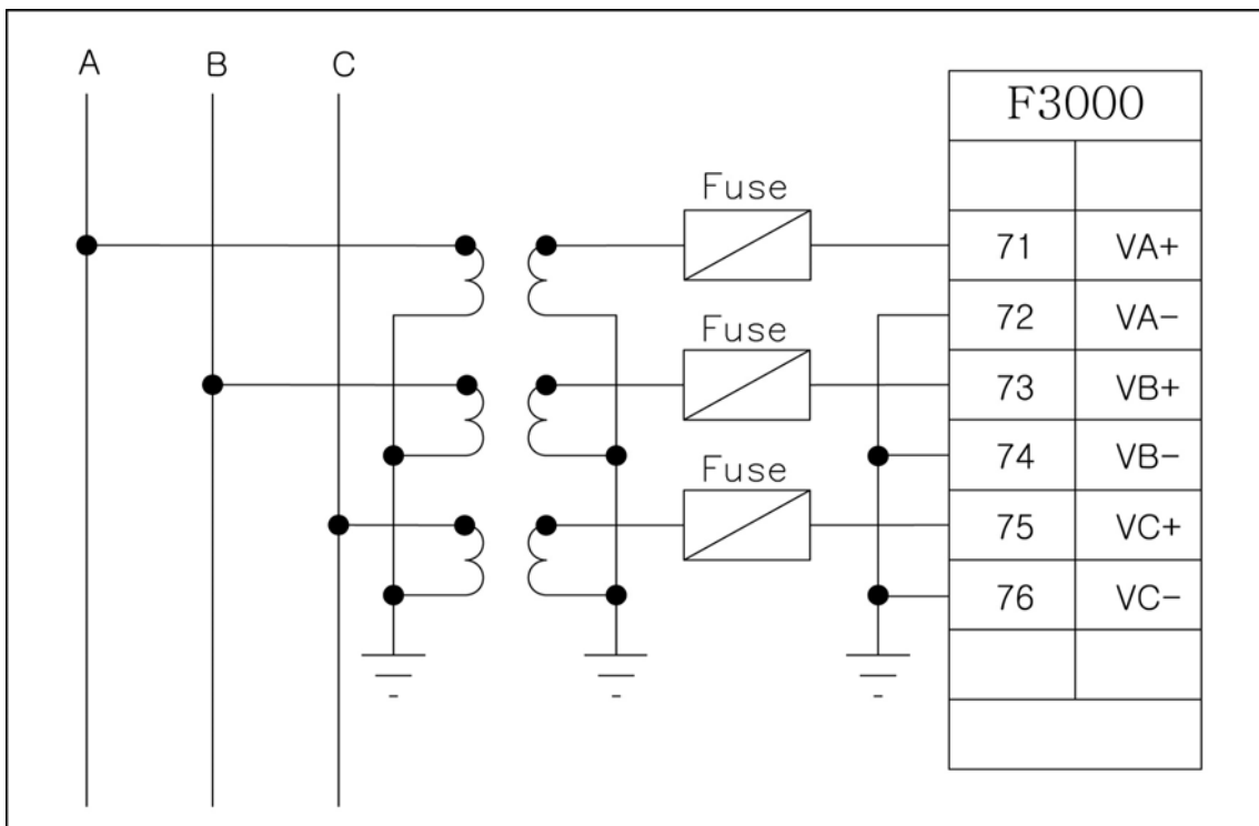
<그림 76. 3상 3선식 3PT 결선 - ABC Rotation>
