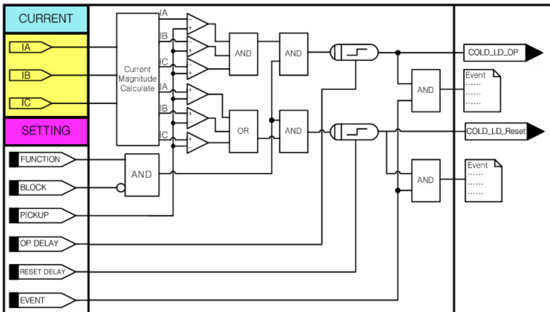
<그림 43. Cold Load Pickup 동작특성>
