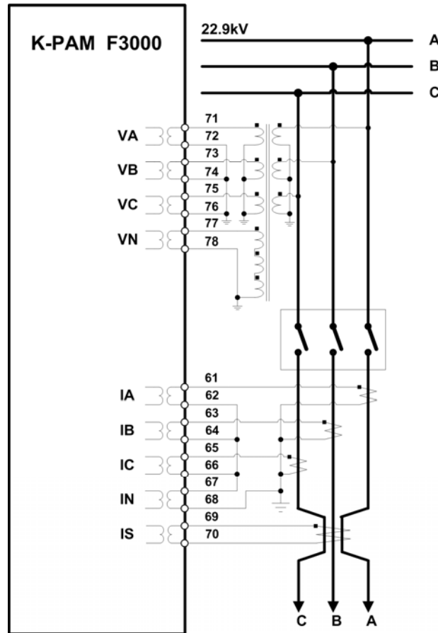
<그림 70. 적용 예시 결선도>
