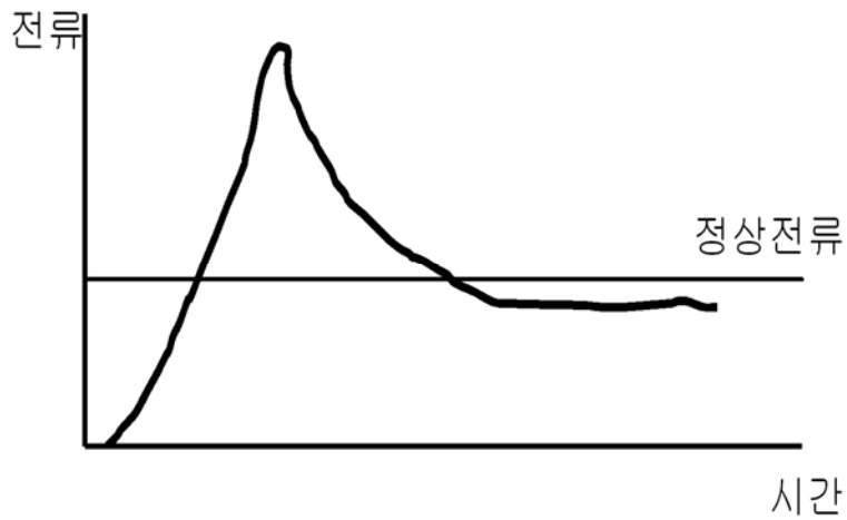
<그림 42. Cold Load Pickup 전류 형태>
