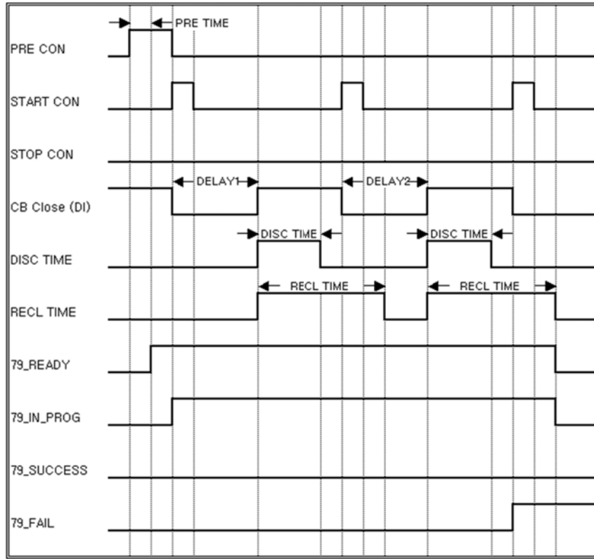
<그림 36. 자동재폐로 2회 재폐로 실패>
