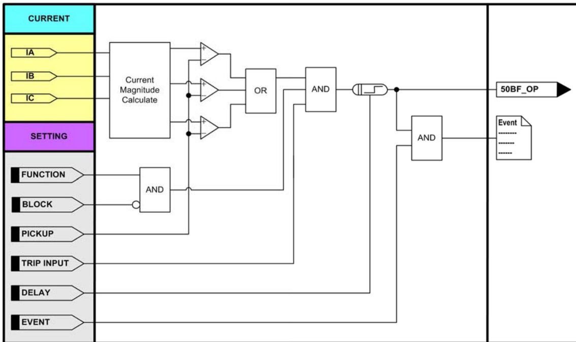
<그림 37. 차단실패 보호 동작특성>
