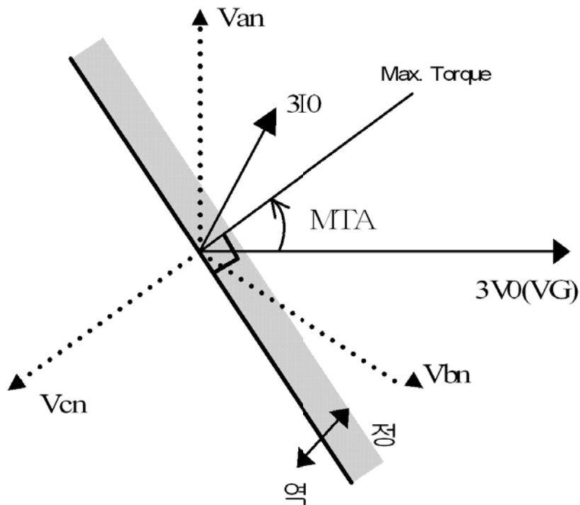
<그림 40. 지락방향 검출 방향 특성>
