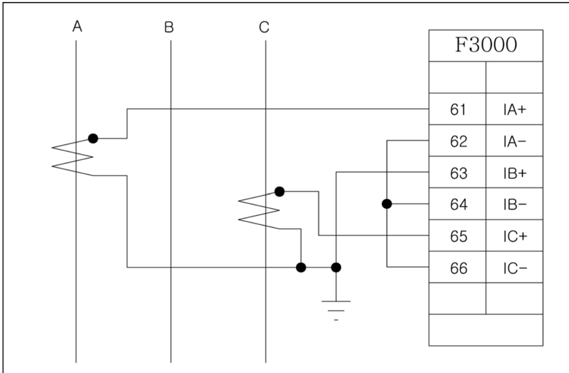
<그림 79. 3상 3선식 2CT 결선 - ABC Rotation>
