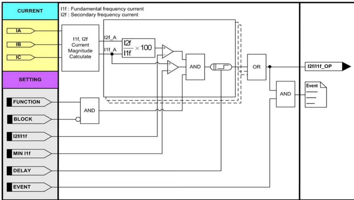
<그림 44. 돌입전류 검출(INRUSH) 동작특성>
