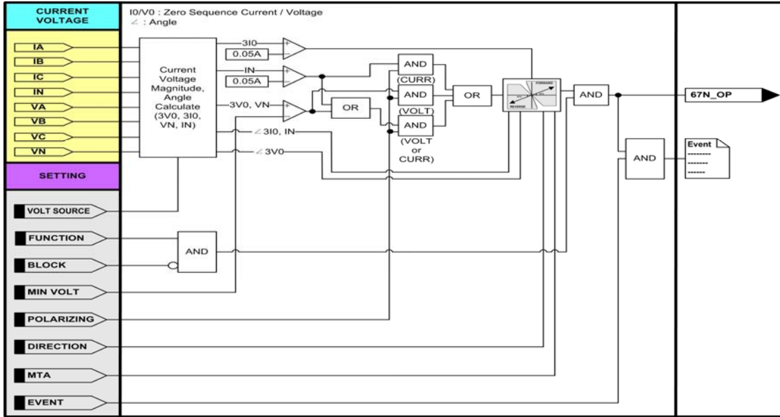
<그림 41. 지락방향 검출 동작특성>
