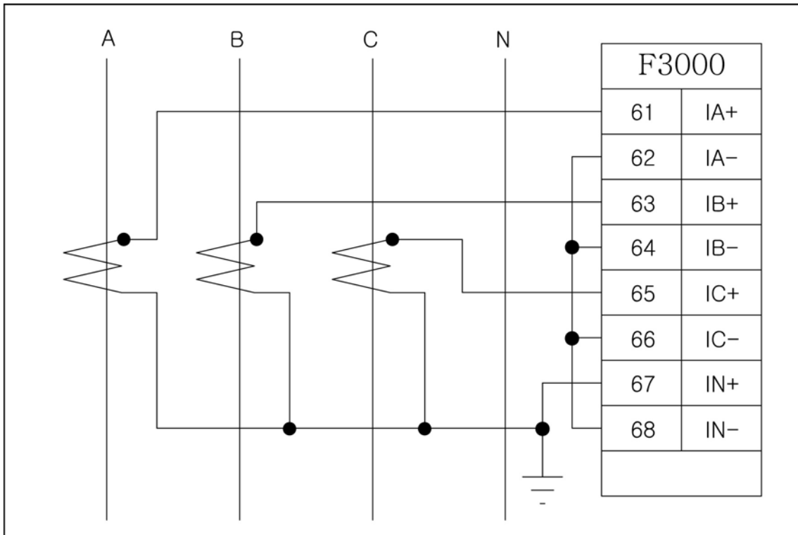
<그림 81. 3상 4선식 3CT 잔류회로 결선 - ABC Rotation>
