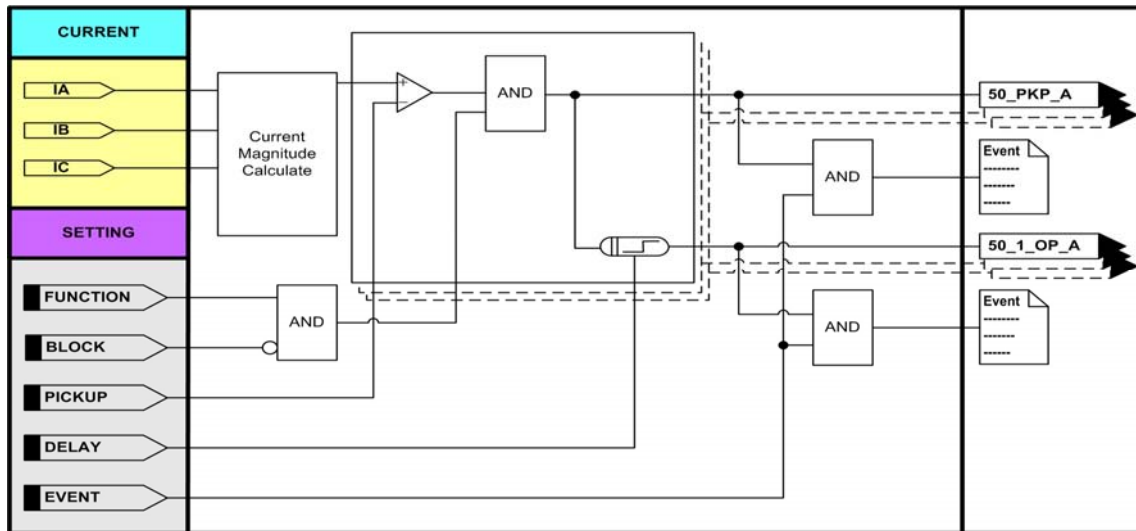
<그림 16. 순시/정한시 단락과전류보호 동작특성>
