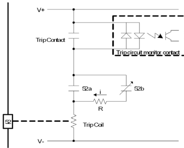
<그림 13. TCS 회로 구성>
