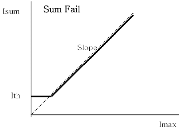
<그림 7. 전류입력회로 감시 특성 Curve>
