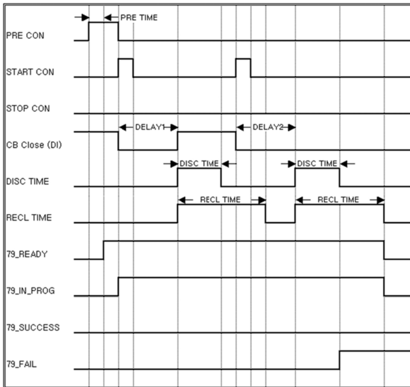
<그림 35. 자동재폐로 2회 재폐로 차단기 투입 실패>
