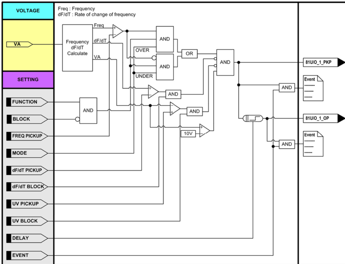
<그림 33. 저/과주파수보호 동작특성>
