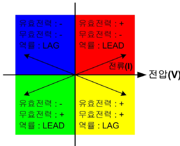
<그림 5. F3000 유효/무효전력의 부호 및 역률 표시>
