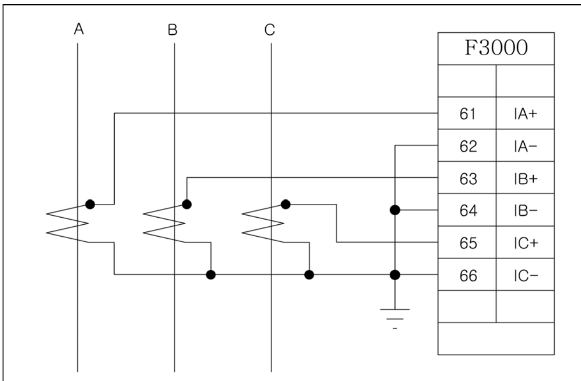
<그림 80. 3상 3선식 3CT 결선 - ABC Rotation>
