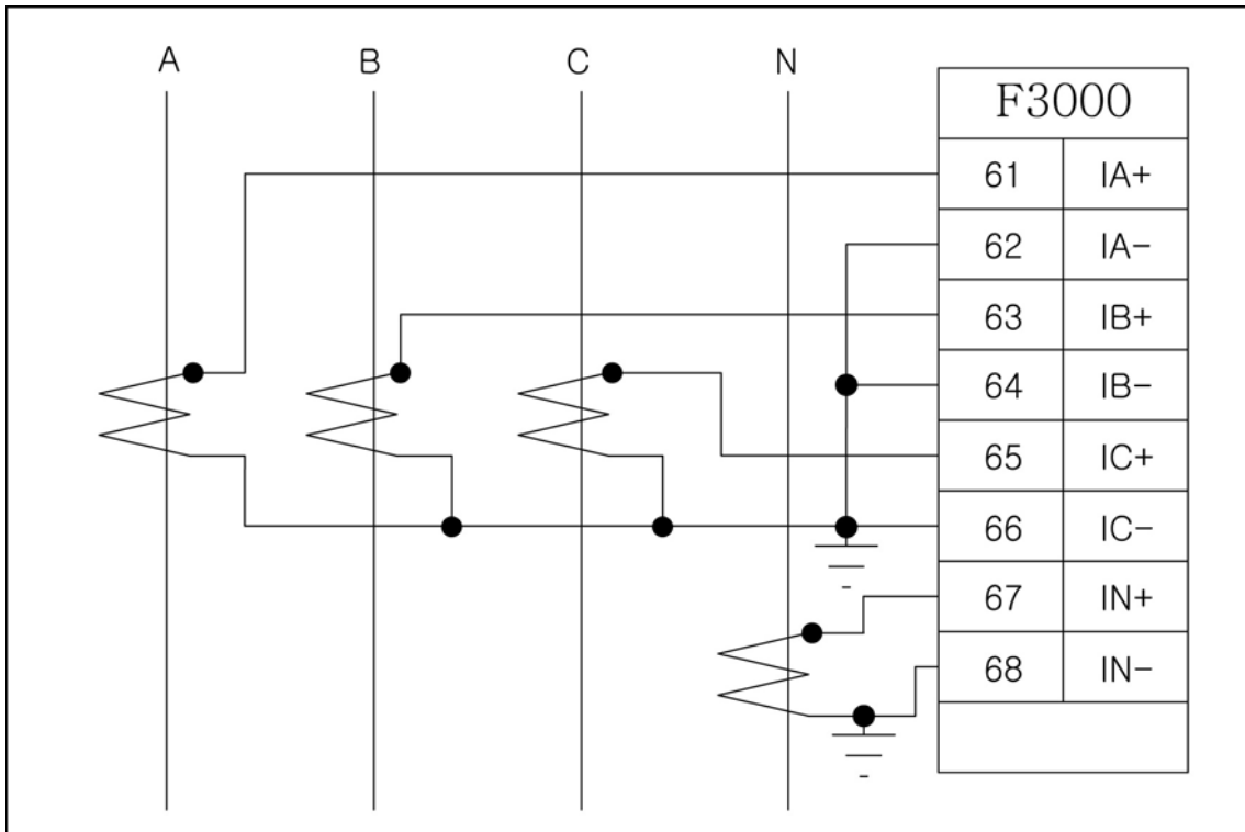
<그림 82. 3상 4선식 4CT 결선 - ABC Rotation>
