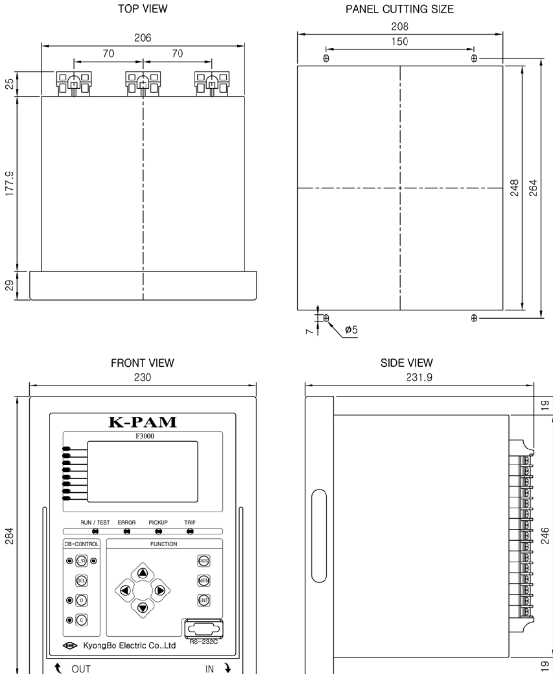
<그림 73. K-PAM F3000 치수도>
