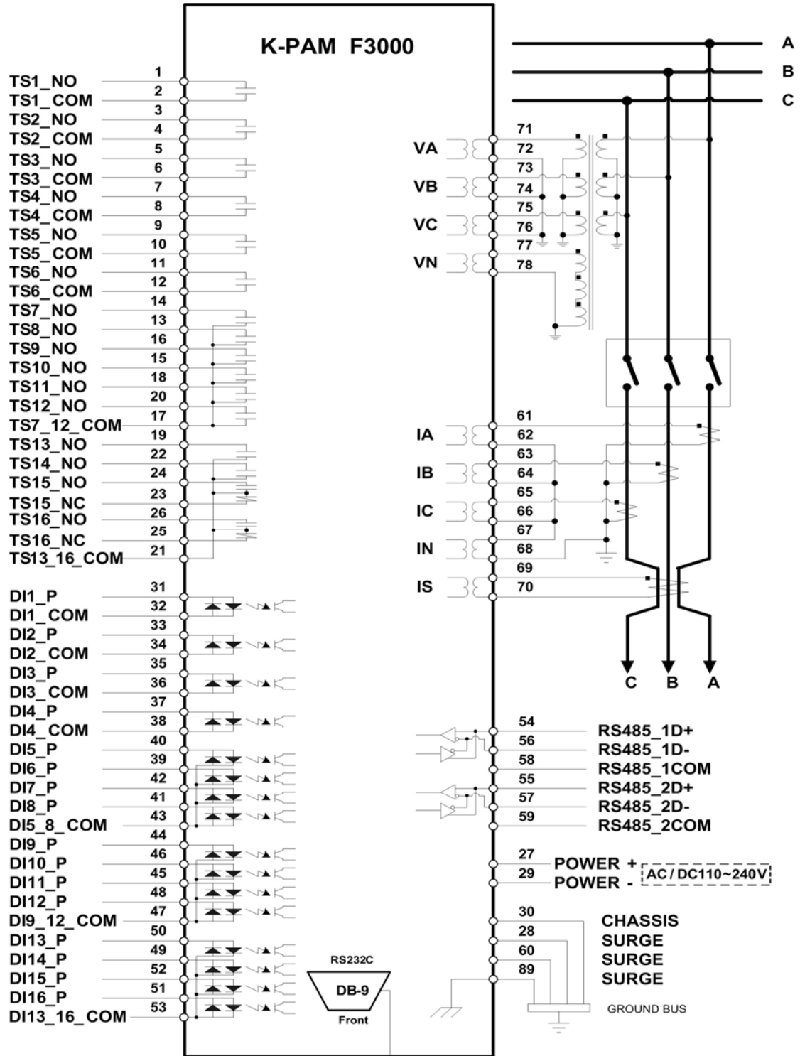
<그림 74. K-PAM F3000 외부 결선도>
