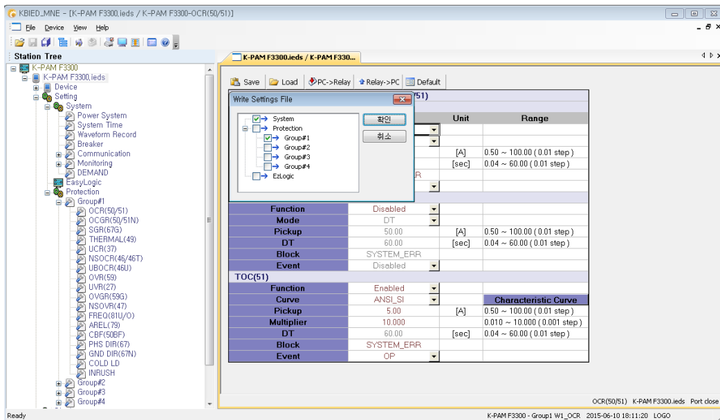
<Figure 56. 저장된 파일 Device로 Write하기>
