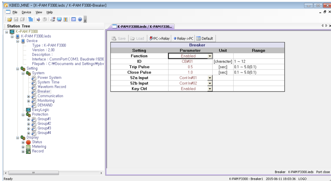
<Figure 64. Breaker 화면>
