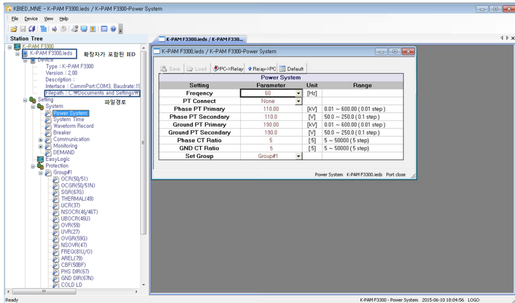
<Figure 52. Project 저장 화면>
