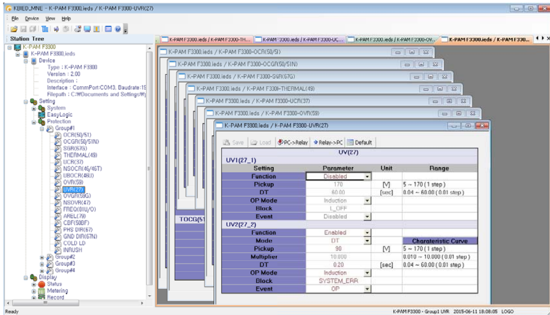
<Figure 68. Protection 화면>
