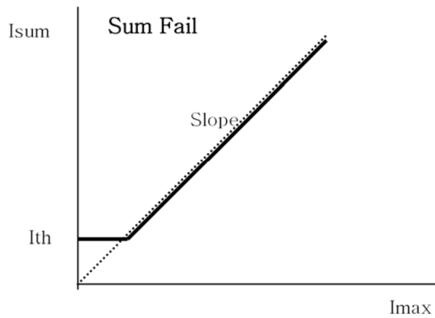
<Figure 7. 전류입력회로 감시 특성 Curve>
