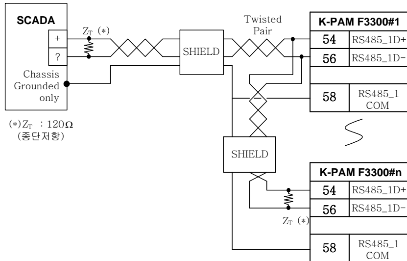
<Figure 104. RS-485 통신포트 결선도>
