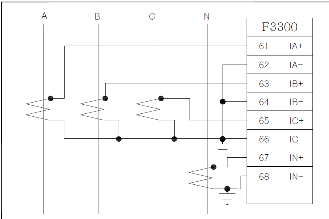
<Figure 100. 3상 4선식 4CT 결선 - ABC Rotation>
