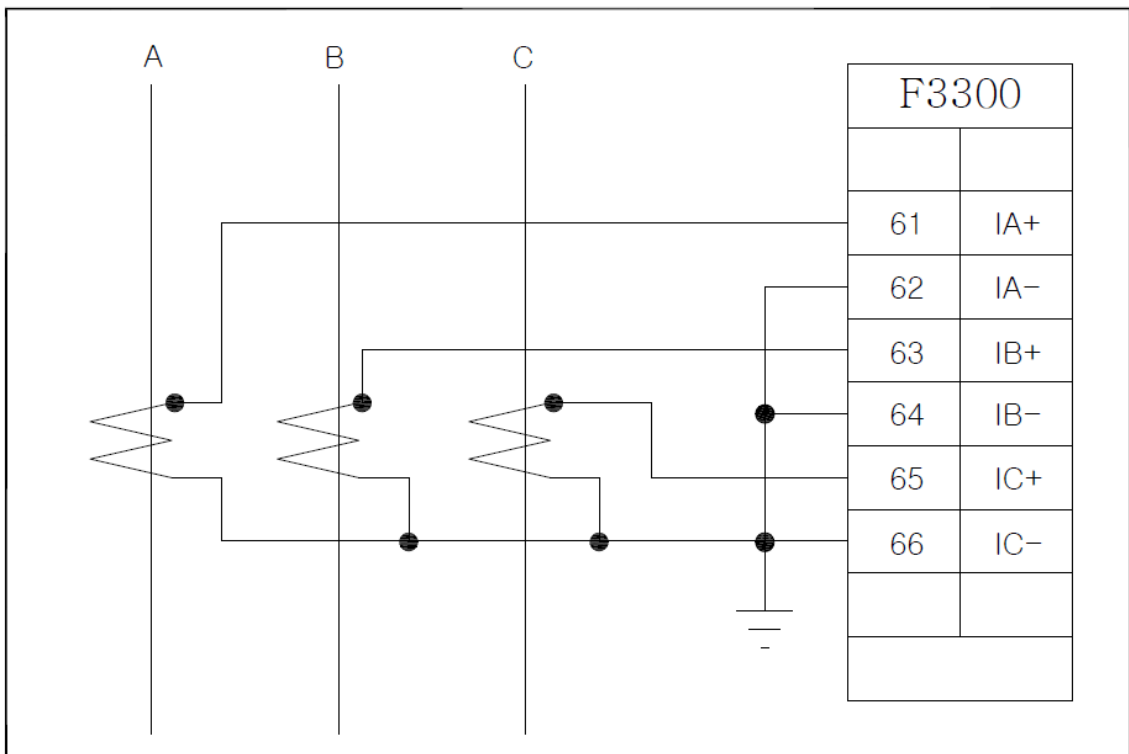
<Figure 98. 3상 3선식 3CT 결선 - ABC Rotation>
