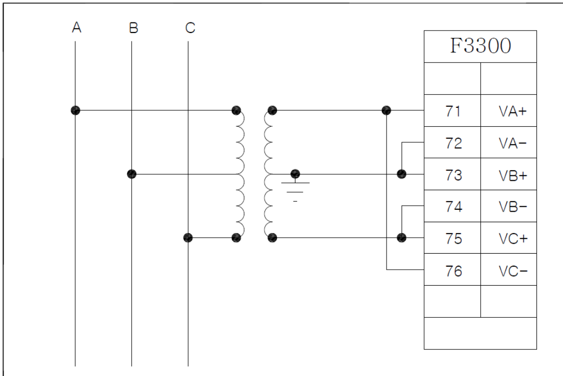
<Figure 93. 3상 3선식 V 결선 - ABC Rotation>
