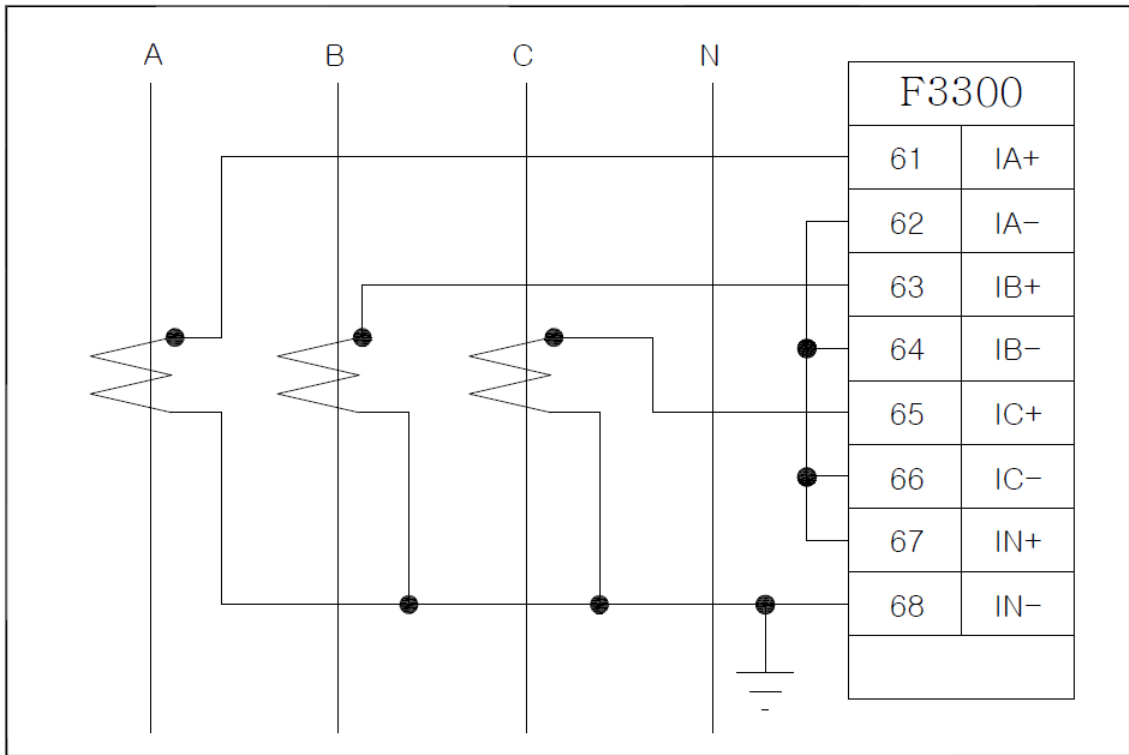
<Figure 99. 3상 4선식 3CT 잔류회로 결선 - ABC Rotation>
