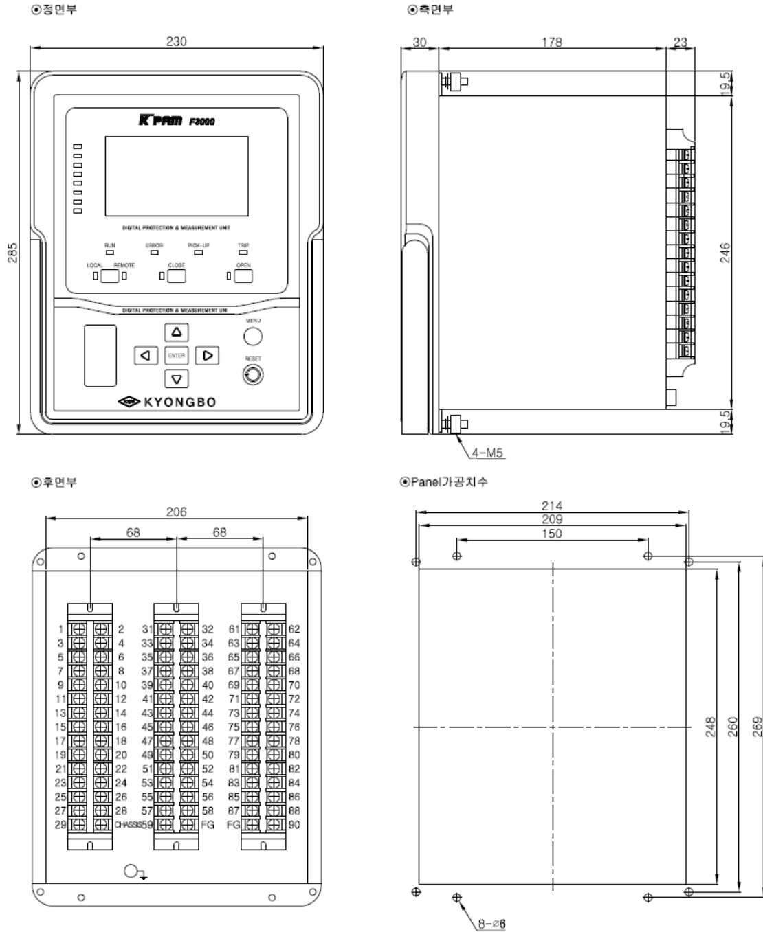
<Figure 91. K-PAM F3300 치수도>
