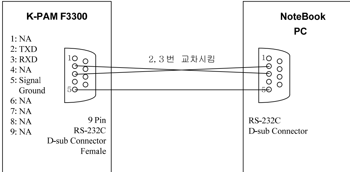
<Figure 103. RS-232C 통신포트 결선도>
