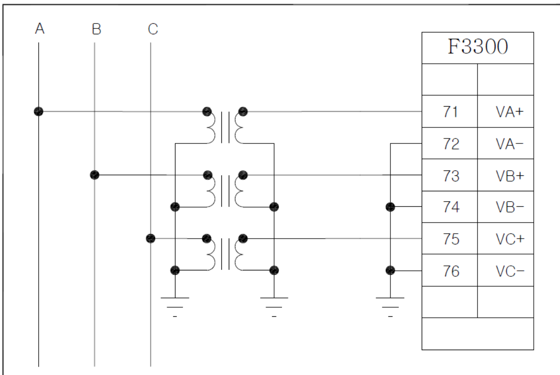
<Figure 94. 3상 3선식 3PT 결선 - ABC Rotation>
