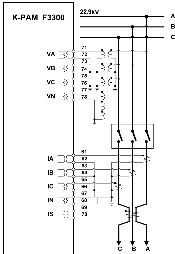
<Figure 88. 적용 예시 결선도>
