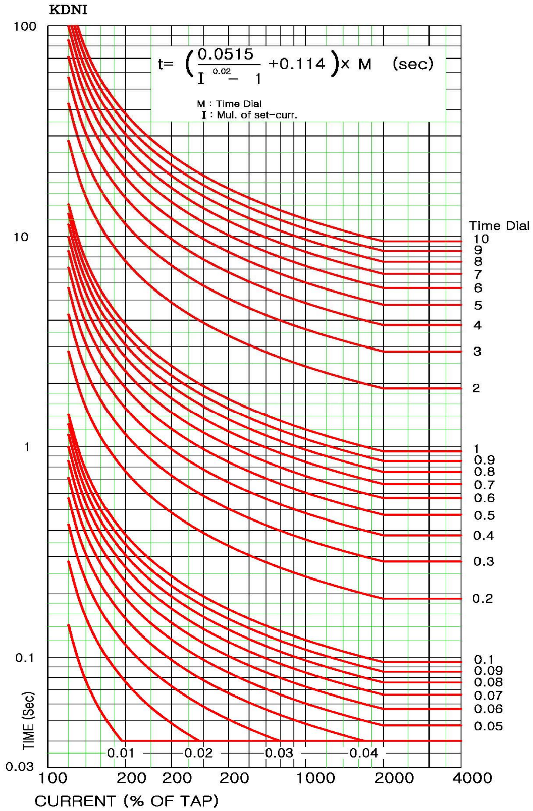
<부도 1.14 과전류/지락과전류/역상과전류 KEPCO_DNI 특성 곡선>
