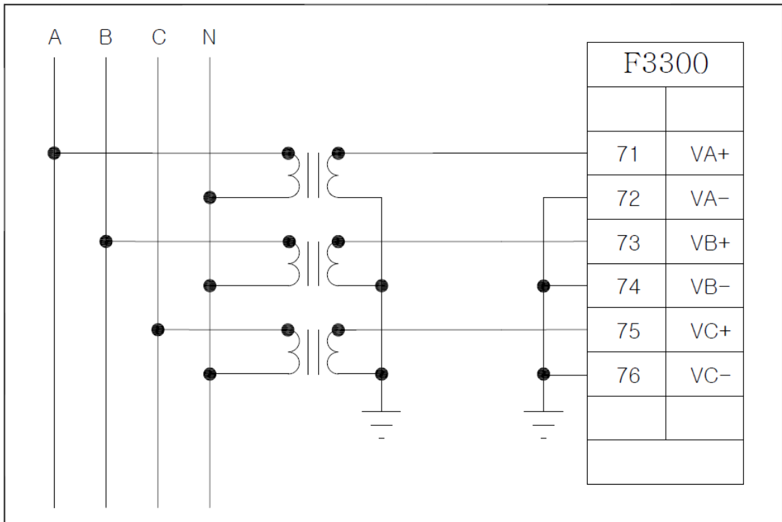
<Figure 95. 3상 4선식 3PT 결선 - ABC Rotation>
