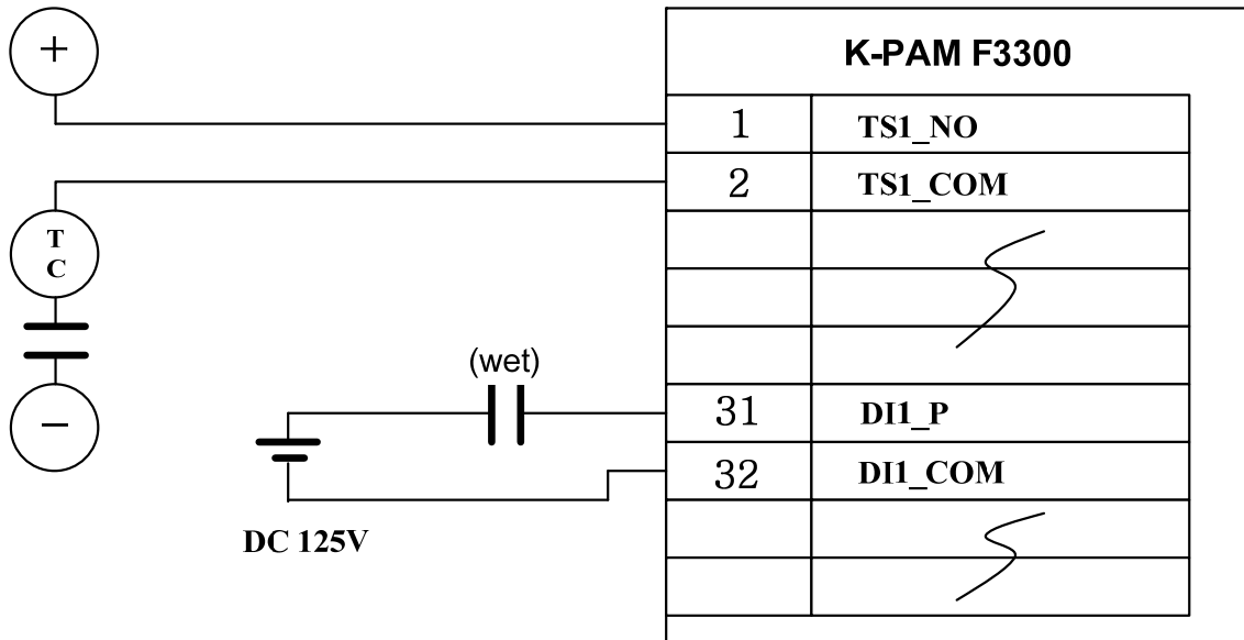
<Figure 102. 입력/출력접점 결선도>
