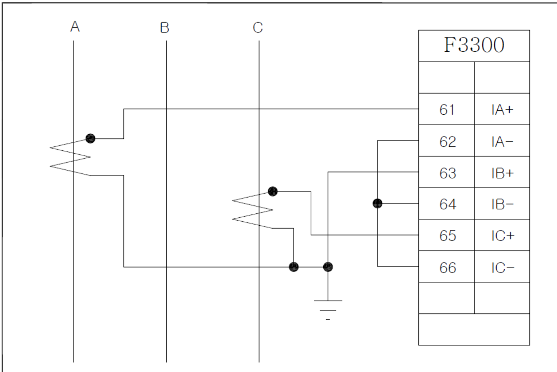
<Figure 97. 3상 3선식 2CT 결선 - ABC Rotation>
