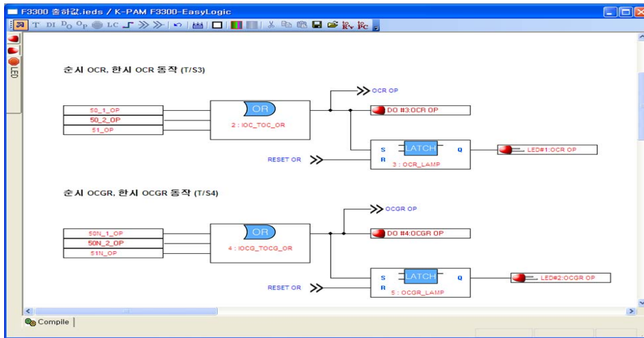
<Figure 69. EasyLogic 구성 예>
