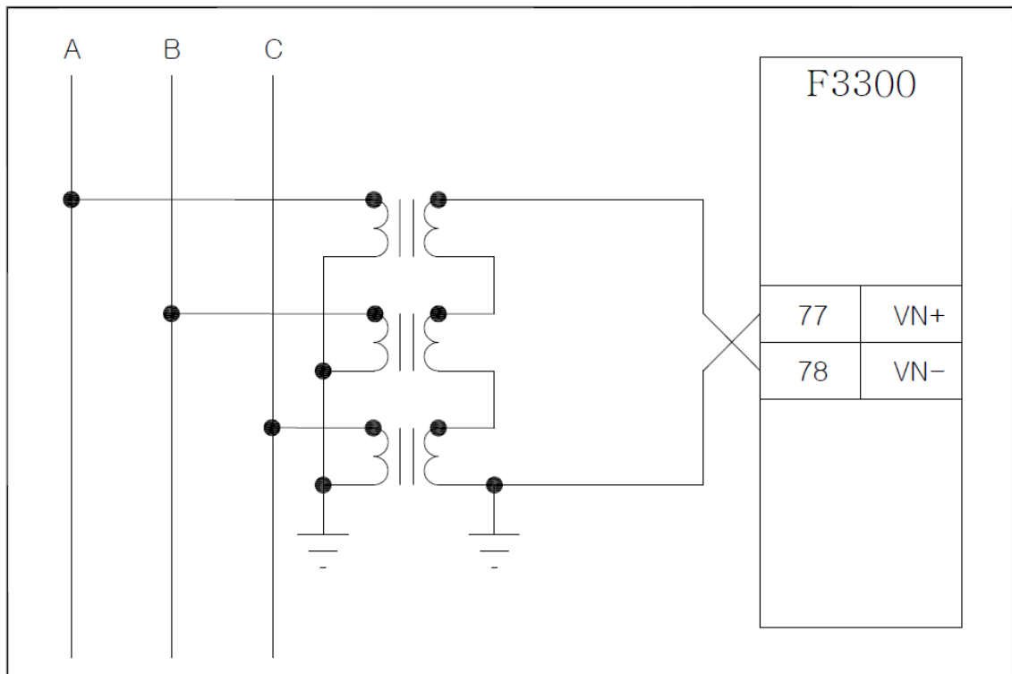
<Figure 96. GPT 결선 >
