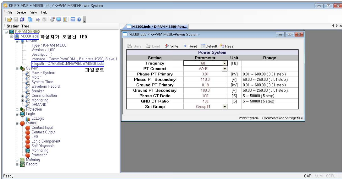
<Figure 51. Project 저장 화면>
