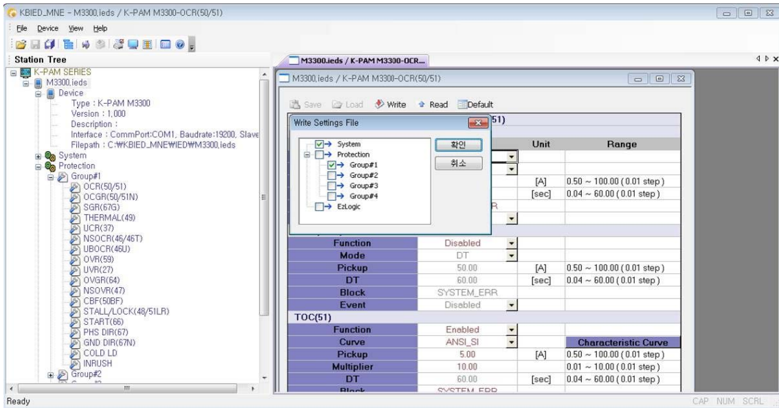
<Figure 55. 저장된 파일 Device로 Write하기>
