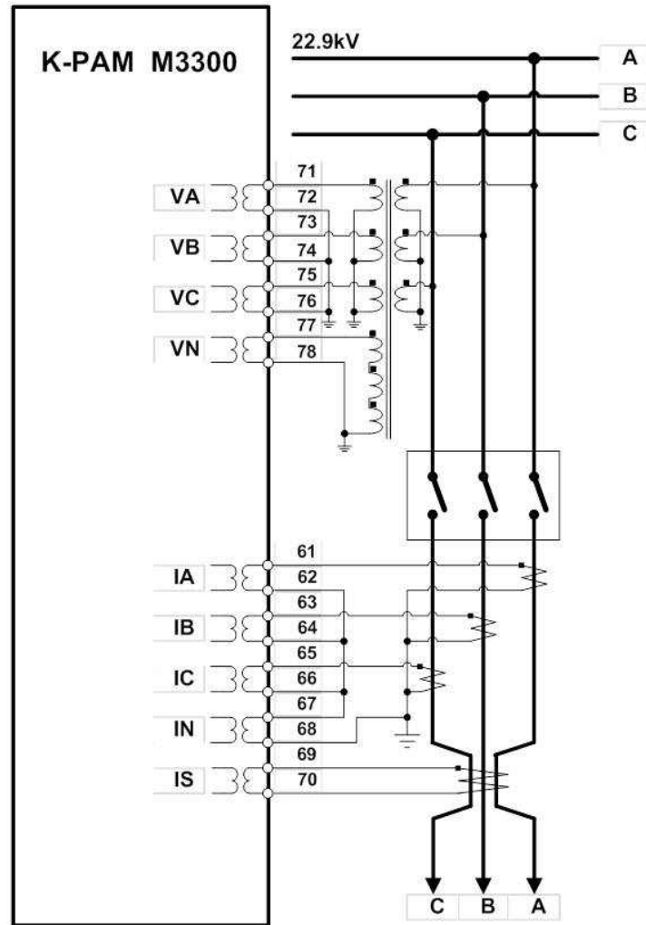
<Figure 91. 적용 예시 결선도>
