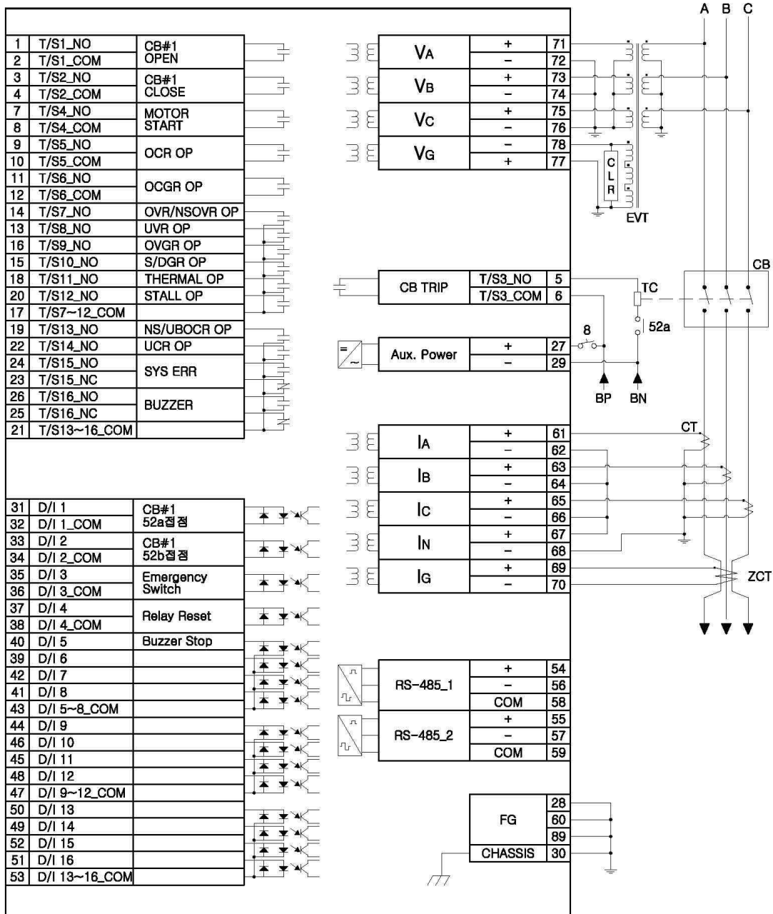
<Figure 95. K-PAM M3300 외부 결선도>
