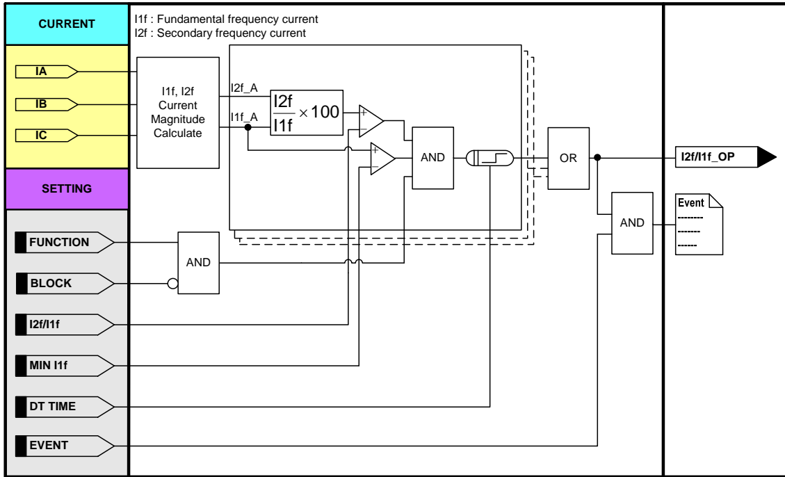
<Figure 27. 돌입전류 검출(INRUSH) 동작특성>
