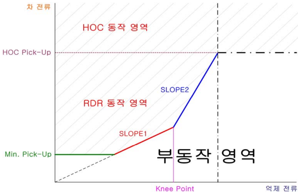
<Figure 7. 전류 단순/비율 차동 보호 동작 영역>
