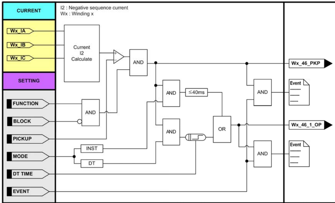
<Figure 15. 순시/제한시 역상 과전류보호 동작특성>
