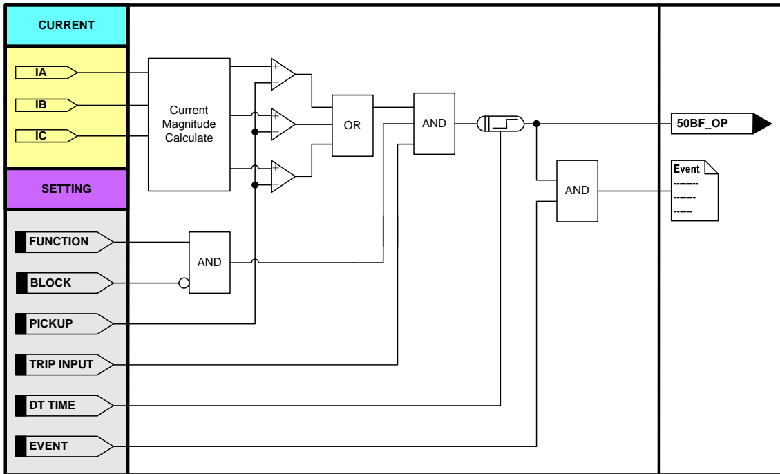
<Figure 24. 차단실패 보호 동작특성>
