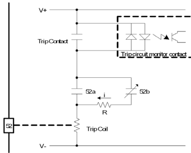
<Figure 5. TCS 회로 구성>
