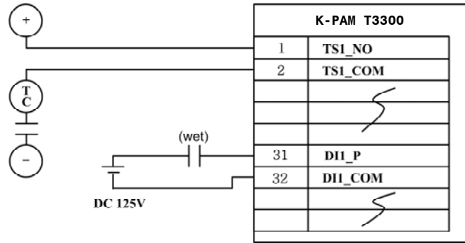
<Figure 74. 입력/출력접점 결선도>
