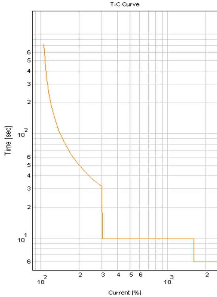
<Figure. 단락/지락 과전류보호 동작특성>
