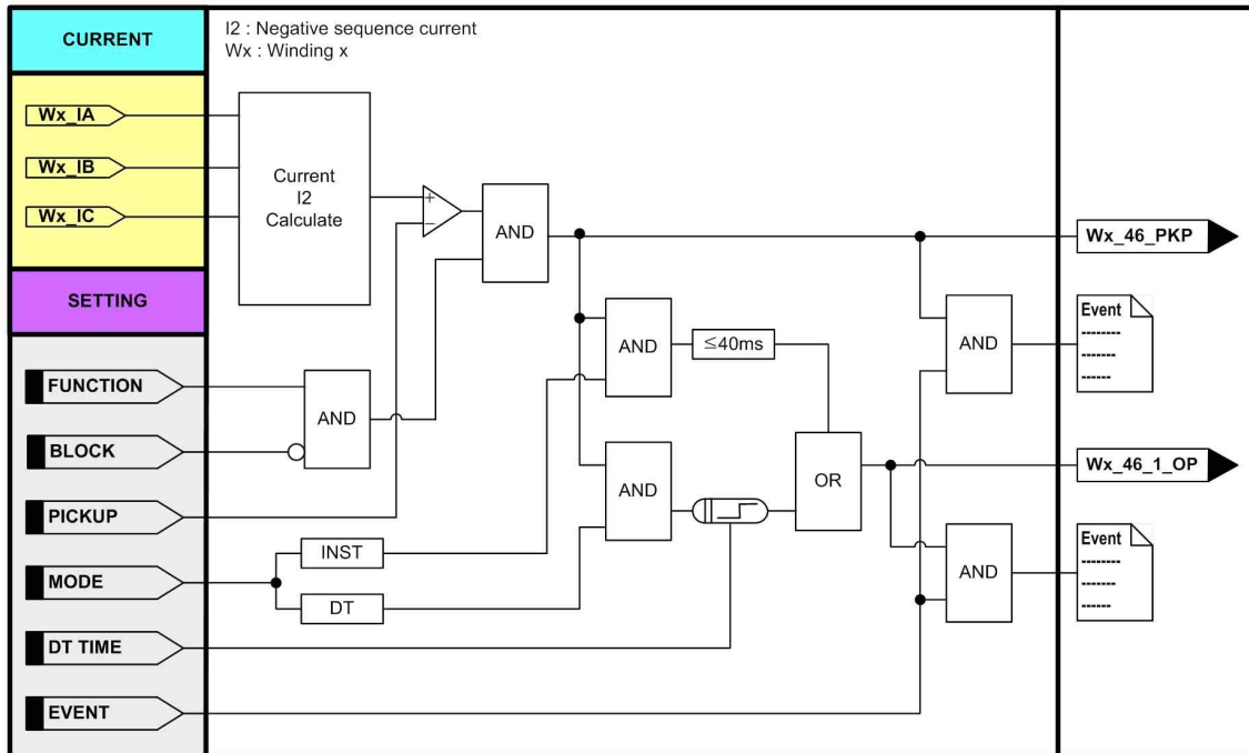
<Figure. 순시/정한시 역상 과전류보호 동작특성>
