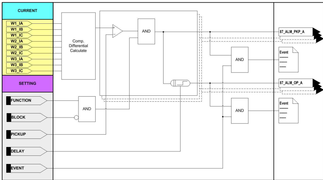
<Figure. 차전류 경보 동작 특성>
