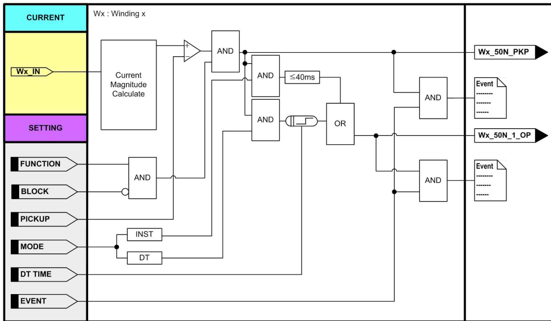
<Figure. 순시/정한시 지락과전류보호 동작특성>
