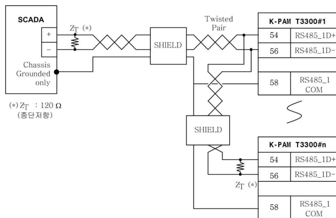
<Figure. RS-485 통신포트 결선도>
