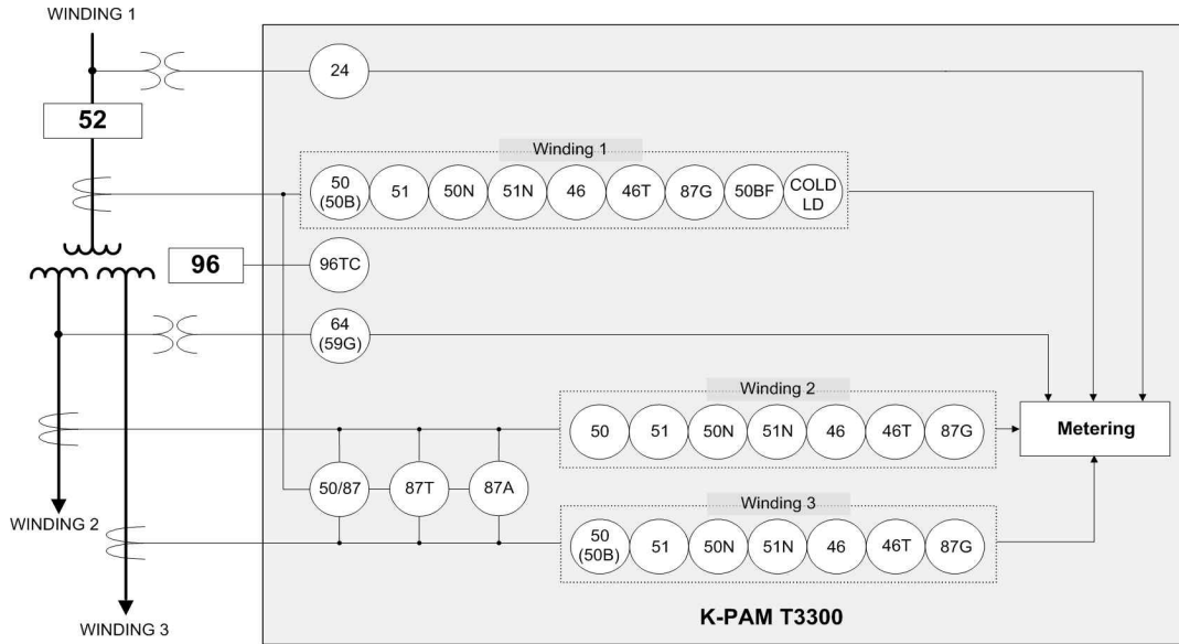
<Figure. 기능 단선도>
