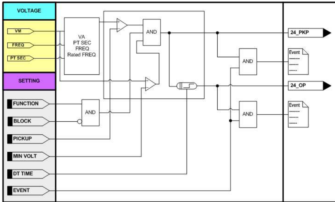
<Figure. 과여자 보호 동작특성>
