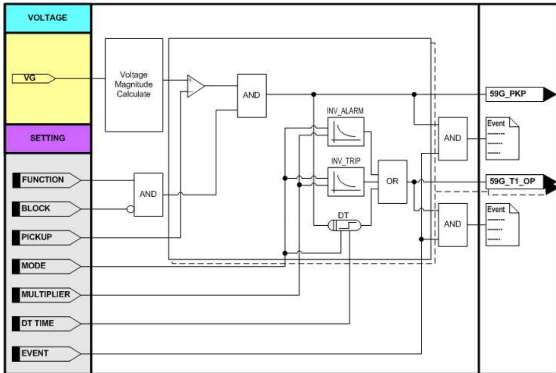
<Figure. 한시 지락 과전압보호 동작특성>
