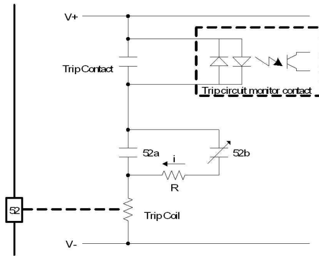
<Figure. TCS 회로 구성>
