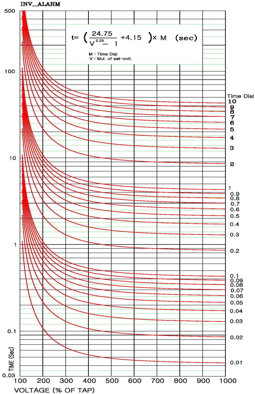
<부도 1.17 지락 과전압 Alarm용 반한시 특성 곡선>
