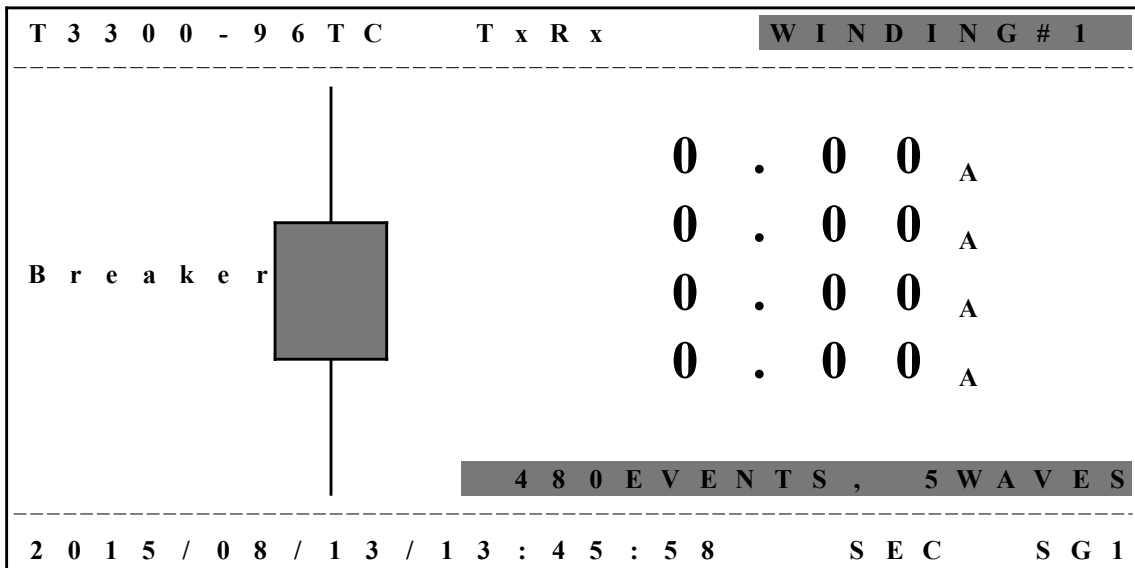
<Figure. 변압기 기계적 보호장치 사용시 전면 표시부>
