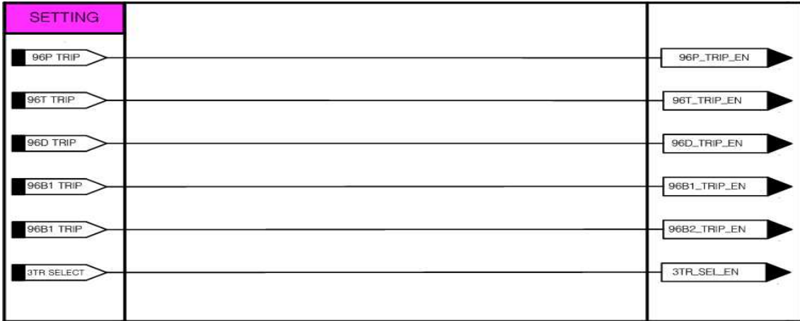
<Figure. 변압기 기계적보호장치 트립제어(96TC) 동작특성>
