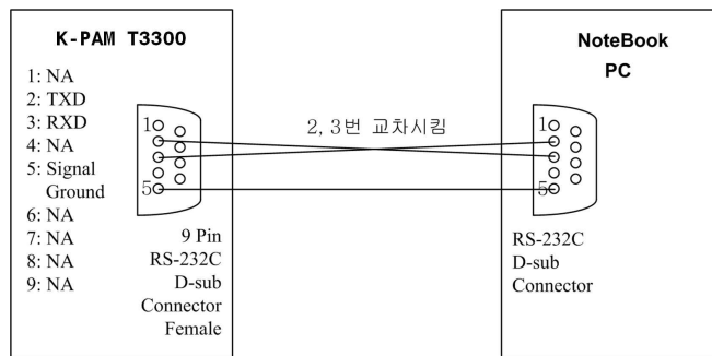
<Figure. RS-232C 통신포트 결선도>
