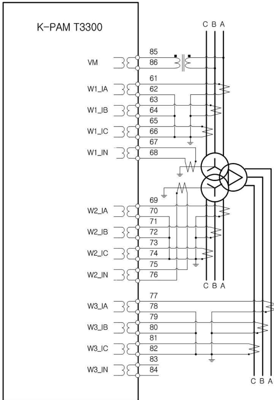
<Figure. K-PAM T3300 3권선 변압기 보호용 외부 결선도>
