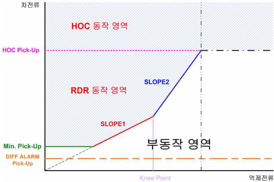
<Figure. 전류 단순차동/비율차동/차전류 경보 동작 영역>
