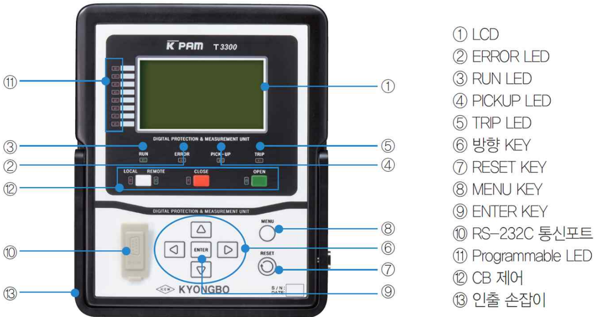
<Figure. 전면 표시부>
