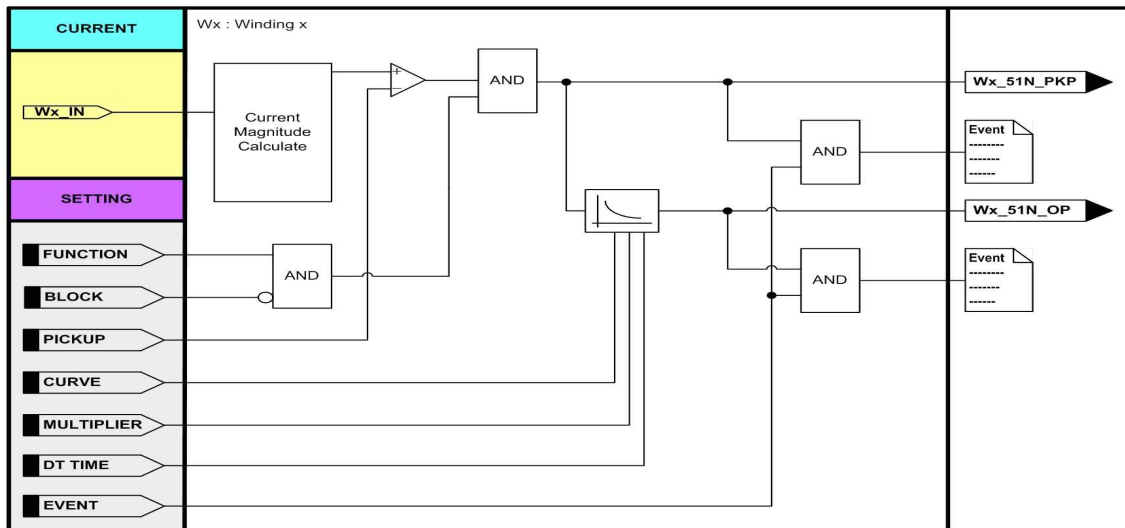
<Figure. 한시 지락과전류보호 동작특성>
