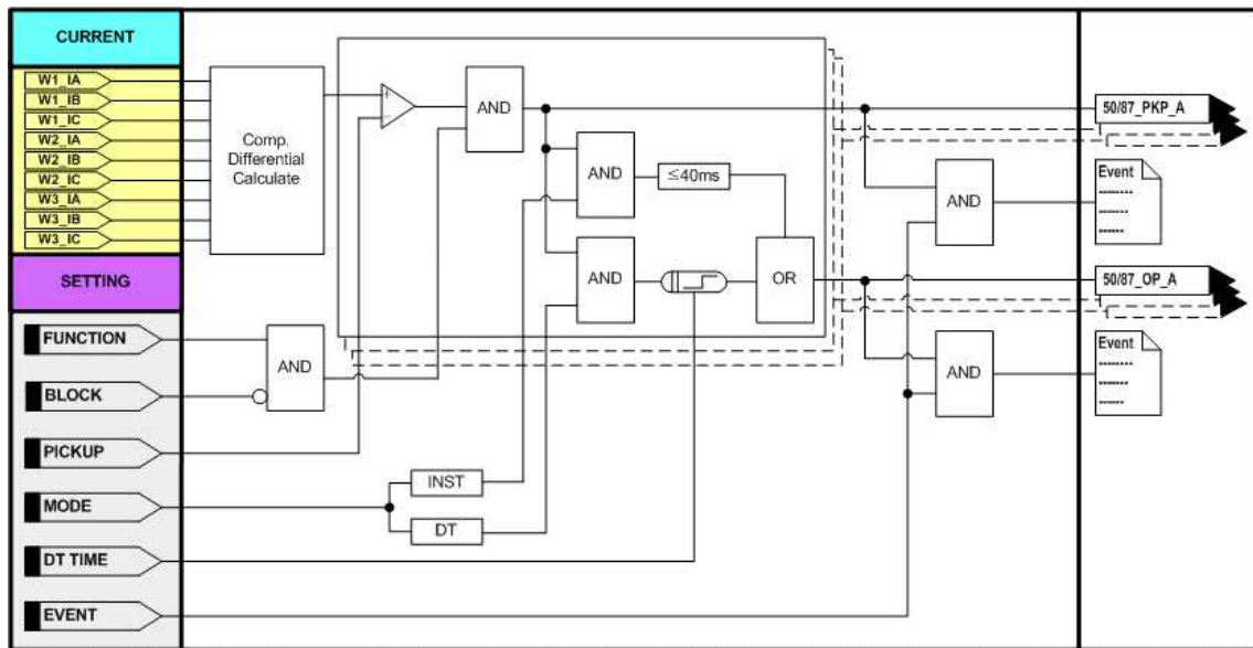
<Figure. 전류 단순 차동 보호 동작 특성>
