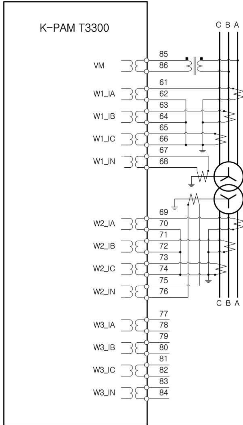
<Figure. K-PAM T3300 2권선 변압기보호용 외부 결선도>
