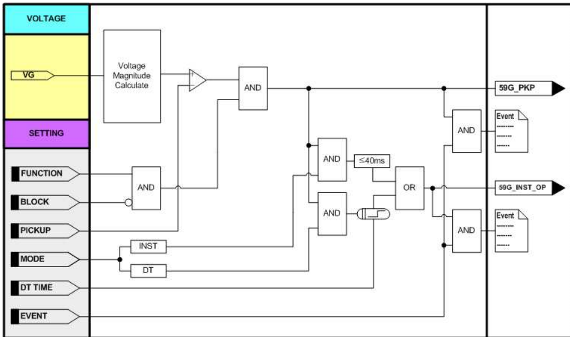
<Figure. 순시/정한시 지락 과전압보호 동작특성>
