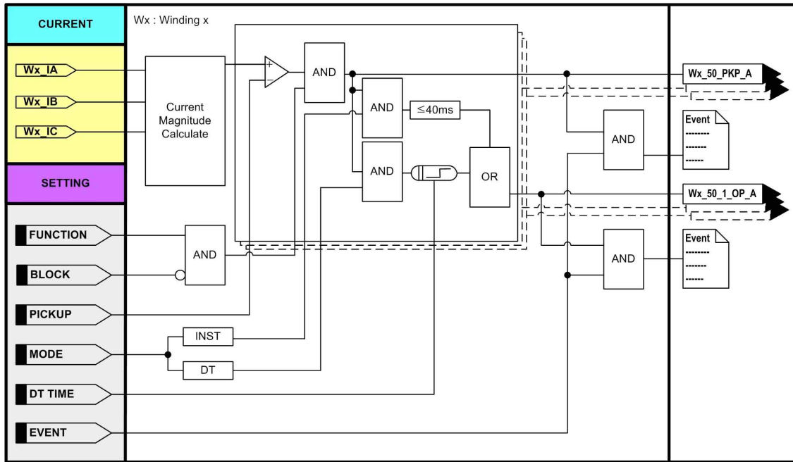
<Figure. 순시/정한시 단락과전류보호 동작특성>
