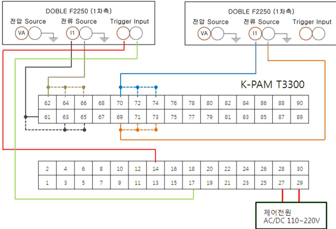
<Figure. 계전기 Test 장비와 K-PAM T3300 결선도>
